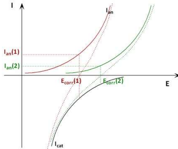
Figure 2-8 : Évolution de E_{corr} (= OCP) en fonction du courant anodique.
