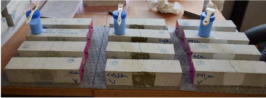
Figure 55 : Photo des échantillons lors de l'application des produits sur des échantillons prismatiques (fissurés)
