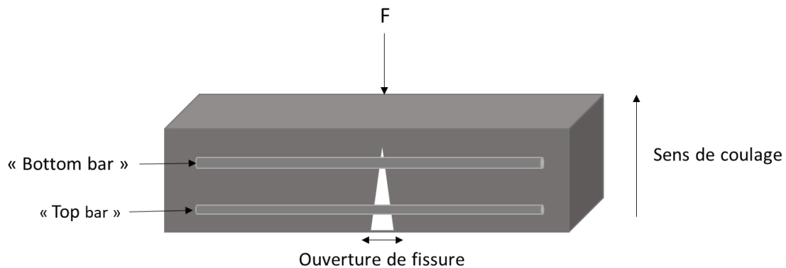
Figure 44 : Schémas de la pré-fissuration d'une poutrelle en flexion 3 points
