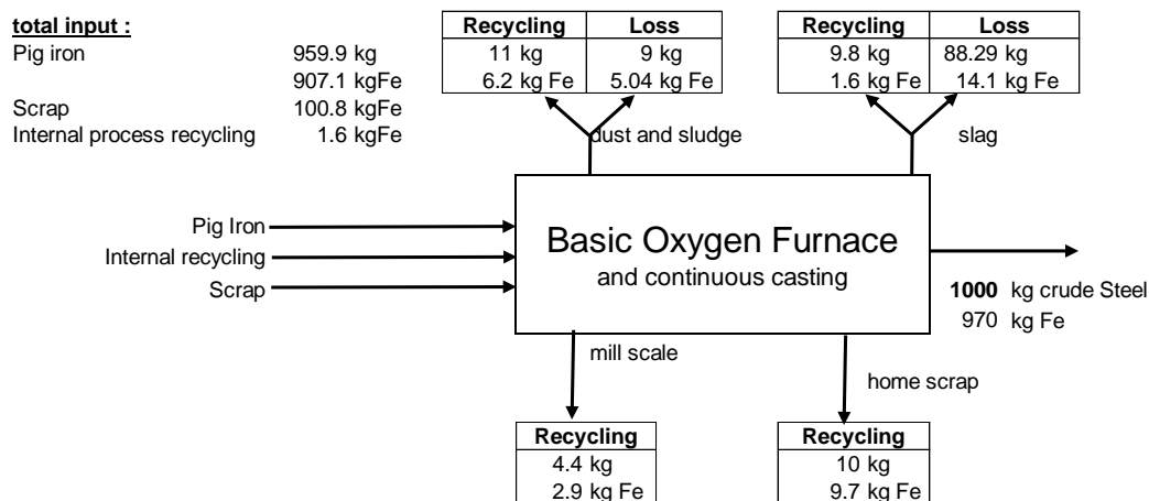
Figure E-5 Flux entrant et sortant de processus BOF en 2015
