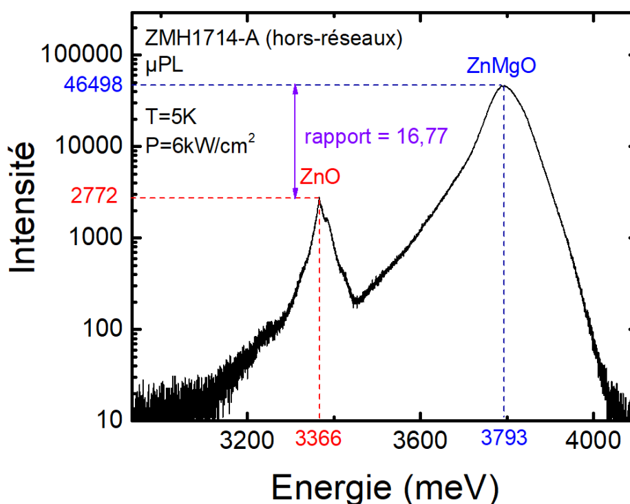
Figure III – 7. Spectres de \mu PL du guide ZMH1714-A, réalisés hors-réseau à 5K et à faible puissance d'excitation P = 6W \cdot cm^{-2} avec le laser Q-Switched. Le rapport des intensités des pics de ZnO et de ZnMgO est de 16,77.
