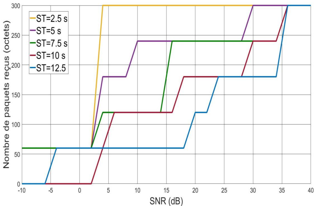
Figure IV. 24: Nombre de paquets reçus en présence du bruit balayant la bande 2.4 GHz - 2.410 GHz
