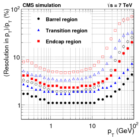
FIG. 3.5: Résolution en impulsion transverse des traces reconstruites [67].
