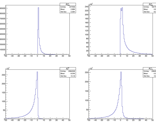
FIG. B.4: Distribution pour A^{ZZ}
