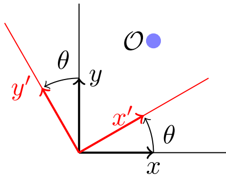
(a) Transformation observateur (passive) où le repère est modifié mais le phénomène est inchangé.
