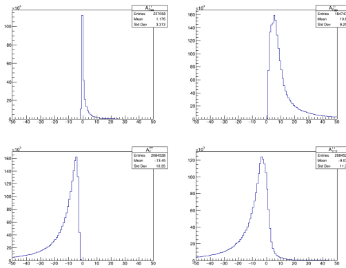
FIG. B.1: Distribution pour A^{TT}
