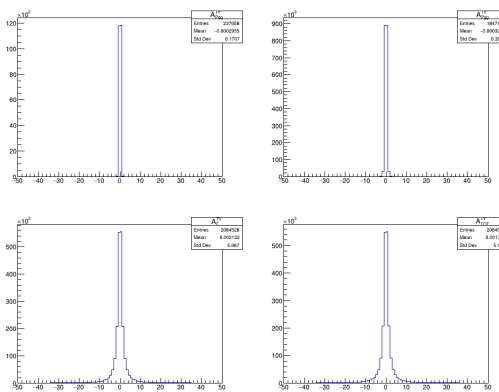
FIG. B.6: Distribution pour A^{TY} et A^{YT}
