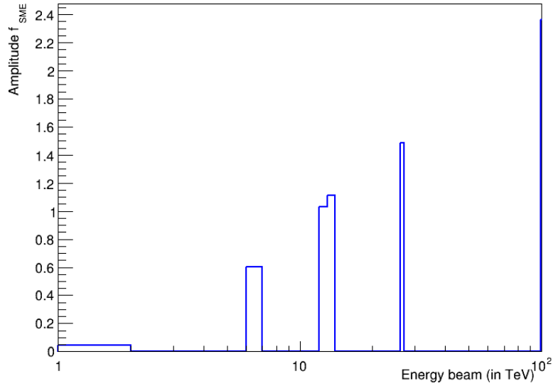
FIG. 2.15: Amplitude de f(t) pour le Tevatron, LHC, HL-LHC, HE-LHC et FCC, pour c_{\text{LXX}} = -c_{\text{LYY}} = 0.01 , pour des évènements générés sans PDF.
