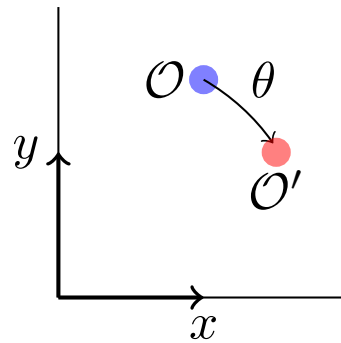
(b) Transformation particule (active) où le repère est inchangé mais le phénomène est transformé.
