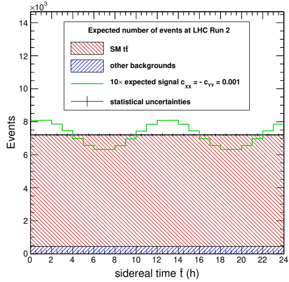
FIG. 2.12: Distribution du nombre d'évènements t\bar{t} avec 1 bin pour 1 heure sidérale [53].
