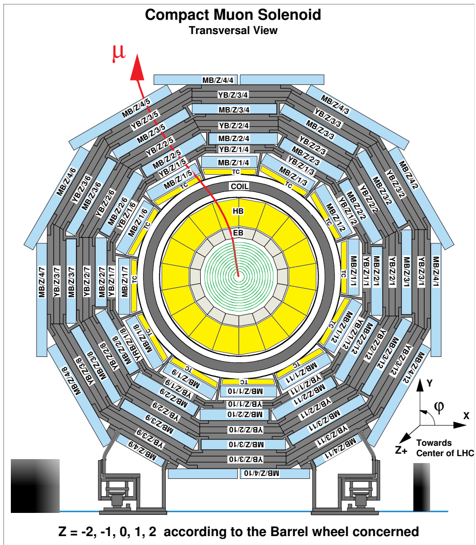
FIG. 3.12: Agencement des tubes à dérives dans le tonneau de CMS (vue transversale). Chaque rectangle bleu correspond à un tube à dérive.
