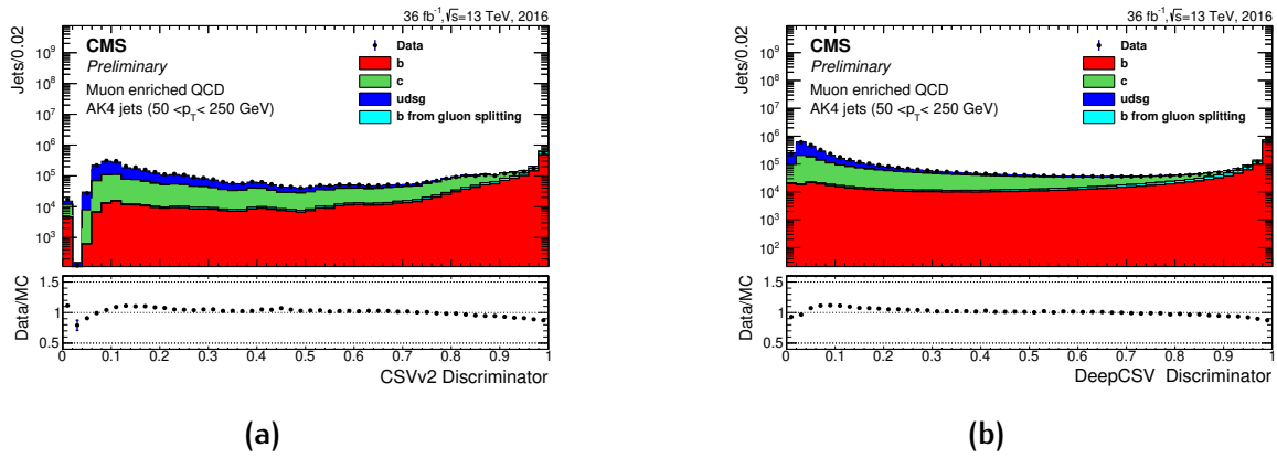
FIG. 4.5: Distribution des algorithmes de CSVv2 (a) et de DeepCSV (b).
