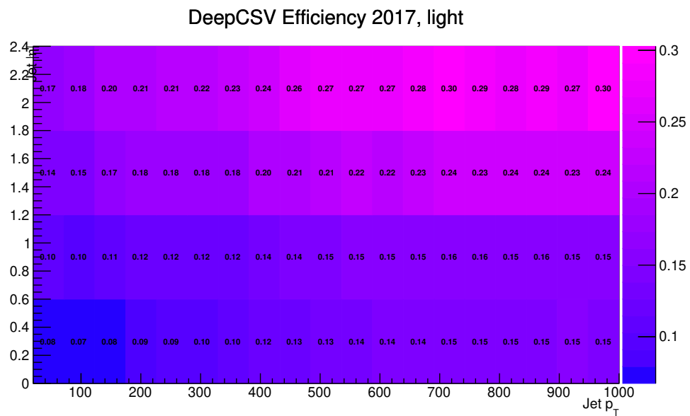
FIG. C.13: Histogramme 2D des facteurs correctifs pour l'efficacité de l'étiquetage des lights jets avec l'algorithme DeepCSV. L'abscisse est l'impulsion transverse p_T du jet considéré et l'ordonnée est sa pseudo-rapidité en valeur absolue |\eta| .
