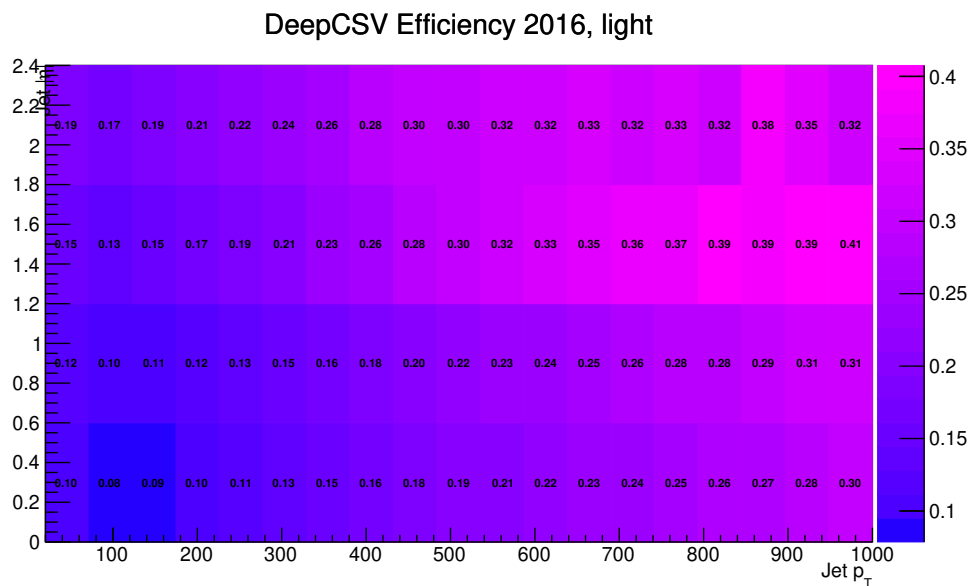
FIG. C.11: Histogramme 2D des facteurs correctifs pour l'efficacité de l'étiquetage des lights jets avec l'algorithme DeepCSV. L'abscisse est l'impulsion transverse p_T du jet considéré et l'ordonnée est sa pseudo-rapidité en valeur absolue |\eta| .
