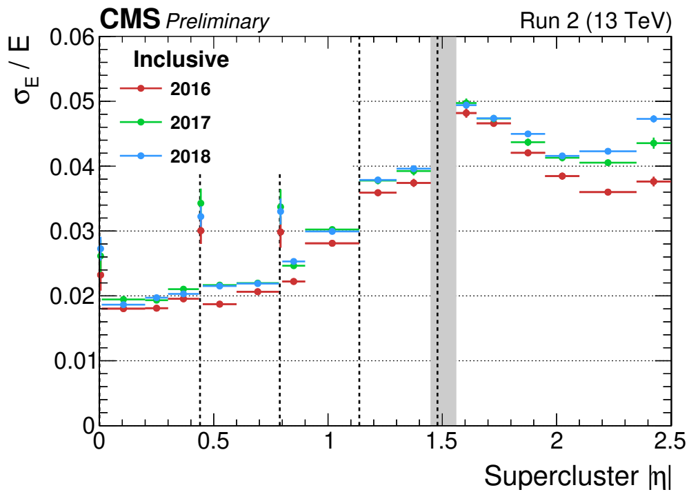
FIG. 3.9: Résolution relative du ECAL lors du Run II en fonction de la position angulaire \eta du super-cluster des électrons issus des désintégrations Z \rightarrow e^-e^+ [69].
