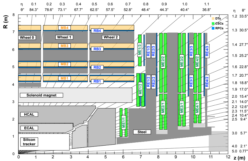
FIG. 3.11: Vue longitudinale des chambres à muons [65].
