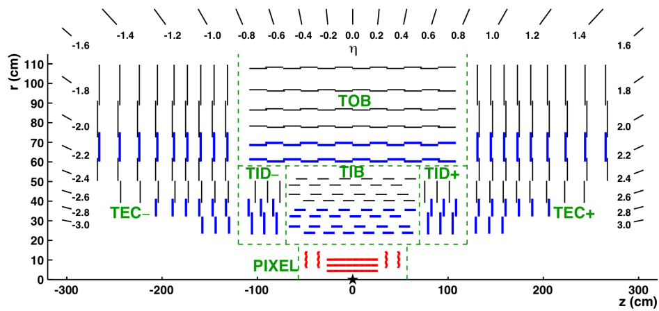
FIG. 3.6: Vue détaillée du trajectographe de l'expérience CMS [65].
