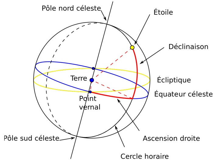
FIG. 2.6: Point Vernal quand le soleil passe de l'hémisphère Sud au Nord
