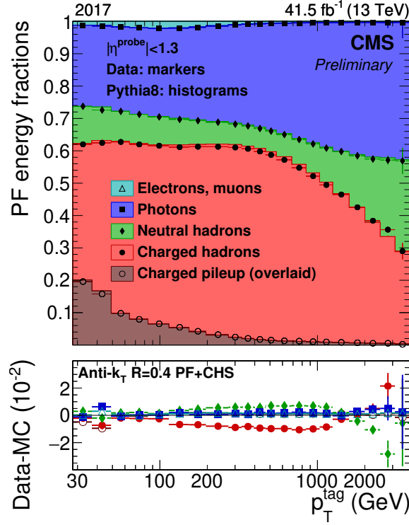
FIG. 4.3: Composition des jets reconstruits à l'aide de l'algorithme anti-k_T en fonction de p_T du jet avec un \Delta R = 0.4 dans des événements dijet sur l'année 2017.
