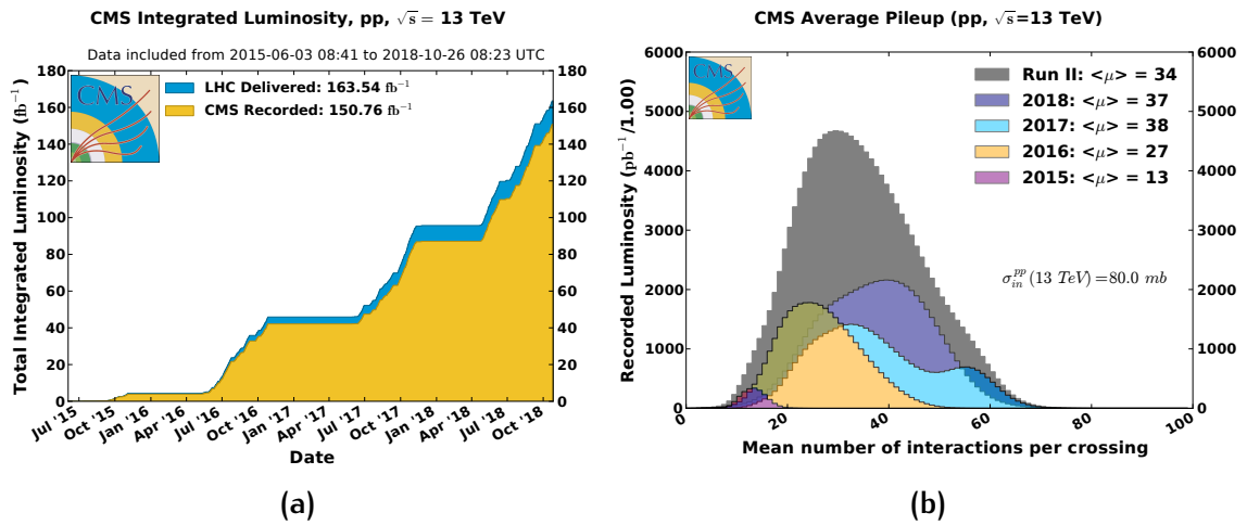
FIG. 3.2: (a) Luminosité intégrée collectée par l'expérience CMS au cours du Run II du LHC. (b) Nombre moyen d'interactions par croisement de faisceaux observées pendant la prise de données de différentes années du Run II.
