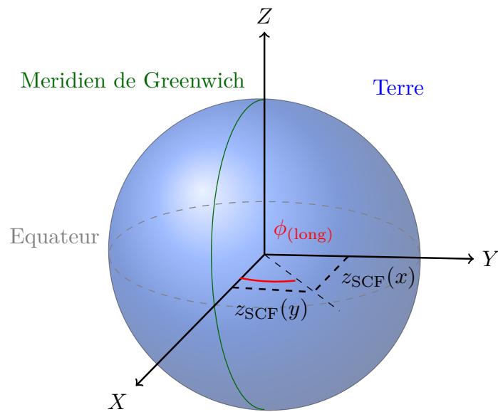
FIG. 2.8: Schéma de la longitude effective.
