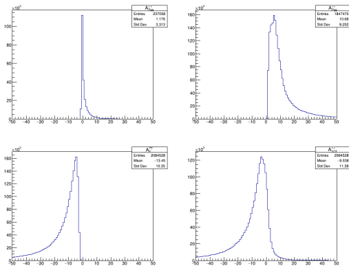
FIG. B.1: Distribution pour A^{TT}
