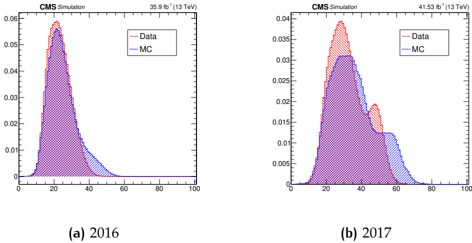
FIG. 5.3: Nombre d'empilement des données observées et simulées normalisé à 1 pour le processus t\bar{t} pour l'année (a) 2016 et (b) 2017, ramené à une luminosité de \mathcal{L} = 1 \text{ fb}^{-1} .
