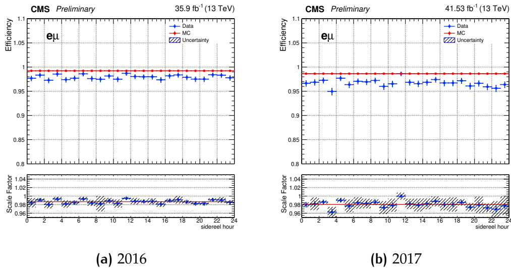
FIG. 5.4: Comparaison de l'efficacité des chemins de déclenchement e\mu fonction du temps sidéral pour l'année (a) 2016 et (b) 2017. Les facteurs correctifs ainsi que leurs incertitudes sont également présentés.
