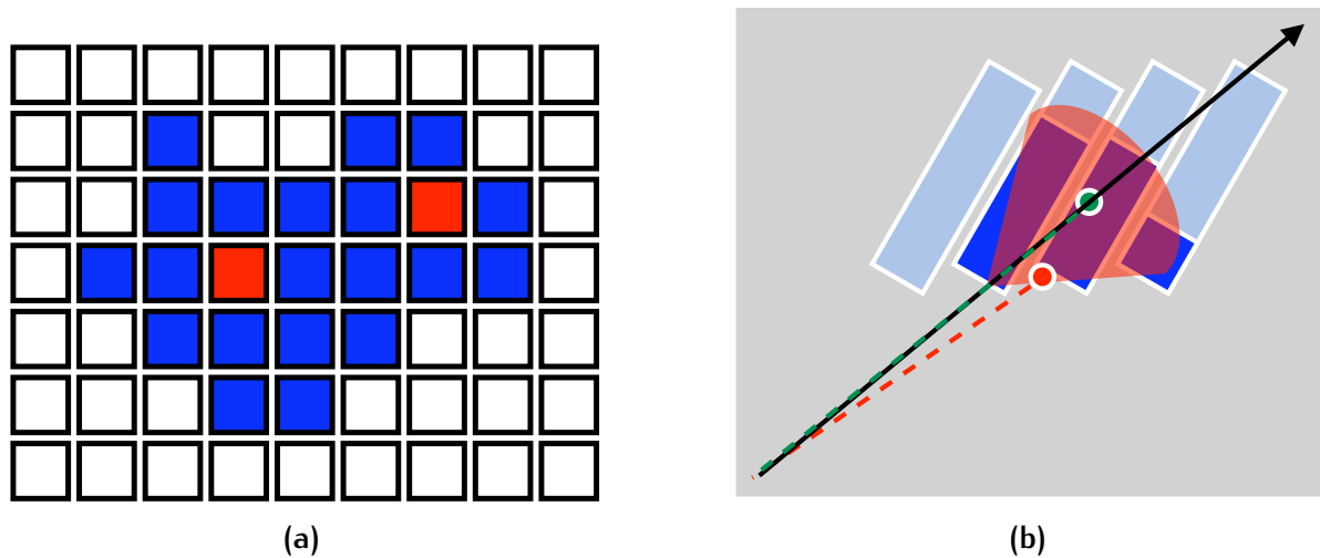
FIG. 4.2: Agglomérat topologique contenant deux graines (a) et détermination de la profondeur du dépôt d'énergie (b). En rouge, la position déterminée sans tenir compte de la profondeur biaisée |\eta| . En vert, la profondeur est correctement estimée.
