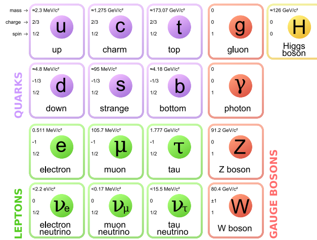
FIG. 1.1: Les particules élémentaires du Modèle Standard.
