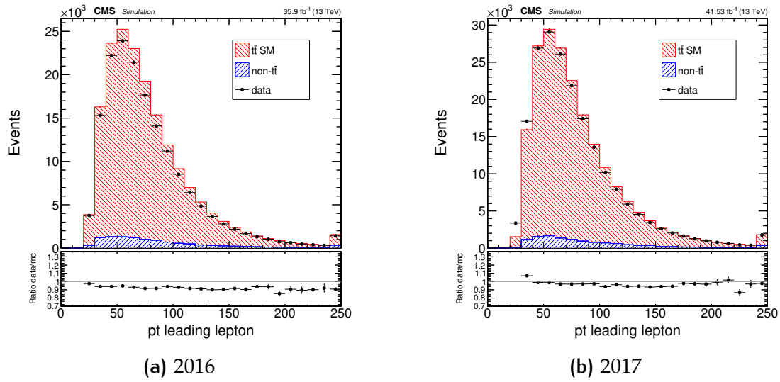
FIG. C.14: Comparaison données/Monte-Carlo pour le p_T du lepton leader pour l'année (a) 2016 et (b) 2017.
