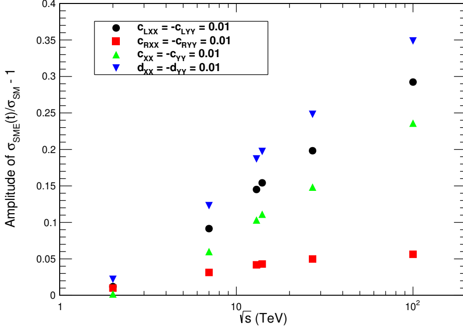
FIG. 2.14: Amplitude de f(t) pour le Tevatron, LHC, HL-LHC, HE-LHC et FCC, pour c_{XX} = -c_{YY} = 0.01 [53].
