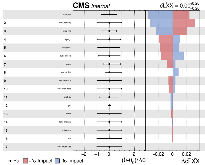
FIG. 5.15: Graphe d'impact des paramètres de nuisances sur la mesure du coefficient de Wilson c_{LXX} en cas de test Asimov pour l'année 2016. Les valeurs sont à multiplier par un facteur 10^{-3} , autrement dit le graphe indiquant \Delta c = 2.4 \times 10^{-1} signifie le résultat \Delta c = 2.4 \times 10^{-4} .
