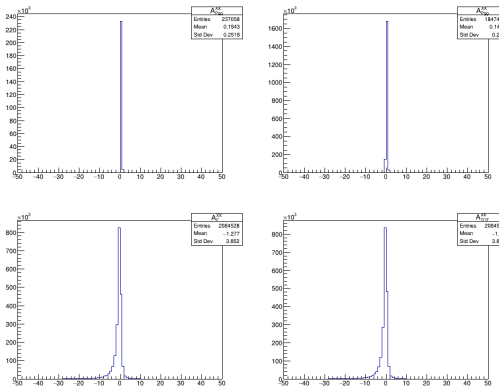
FIG. B.2: Distribution pour A^{XX}
