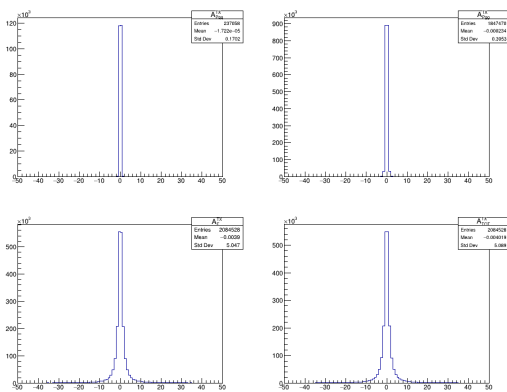
FIG. B.5: Distribution pour A^{TX} et A^{XT}
