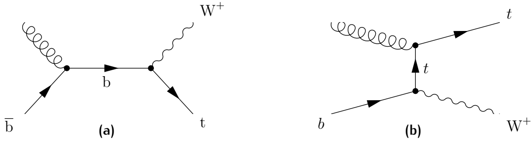
FIG. 2.3: Diagrammes de Feynman de la production associée d'un quark top célibataire et d'un boson W (voie tW).
