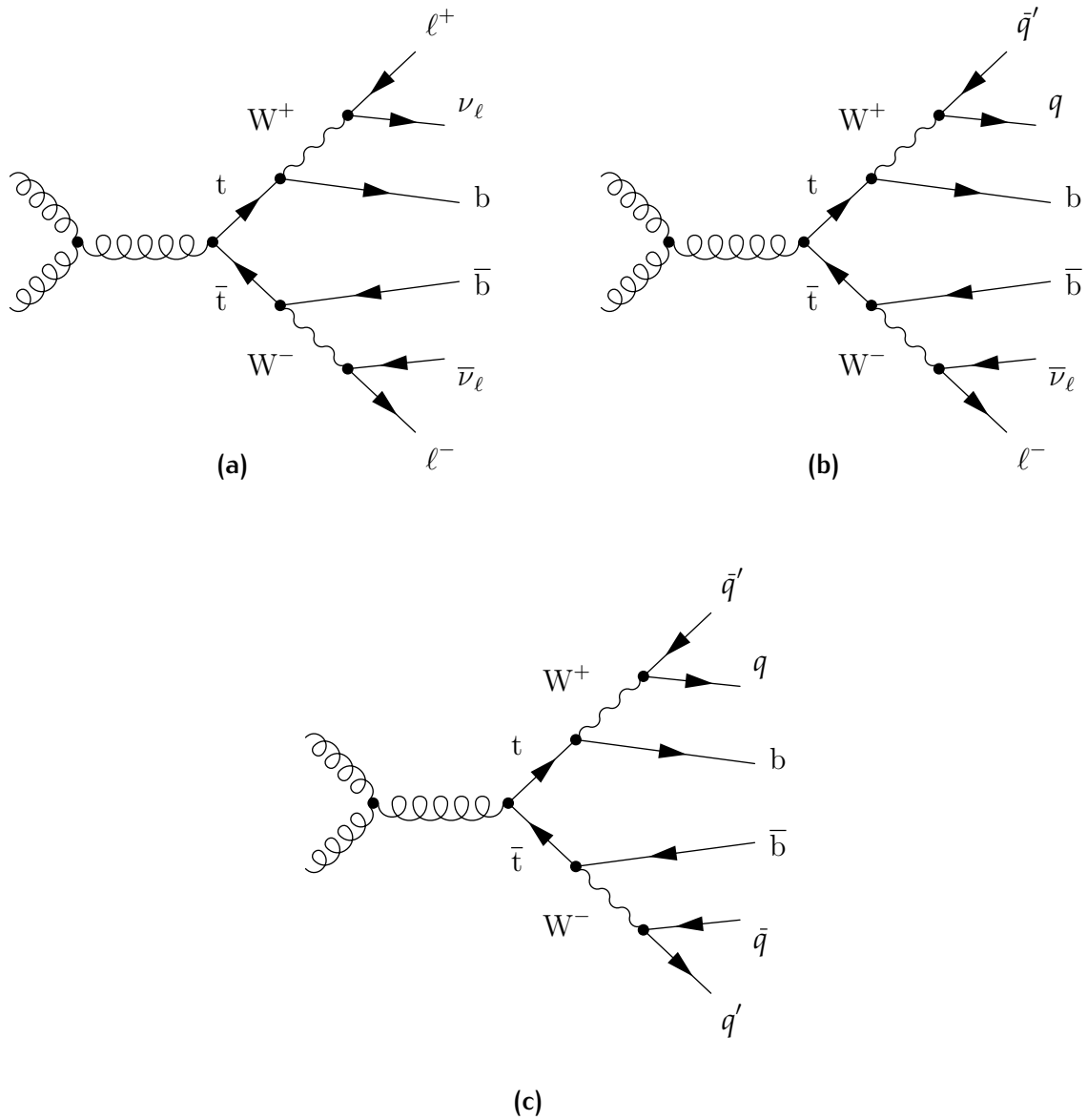
FIG. 2.5: Diagrammes de Feynman de la désintégration d'une paire t\bar{t} dans (a) le canal di-leptonique, (b) le canal semi-leptonique, ainsi que (c) le canal tout-hadronique.
