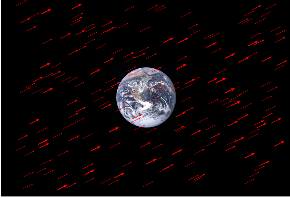
FIG. 1.7: Représentation de la Terre plongée dans un espace comportant un champ additionnel orienté constant, symbolisé par des flèches rouges.
