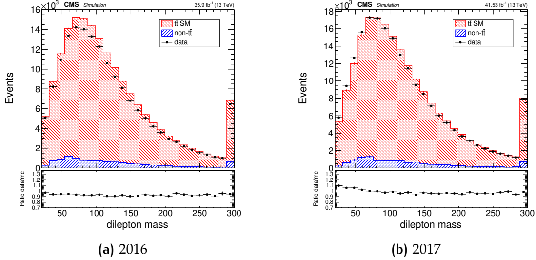
FIG. 5.11: Comparaison données/Monte-Carlo pour la masse dilepton pour l'année (a) 2016 et (b) 2017.
