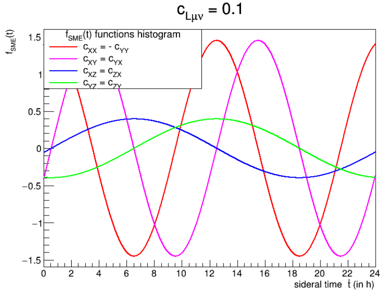
FIG. 2.11: Tracé des fonction f(t) pour les différents couples de coefficient gauche non-nuls dans le scenario LHC 13 TeV.
