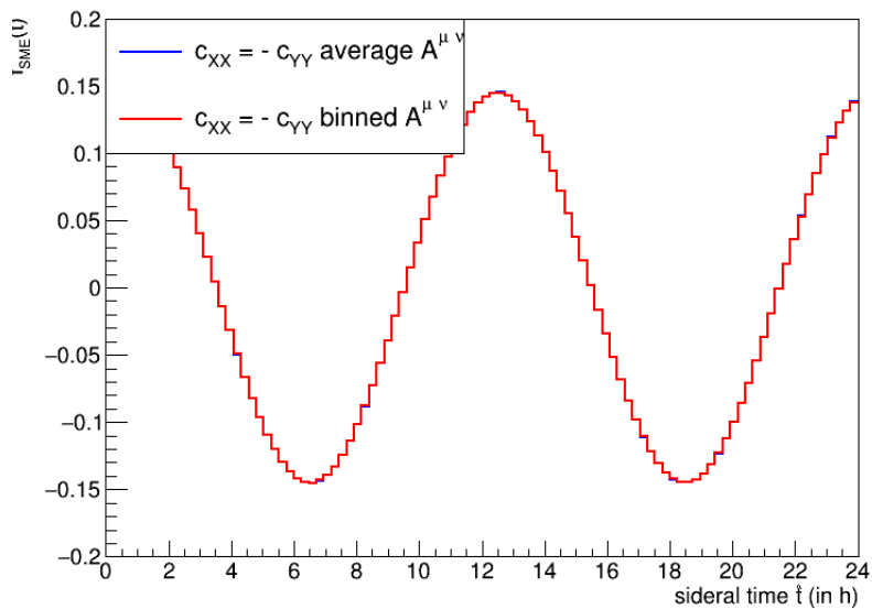
FIG. B.15: Moyenne de la composante cinétique en 100 bins
