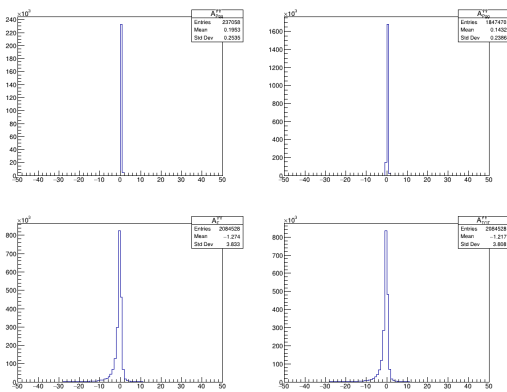
FIG. B.3: Distribution pour A^{YY}
