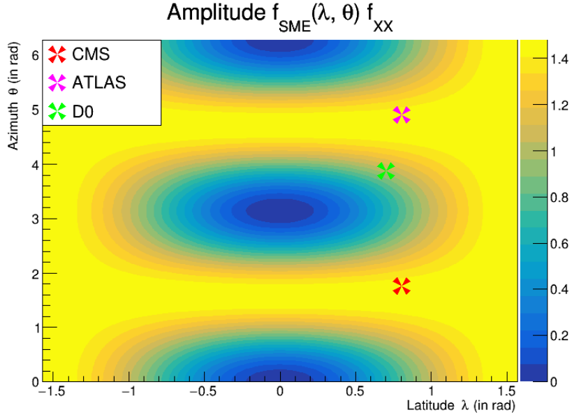
FIG. 2.16: Amplitude de f(\lambda, \theta) en fonction de la latitude et de l'azimut pour c_{XX} = -c_{YY} dans un scénario à 13 TeV avec les orientations de détecteurs CMS, ATLAS et D0 [55].
