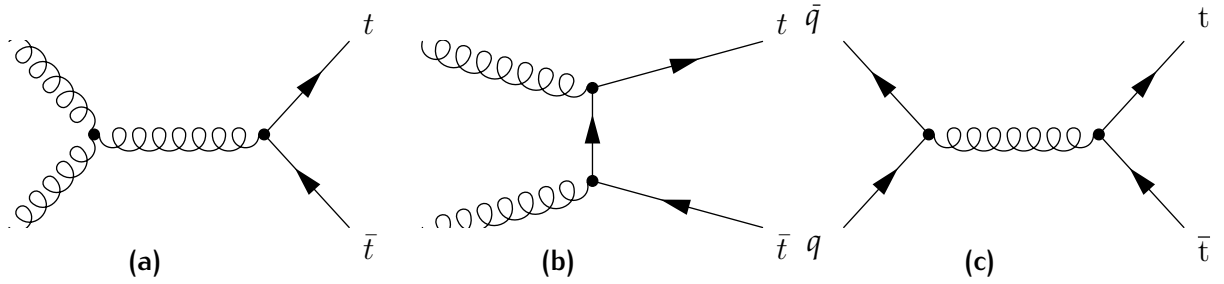
FIG. 2.1: Diagrammes de Feynman de production de paires t\bar{t} par fusion de gluons (a, b), ainsi que par annihilation de quarks (c).
