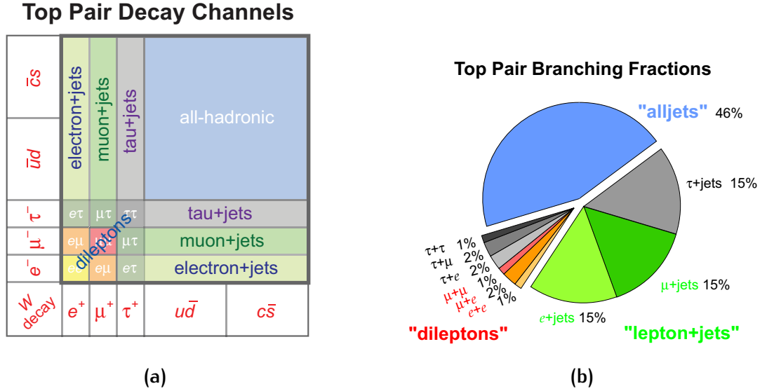
FIG. 2.4: Canaux de désintégration d'une paire t\bar{t} (a) et rapports d'embranchements des différents canaux de désintégration d'une paire t\bar{t} (b).
