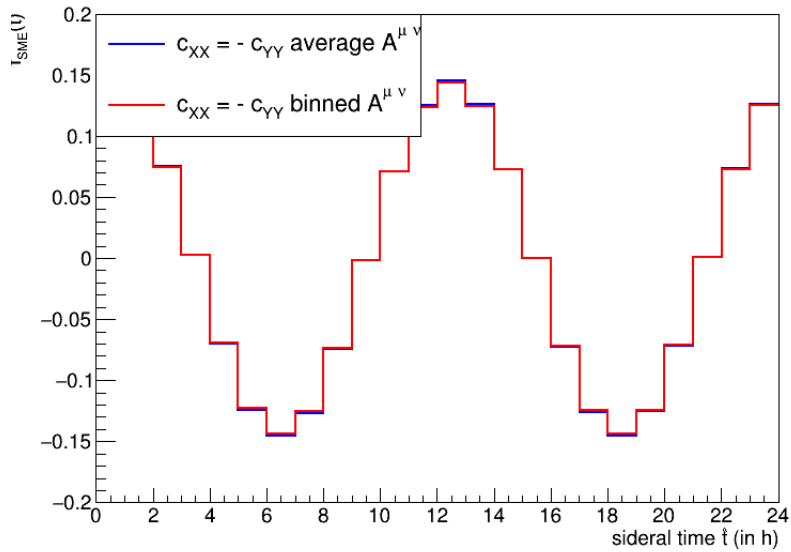
FIG. B.14: Moyenne de la composante cinétique en 24 bins
