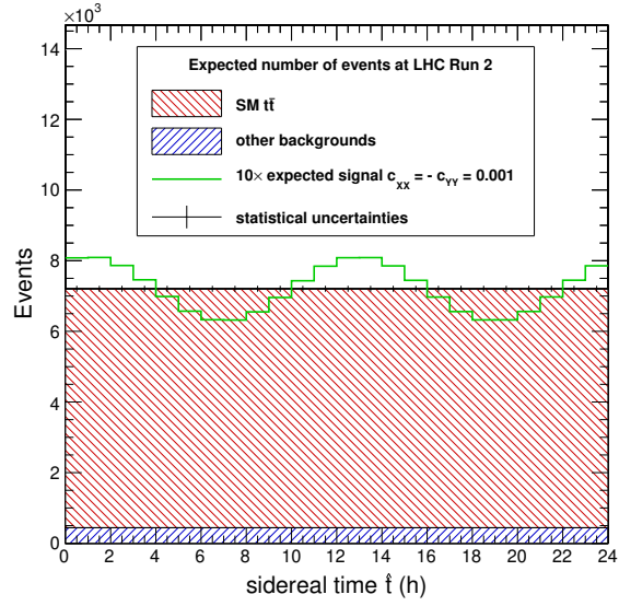
FIG. 2.12: Distribution du nombre d'évènements t\bar{t} avec 1 bin pour 1 heure sidérale [53].
