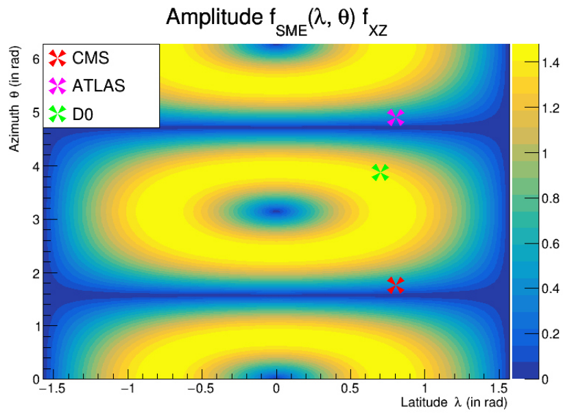
FIG. B.16: Amplitude de f(\lambda, \theta) en fonction de la latitude et de l'azimut pour c_{XZ} = c_{ZX} dans un scénario à 13 TeV avec les orientations de détecteurs CMS, ATLAS et D0.
