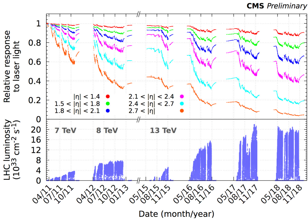
FIG. 3.8: Réponse relative des cristaux du ECAL en fonction du temps, pour différentes zones en |\eta| ( haut ) et luminosité instantanée du LHC ( bas ) [68].
