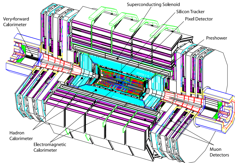
FIG. 3.3: Vue en perspective du détecteur CMS et de ses sous-détecteurs [65].
