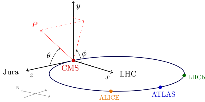
FIG. 3.4: Système de coordonnées du détecteur CMS par rapport à l'anneau du LHC [65].
