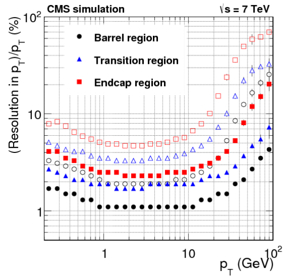
FIG. 3.5: Résolution en impulsion transverse des traces reconstruites [67].
