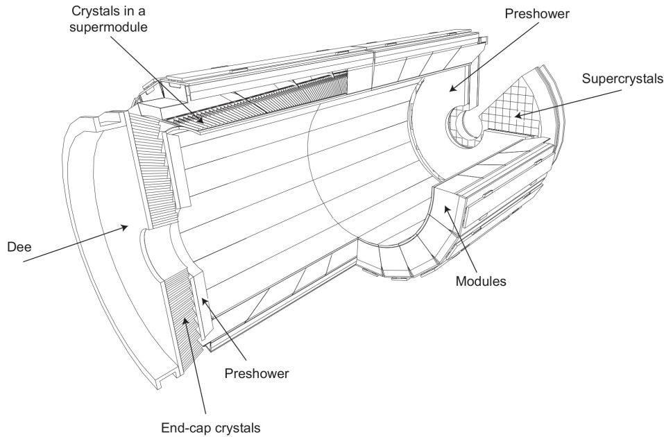
FIG. 3.7: Vue en perspective du calorimètre électromagnétique et de ses sous-éléments [65].
