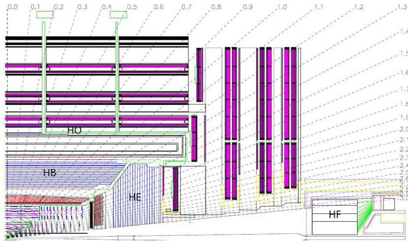
FIG. 3.10: Vue longitudinale du calorimètre hadronique [65].
