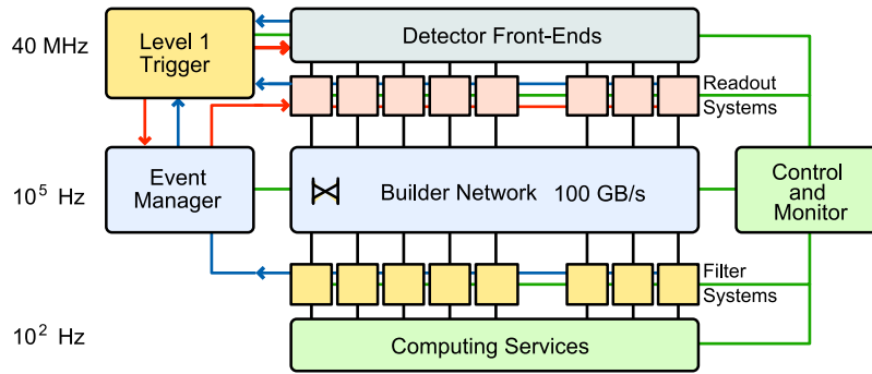
FIG. 3.14: Schéma de la chaîne d'acquisition de données de CMS
