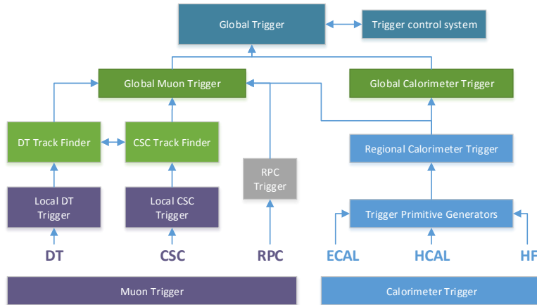
FIG. 3.13: L'architecture du déclencheur de niveau 1
