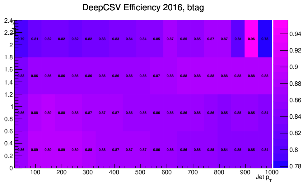
FIG. C.9: Histogramme 2D des facteurs correctifs pour l'efficacité de l'étiquetage b avec l'algorithme DeepCSV. L'abscisse est l'impulsion transverse p_T du jet considéré et l'ordonnée est sa pseudo-rapidité en valeur absolue |\eta| .
