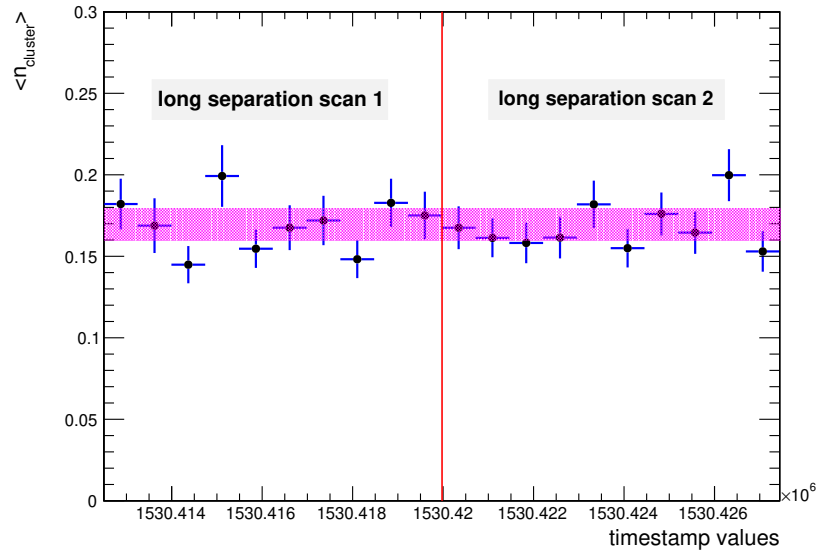
FIG. 3.15: Incertitude systématique du comptage de clusters de pixels avec \langle n_{\text{cluster}} \rangle en fonction du temps, pour les deux scans à longue séparation.
