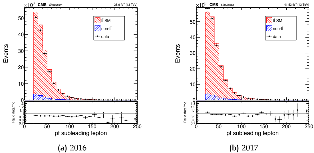
FIG. C.15: Comparaison données/Monte-Carlo pour le p_T du lepton subleader pour l'année (a) 2016 et (b) 2017.
