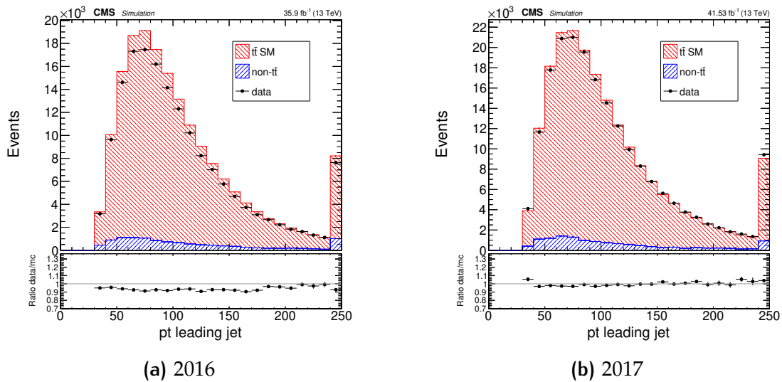
FIG. C.19: Comparaison données/Monte-Carlo pour le p_T du jet leader pour l'année (a) 2016 et (b) 2017.
