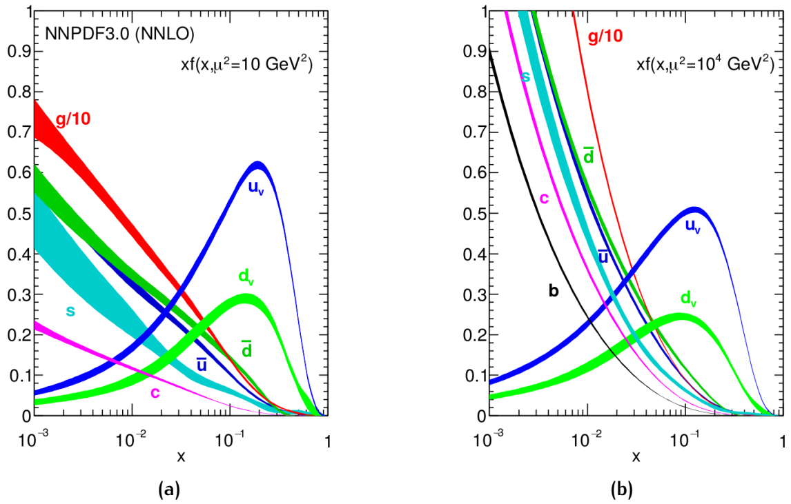
FIG. 1.4: Fonctions de densité partonique pour une échelle en énergie (a) \mu^2 (= Q^2) = 10 \text{ GeV}^2 et (b) \mu^2 (= Q^2) = 10^4 \text{ GeV}^2 [23].
