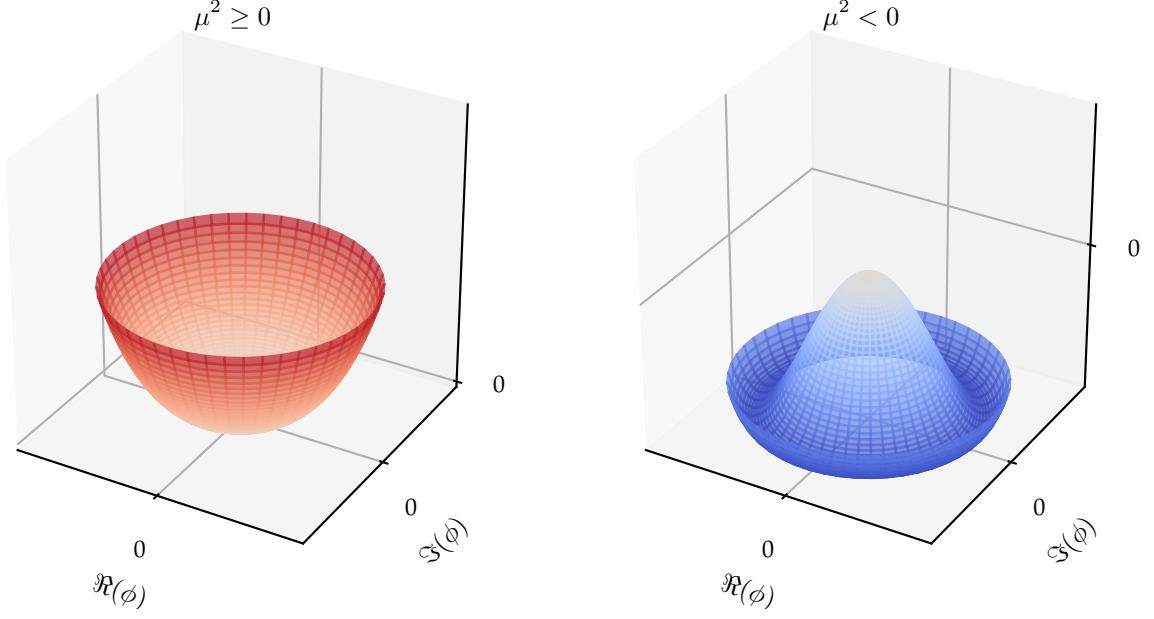
FIG. 1.2: Forme du potentiel de Higgs V selon le signe de \mu
