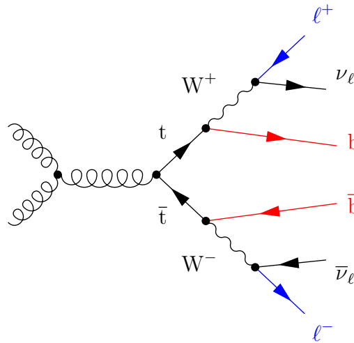
FIG. 5.1: Diagramme de Feynman du processus t\bar{t} dans le canal dilepton. Les produits caractéristiques de ce canal portent les couleurs bleue pour les leptons et rouge pour les quarks b.
