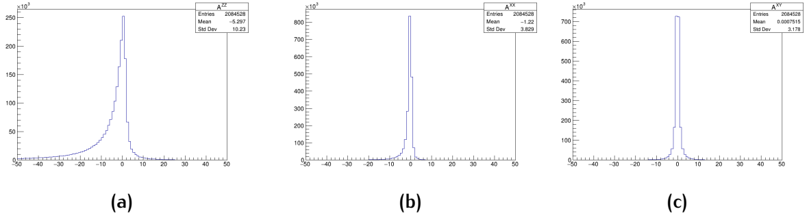
FIG. 2.10: Histogramme de valeur des composantes de la matrice A_{TOT}^{\mu\nu} = \frac{\Gamma_{q\bar{q}}}{2} A_{q\bar{q}}^{\mu\nu} + \frac{\Gamma_{gg}}{2} A_{gg}^{\mu\nu} + A_F^{\mu\nu} pour \mu\nu = ZZ (a), XX (b) et XY (c).
