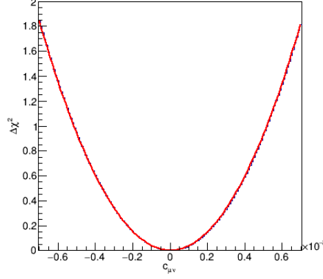
FIG. 2.13: Méthode \chi^2 pour l'évaluation du coefficient c_{LXX} = -c_{LYY} .
