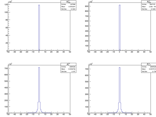
FIG. B.8: Distribution pour A^{XY} et A^{YX}
