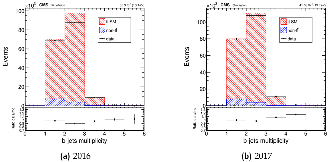
FIG. C.16: Comparaison données/Monte-Carlo pour le nombre de jets étiqueté b pour l'année (a) 2016 et (b) 2017.
