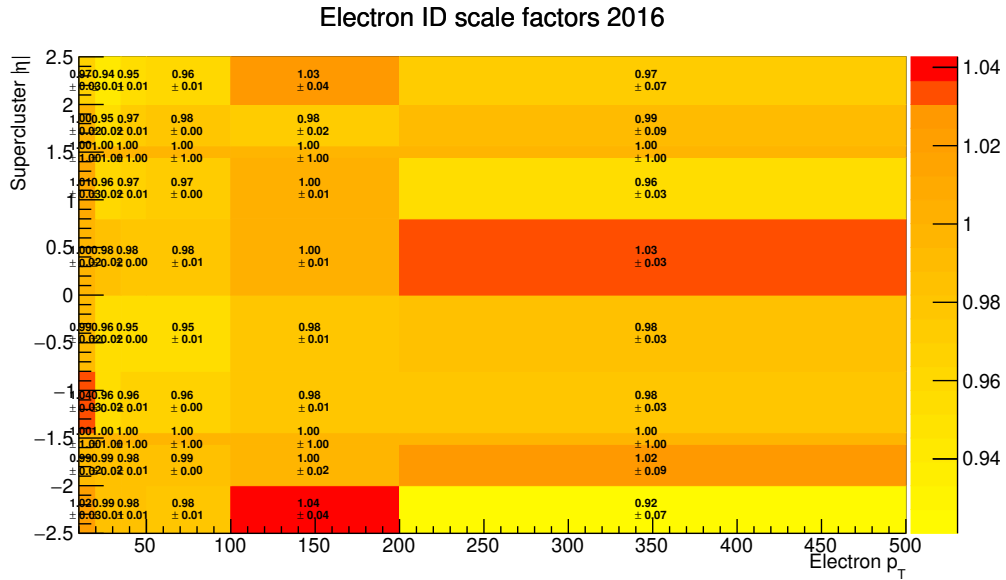
FIG. C.1: Histogramme 2D des facteurs correctifs d'identification des électrons pour l'année 2016. L'abscisse est l'impulsion transverse p_T du jet considéré et l'ordonnée est sa pseudo-rapacité en valeur absolue |\eta| .
