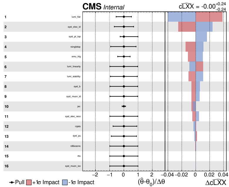
FIG. 5.16: Graphe d'impact des paramètres de nuisances sur la mesure du coefficient de Wilson c_{LXX} en cas de test Asimov pour l'année 2017. Les valeurs sont à multiplier par un facteur 10^{-3} , autrement dit le graphe indiquant \Delta c = 2.4 \times 10^{-1} signifie le résultat \Delta c = 2.4 \times 10^{-4} .
