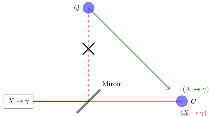
FIG. 1.5: Expérience de pensée menant au paradoxe d'un phénomène qui s'est à la fois produit et pas produit en même temps.
