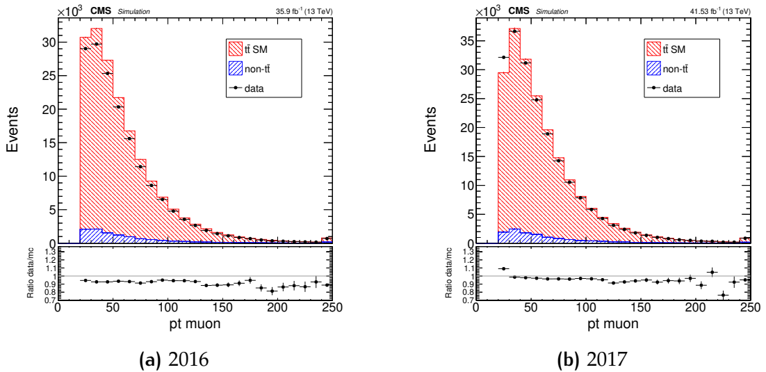
FIG. C.17: Comparaison données/Monte-Carlo pour le p_T du muon pour l'année (a) 2016 et (b) 2017.
