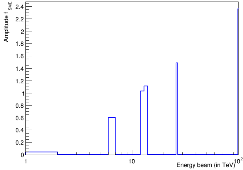
FIG. 2.15: Amplitude de f(t) pour le Tevatron, LHC, HL-LHC, HE-LHC et FCC, pour c_{LXX} = -c_{LYY} = 0.01 , pour des évènements générés sans PDF.
