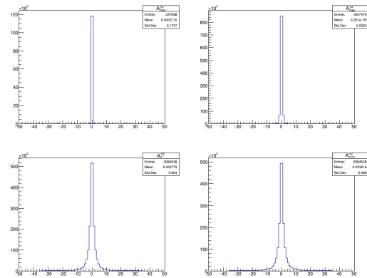
FIG. B.10: Distribution pour A^{YZ} et A^{ZY}
