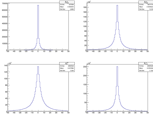
FIG. B.7: Distribution pour A^{TZ} et A^{ZT}
