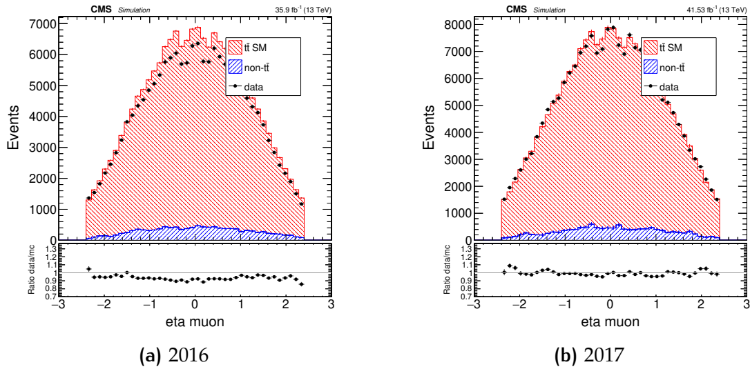
FIG. C.18: Comparaison données/Monte-Carlo pour le \eta du muon pour l'année (a) 2016 et (b) 2017.
