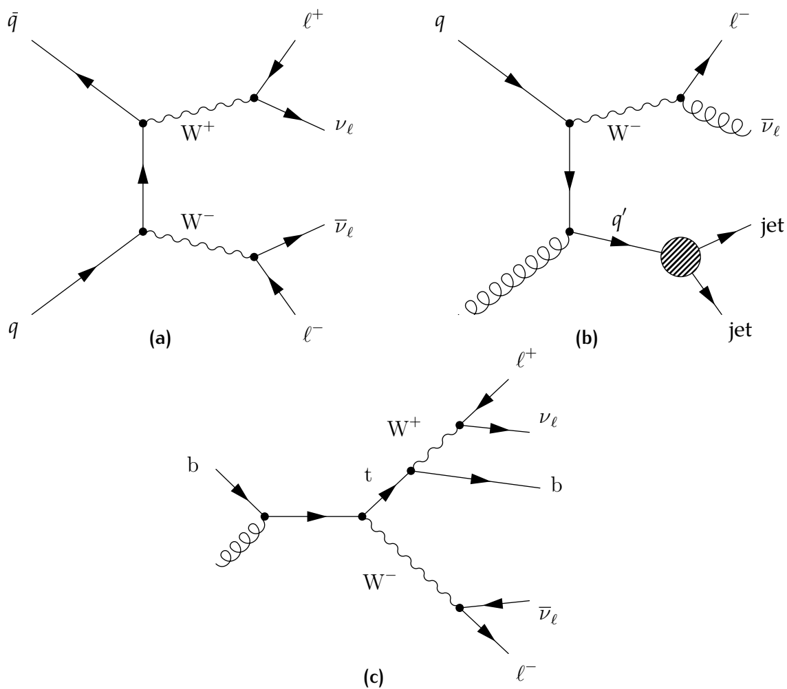
FIG. 5.2: Diagrammes de Feynman des processus de bruit de fond de (a) WW, (b) W + jets et (c) top solitaire dans le canal tW.
