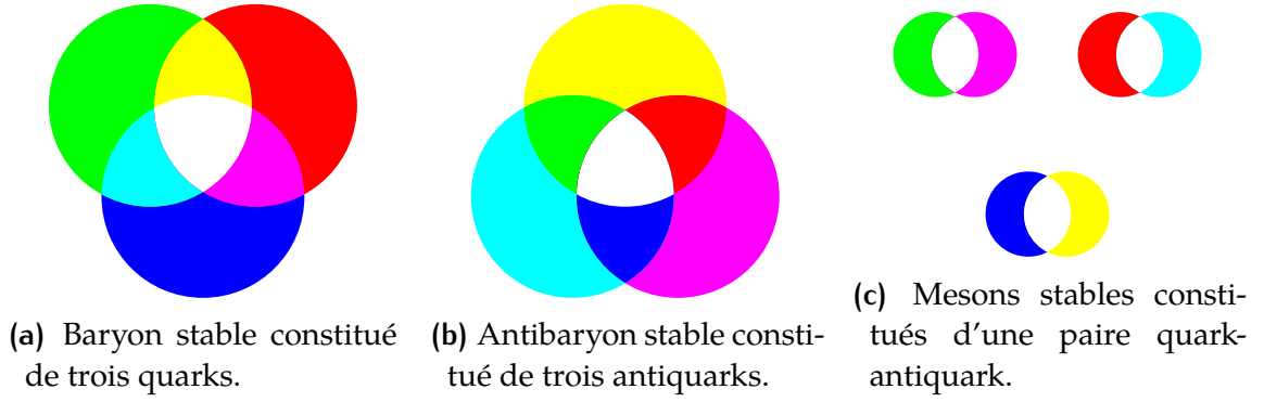
FIG. 1.3: Représentation de hadrons stables à l'interaction de couleur (blanche).
