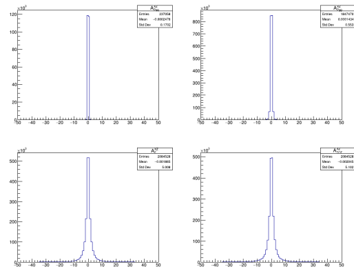
FIG. B.9: Distribution pour A^{XZ} et A^{ZX}
