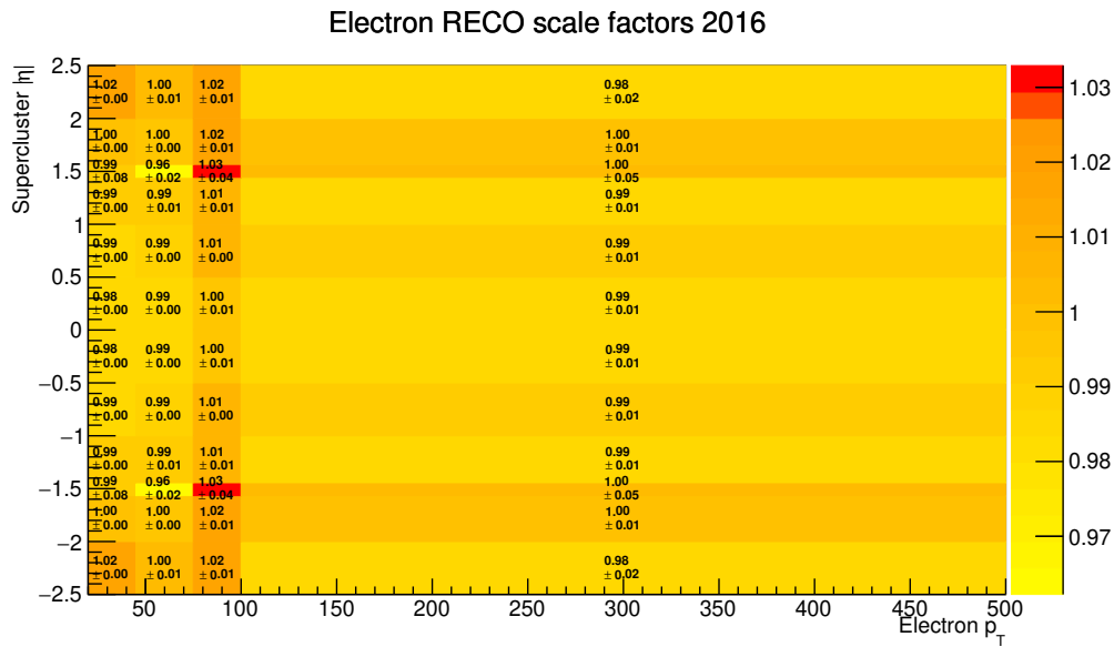
FIG. C.2: Histogramme 2D des facteurs correctifs de reconstructions des électrons pour l'année 2016. L'abscisse est l'impulsion transverse p_T du jet considéré et l'ordonnée est sa pseudo-rapidité en valeur absolue |\eta| .
