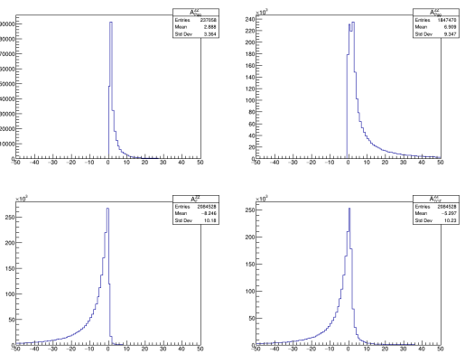
FIG. B.4: Distribution pour A^{ZZ}
