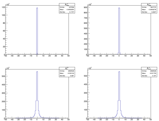
FIG. B.6: Distribution pour A^{TY} et A^{YT}
