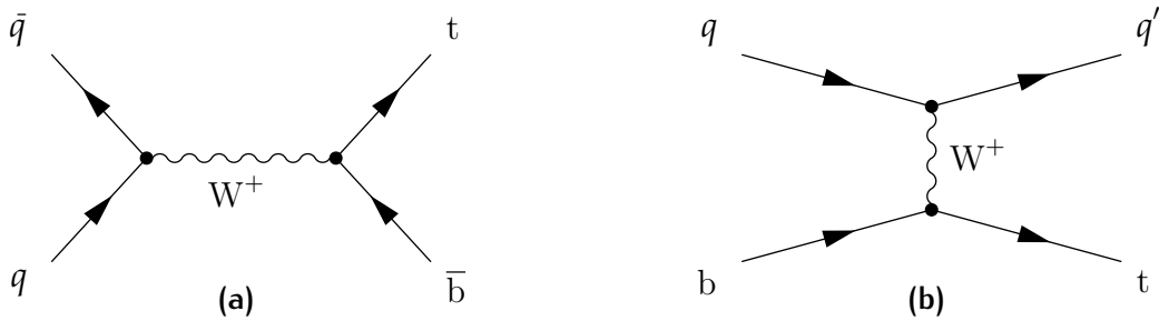
FIG. 2.2: Diagrammes de Feynman de la production de quark top célibataire, en voie s (a) et en voie t (b).
