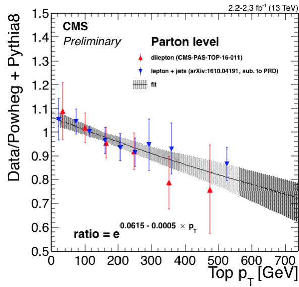
FIG. 5.5: Histogramme présentant l'écart en p_T dans les échantillons avec quark t avec la mesure dans les données.
