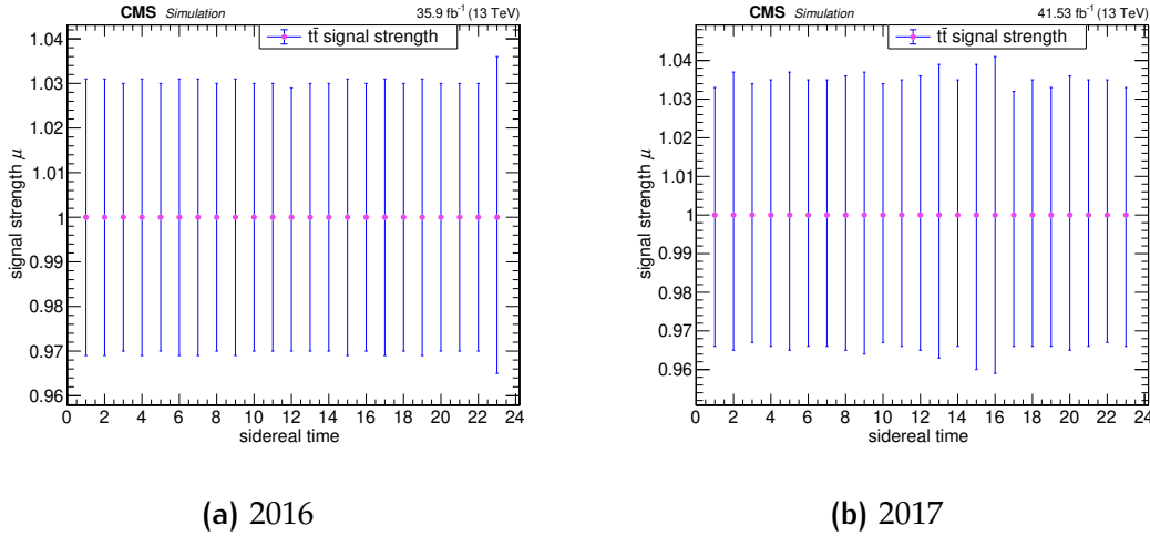
FIG. 5.13: Mesure différentielle de l'intensité du signal \mu de la masse dilepton au cours du temps sidéral pour l'année (a) 2016 et (b) 2017, dans la simulation (lot de données Asimov)
