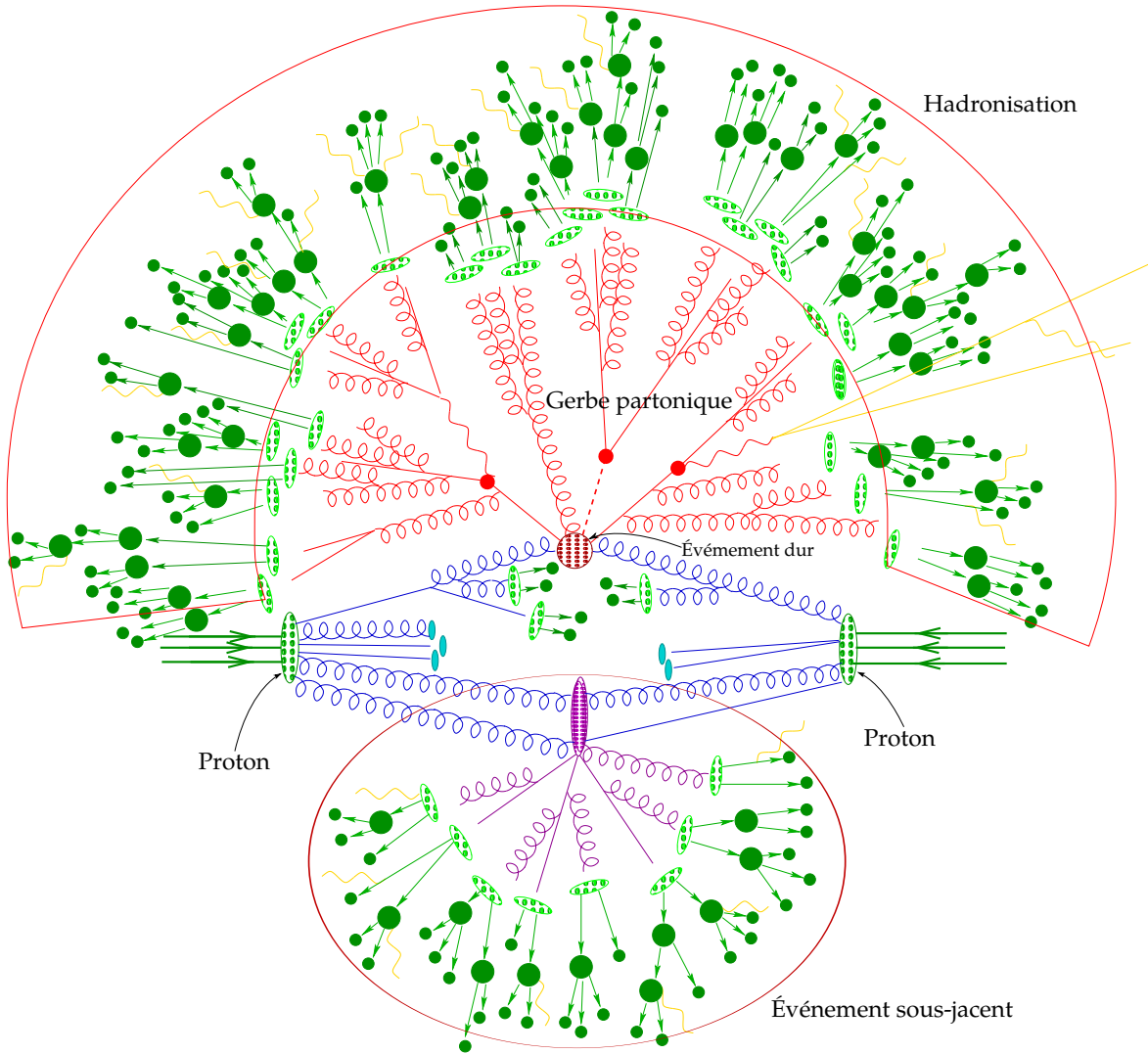
FIG. 4.1: Représentation graphique d'une collision de deux protons simulée à l'aide d'un générateur.
