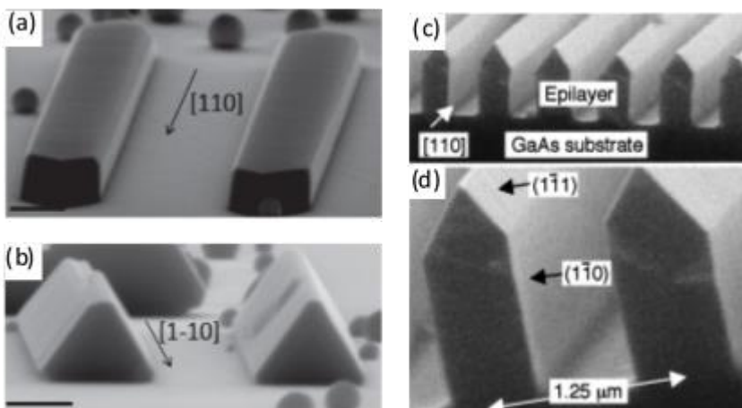
Figure 1.41 : Images MEB d'une croissance de 200 nm d'InP sur InP(001) avec des ouvertures dans le masque de 200 nm sur 4 μm (a-b) [102] et 2 μm de GaAs sur un substrat GaAs (001) avec masque SiO 2 de 1 μm de large (c-d) [101] . L'échelle sur les images a et b représente 200 nm.
