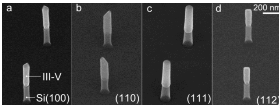
Figure 1.25 : Images MEB de nanopiliers InAs faits par TASE sur des substrats silicium orientés (a) [100], (b) [110], (c) [111] et (d) [112]. [75]
