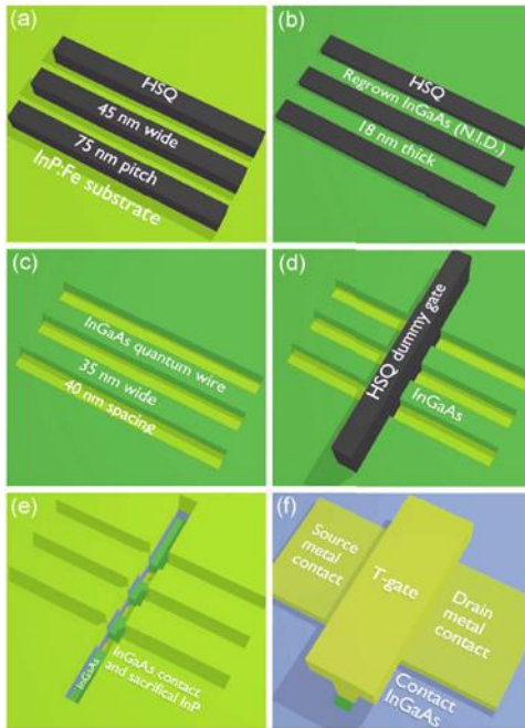
Figure 1.34 : Méthode de fabrication de MuGFETs par nano-impresseion de HSQ [90]
