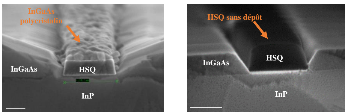
Figure 2.6 : Croissances localisées d'InGaAs sur substrat InP avec masque HSQ. À gauche, croissance sans utilisation d'hydrogène atomique ; à droite, croissance assistée par hydrogène atomique.
