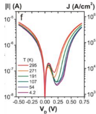
Figure 4.33 : Caractéristiques de la diode Esaki réalisée par Ganjipour et al [12] présentée dans le chapitre 1.
