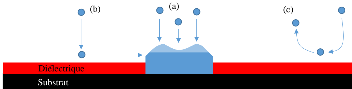
Figure 1.18 : Schéma de coupe d'une croissance sélective. (a) Les éléments cristallisent sur le substrat, dans les ouvertures ; Les éléments arrivant sur le masque sont adsorbés et diffusent jusque l'ouverture la plus proche (b), ou sont réévaporés (c). Les diffusions des éléments en surface du masque et sur les facettes latérales provoquent une accumulation de matériaux sur les facettes possédant les énergies de surface les plus faibles, représentée ici en clair.
