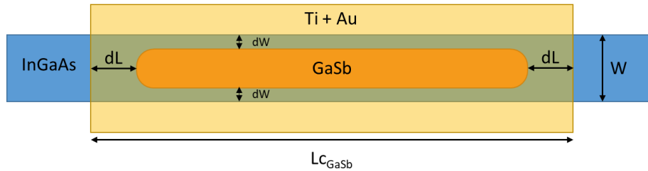
Figure 4.10 : Vue de dessus de la possible structure présente sous le contact de GaSb
