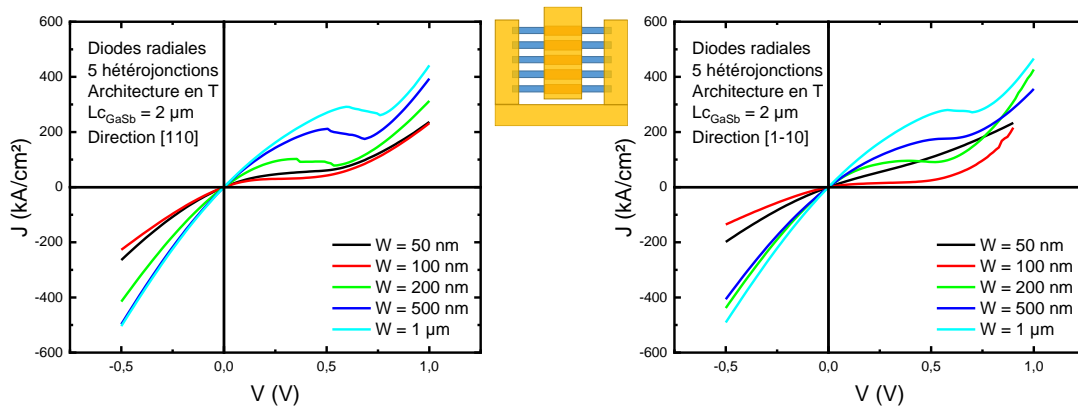
Figure 4.15 : Caractéristiques J=f(V) de diodes InGaAs/GaSb en T composées de réseaux de 5 hétérostructures. Le courant est normalisé par la jonction 5 * W * L_{cGaSb} .
