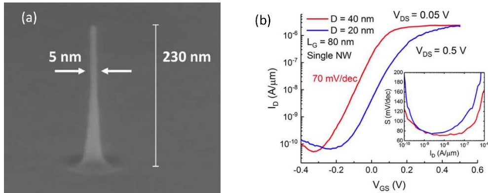
Figure 1.2: Exemple de nanofil vertical réalisé par gravure digitale (a) et caractéristique électrique (b) d'un composant de type MOSFET correspondant [4] .
