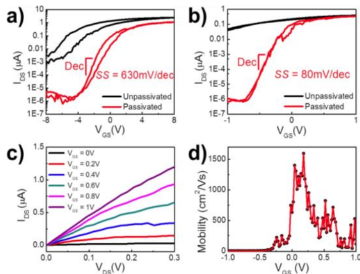
Figure 1.14 : Caractéristiques électriques du MOSFET de L.F. Shen et al [51] . (a) Caractéristique I_d(V_{gs}) pour une commande par grille arrière ; (b-d) Caractéristiques du composant pour une commande par grille enrobante.
