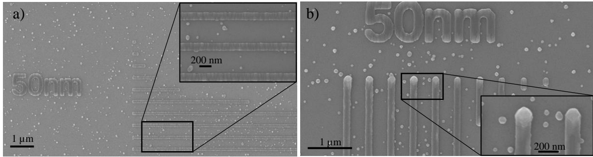
Figure 2.10 : Images MEB d'une croissance localisée suivant les directions [110] (a) et [1-10] (b) de 30 nm d' \text{InGaAs:Si} . La température de l'échantillon était de 470\text{ }^\circ\text{C} .
