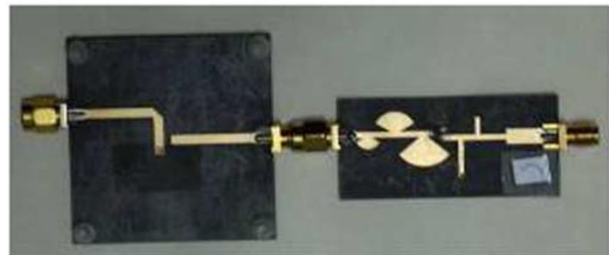
Figure I. 6: Photographie de la rectenna. 6
