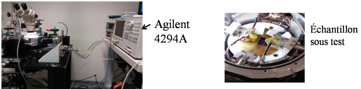
Figure III. 9: Banc expérimental de la mesure de spectroscopie d'admittance.
