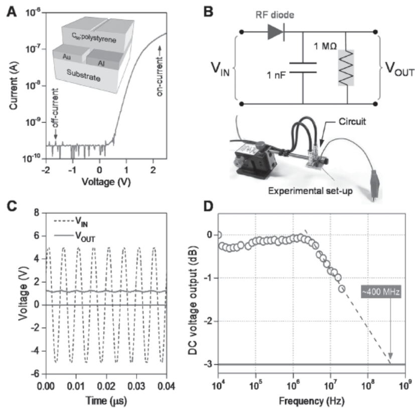
Figure I. 21: a) Caractéristique électrique de la diode utilisant le mélange C60 : PS, b) Circuit de redressement, c) Tension de sortie résultante à une fréquence de 13.56 MHz, d) tension de sortie en fonction de différentes fréquences montrant la fréquence de coupure. 32
