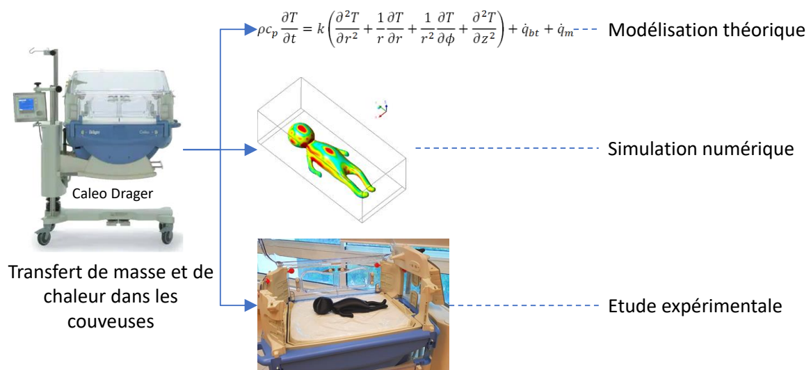
Figure 1.3: Schéma représentant les différentes méthodes utilisées pour l'analyse des transferts thermiques dans les couveuses de nouveau-nés
