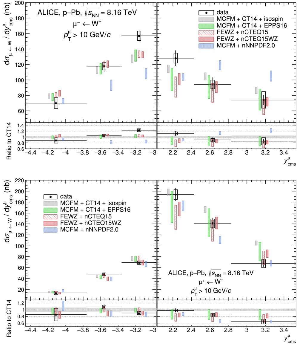
Figure 10: Section efficace de production du procédé W^{\pm} \rightarrow \mu^{\pm} \nu_{\mu} pour les bosons W^{-} (haut) et W^{+} (bas) en fonction de la rapidité, dans les collisions p-Pb à \sqrt{s_{\text{NN}}} = 8.16 TeV. Les mesures sont comparées avec des prédictions obtenues en utilisant plusieurs modèles de nPDF, ainsi qu'avec des prédictions obtenues avec le modèle de PDF libre CT14, incluant l'effet d'isospin mais sans modifications nucléaires. Les panneaux inférieurs de chaque figure indiquent le rapport entre les mesures et prédictions nucléaires, et les prédictions CT14. Les barres et boîtes autour des points expérimentaux correspondent respectivement aux incertitudes statistiques et systématiques, la bande grise dans les panneaux inférieurs indique l'incertitude sur les prédictions CT14. Les points expérimentaux sont centrés dans les intervalles en rapidité, les points théoriques sont décalés horizontalement pour une meilleure visibilité. xxix
