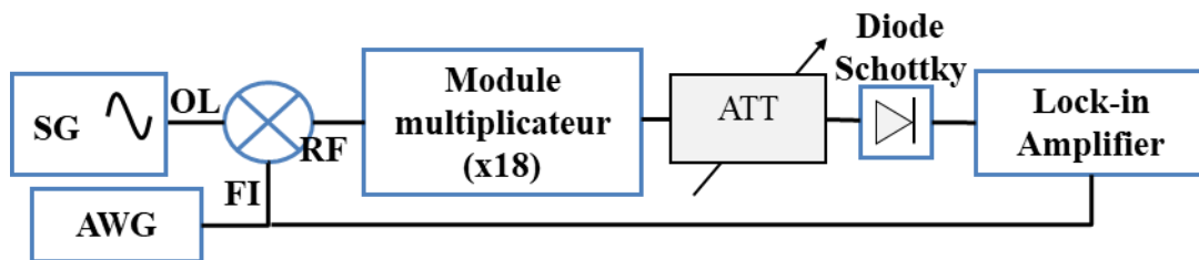
Figure 2.19: Schéma bloc de la calibration faite avec notre banc mesure.
