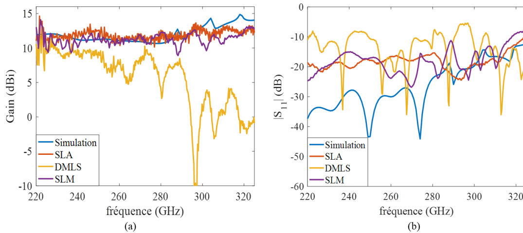
Figure 3.9: (a) Gain axial. (b) S_{11} . Simulés et mesurés de l'antenne cornet réalisée par SLA, DMLS et SLM.
