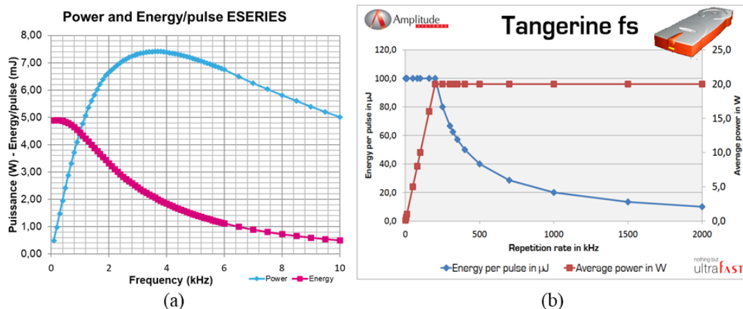
Figure 4.7: Évolution de la puissance moyenne et de l'énergie par pulse fonction du taux de répétition du laser (a) nanoseconde et (b) femtoseconde.
