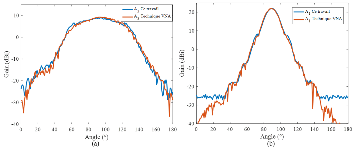
Figure 2.32: Diagrammes de rayonnement du plan H de A_1 (droite) et de A_3 (gauche) à 240 GHz entre notre technique de mesure et la technique de mesure VNA.
