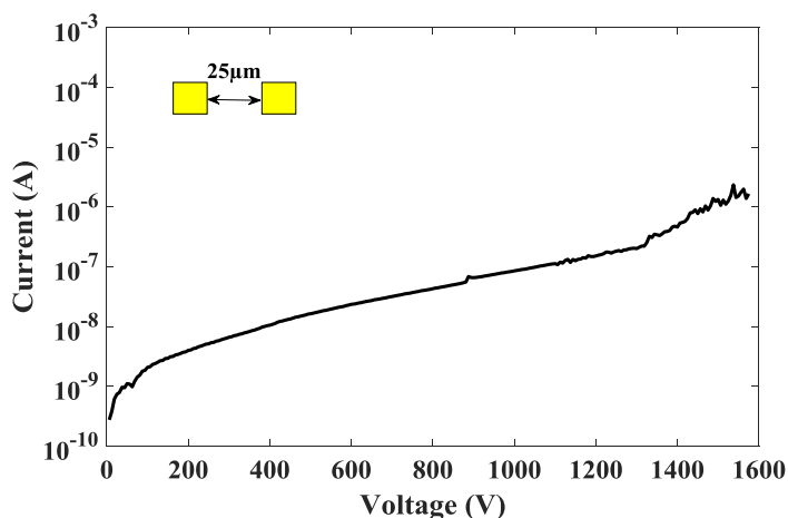
Figure 153 Claquage latéral entre deux contacts isolés distants de 25 \mu\text{m}
