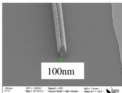
Figure 154 Image SEM d'une grille de 100nm fabriquée sur l'échantillon HEMT ultrafin
