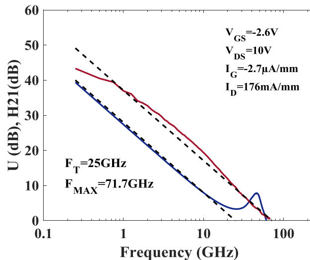
Figure 70 Caractéristiques petit signal typiques d'un composant 2x75μm de la filière GH25
