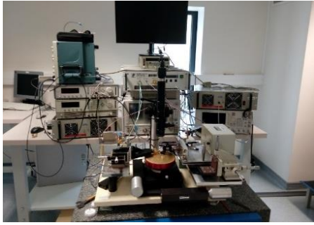
Figure 25 Photo du banc load pull actif et son synoptique optimisé par notre groupe [30]
