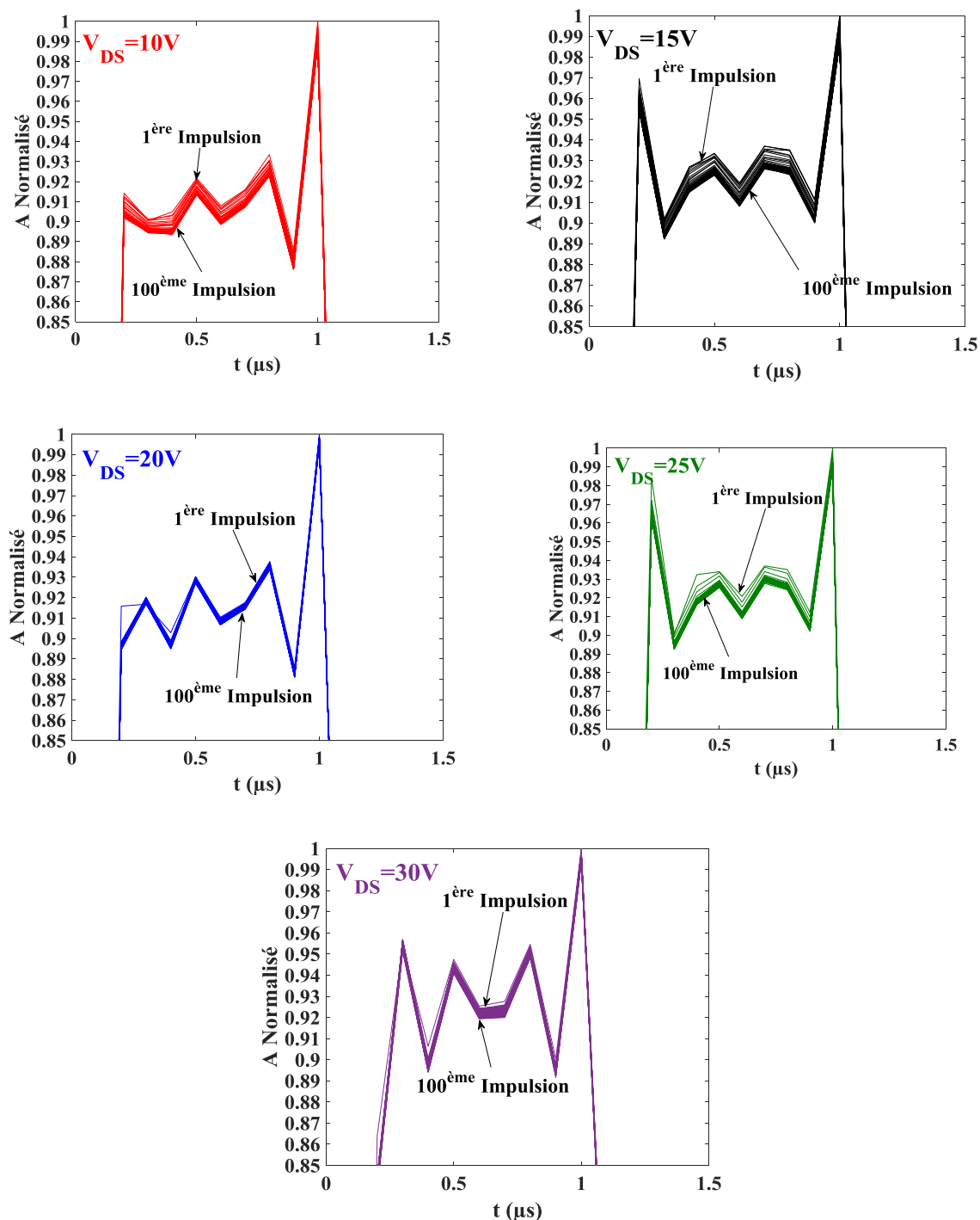
Figure 96 Diagramme de l'œil en amplitude pour différentes tensions de polarisation d'un transistor 8 \times 50 \mu\text{m} de la technologie GH15
