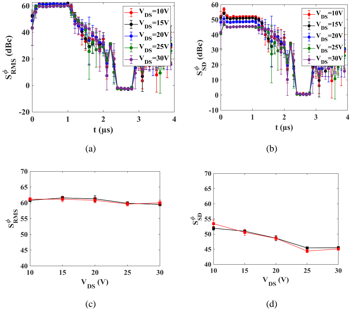
Figure 101 Stabilité de phase obtenue sur un transistor 8 \times 50 \mu m par la méthode RMS (gauche) et la méthode SD (droite)
