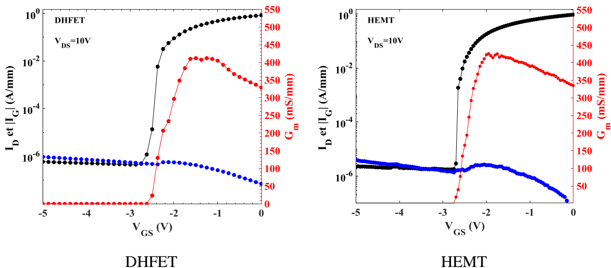
Figure 119 Caractéristiques de transfert obtenues sur les structures DHFET et HEMT
