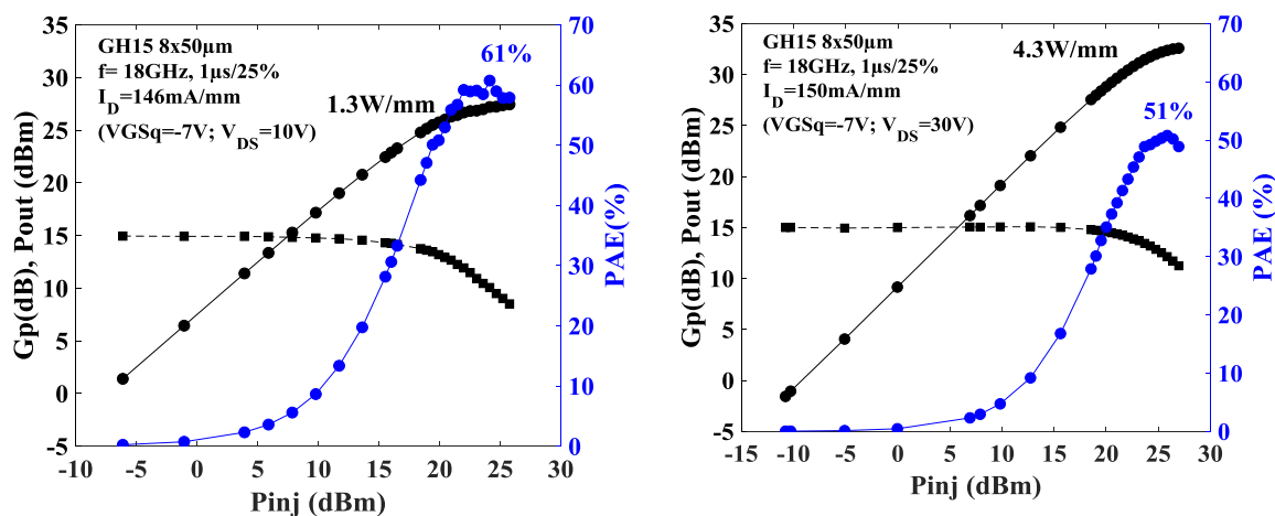
Figure 94 Performances RF 18 \text{GHz} à V_{\text{DS}} = 10 \text{V} et V_{\text{DS}} = 30 \text{V} dans le cadre des applications senseurs aéroportés d'un transistor 8 \times 50 \mu\text{m} de la technologie GH15.
