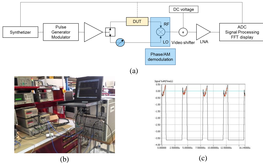
Figure 34 (a) Synoptique du banc P2P (b) Photo du banc, (c) image de l'interface avec la sélection des points (c)
