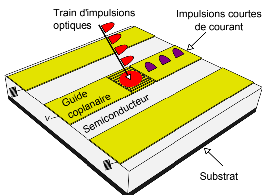
FIGURE 1.8 – Principe de génération d'impulsions de photocourant sous éclairage impulsif dans un photodétecteur sur ligne coplanaire interrompue par une zone interdigitée (a) Le même principe est illustré dans le cas d'une onde rayonnée par un photodétecteur intégré à une antenne dipôle
