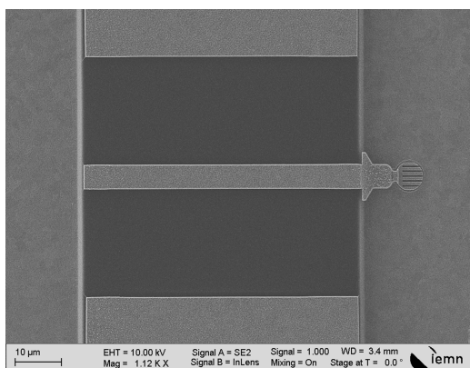
e) MSM-InAlAs/InGaAs
