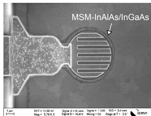
f) MSM-InAlAs/InGaAs
