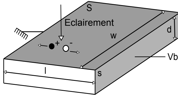
FIGURE 2.3 – Géométrie simplifiée d'un photoconducteur planaire
