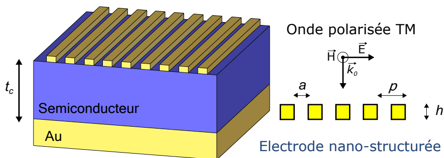
FIGURE 3.10 – Représentation schématique d'une cavité résonante à réseau de diffraction
