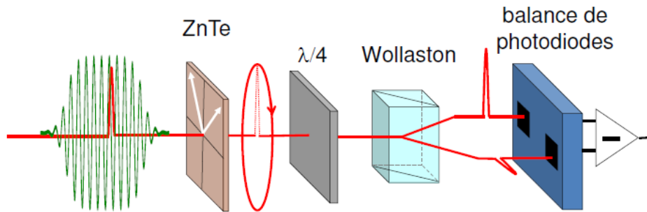
FIGURE 1.11 – Système de détection électro-optique d'ondes THz utilisant un cristal de ZnTe. La figure est issue de la référence [Maysonnave, 2014]
