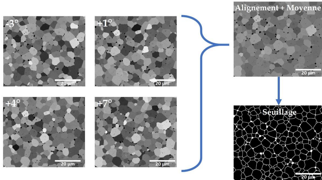
Figure 63 : Etapes du traitement d'image à l'aide du logiciel ImageJ illustrées avec une zone de la pastille, composée de nano-poudres, frittée à 1600°C pendant 1h. Les traits blancs représentent les joints de grains et les points blancs représentent les pores. 178 grains sont analysés sur cette zone.
