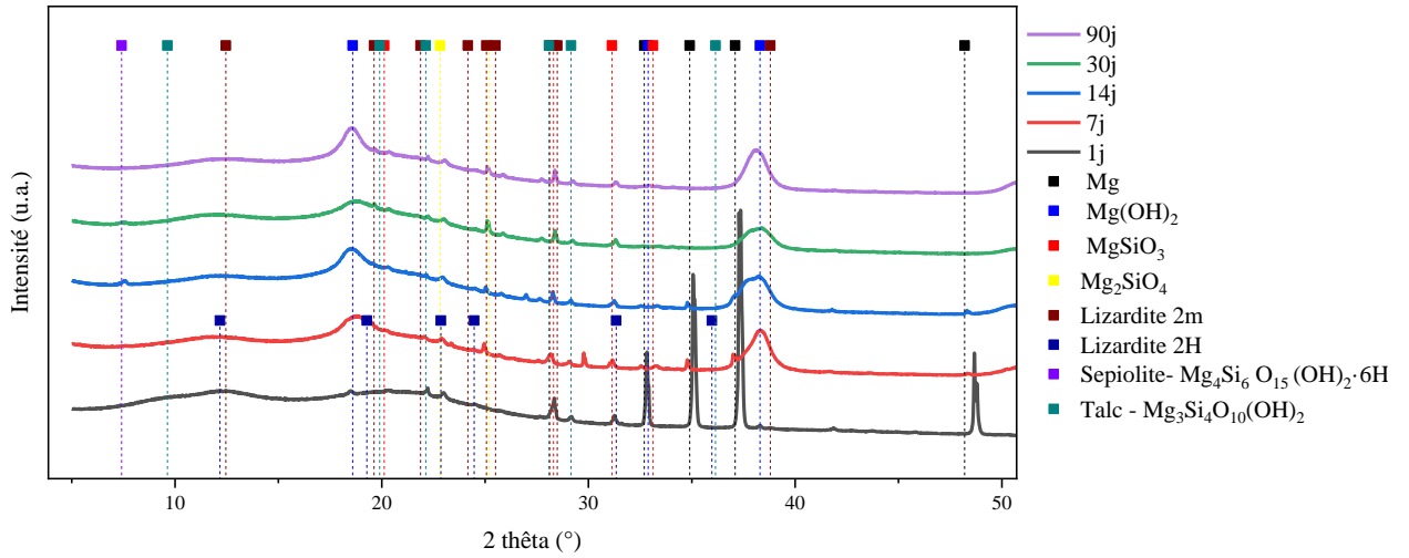
Figure 156 : Evolution des PC de corrosion par DRX-IR de l'échantillon SP-14 au cours du temps avec un angle incident de 0.2°.
