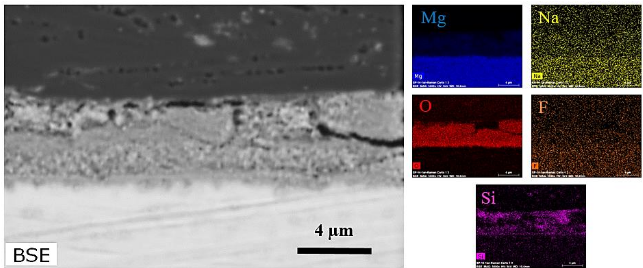
Figure 170 : Micrographies enregistrées d'une zone de la section polie de l'échantillon SP-14 corrodé pendant 1 an et cartographies élémentaires EDX correspondantes des éléments Mg, O, Si, F et Na
