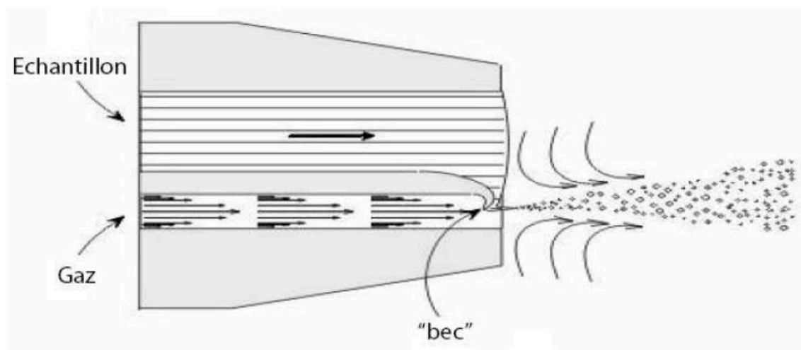
Figure 26. Schéma de fonctionnement de la pointe d'un nébuliseur parallèle (Burgener).
