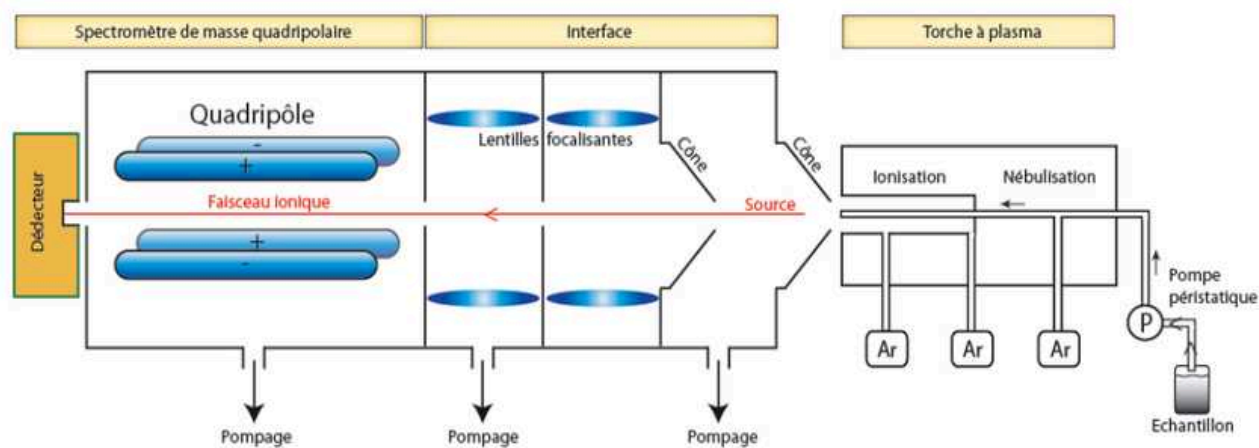
Figure 18. Schéma de fonctionnement hors couplage d'un ICP-MS [17].
