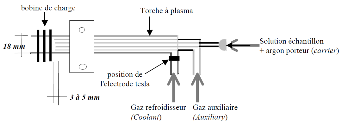
Figure 19. Schéma de positionnement des composants de la source d'ionisation de l'ICP-MS [3].
