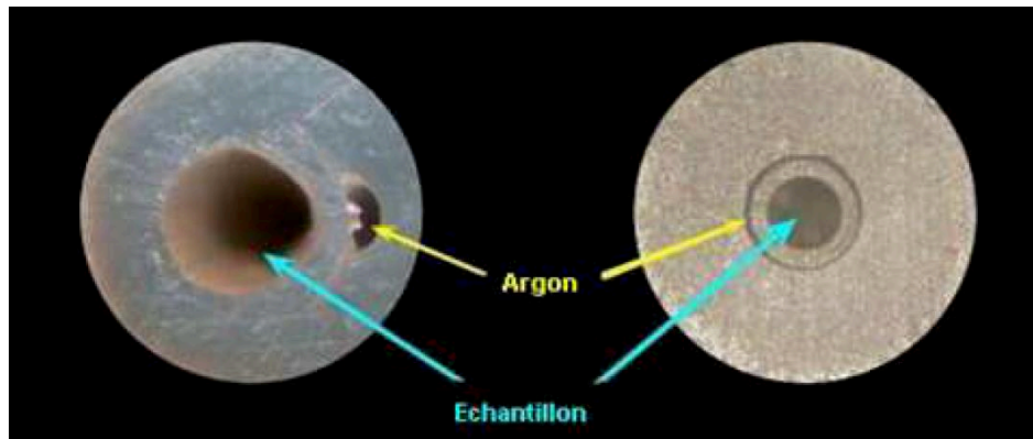
Figure 25. Nébuliseur parallèle (gauche) et nébuliseur concentrique (droite) à la même échelle (Burgener).
