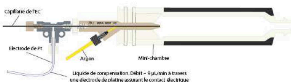
Figure 22. Représentation de l'interface commerciale Mira Mist CE ® (Burgener Research, Mississauga, Ontario, Canada).
