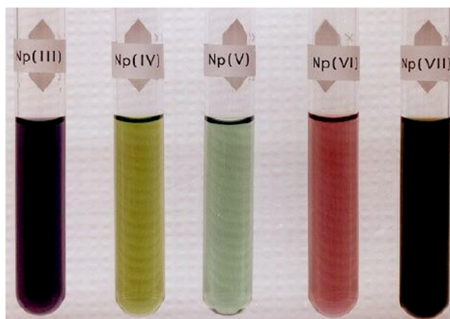
Figure 4. Observation de solutions concentrées de neptunium présent à différents degrés d'oxydation [17].
