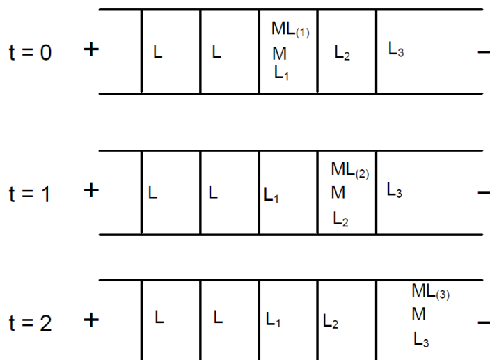
Figure 32. Schéma représentant le comportement d'un complexe ML labile en présence de ligand au sein de l'électrolyte. t=0 : le complexe, le métal et le ligand L 1 (ligand complexé) sont localisés dans la même tranche d'électrolyte. t=1 : Le complexe et le métal migrent plus rapidement que L 1 , le ligand du complexe est alors remplacé par le ligand L 2 contenu dans la tranche d'électrolyte suivante. t=2 : même chose entre L 2 et L 3 .
