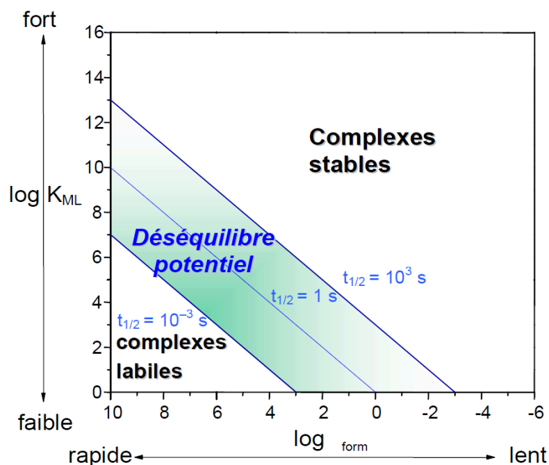
Figure 30. Comportement des complexes lors de la séparation électrophorétique en fonction de leur temps de demi-vie [33].
