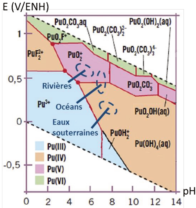
Figure 8. Diagramme de Pourbaix à 25 °C du plutonium ( C_{Pu} = 10^{-8} M) en milieu aqueux en présence d'anions CO_3^{2-} , F^- et OH^- [41].
