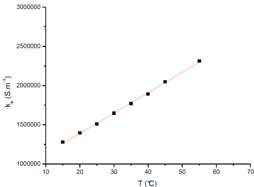
Figure 14. Variation de la conductivité électrique d'un électrolyte de perchlorate de sodium présent à la concentration de 0,20 M en fonction de la température.
