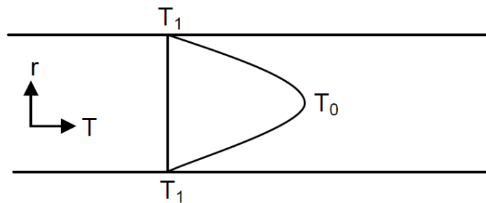
Figure 12. Représentation du profil de température au sein de l'électrolyte parcourant le capillaire [3].
