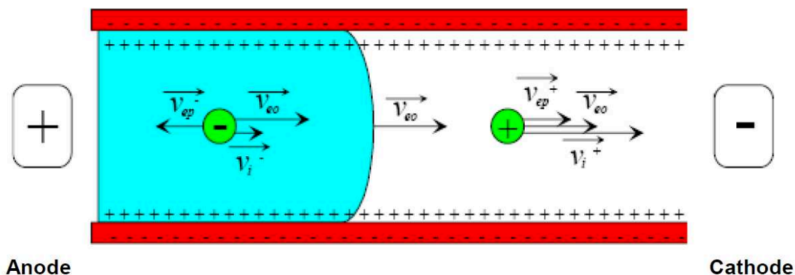
Figure 10. Représentation du mouvement des ions en solution au sein d'un capillaire sous l'effet d'un champ électrique [3].
