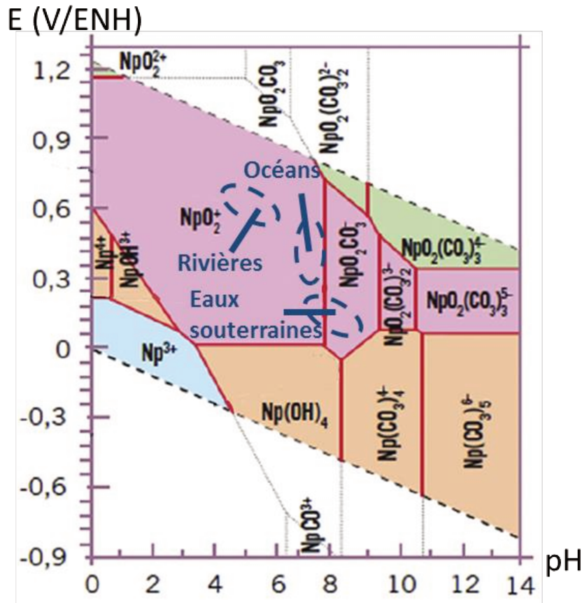
Figure 7. Diagramme de Pourbaix à 25 °C du neptunium ( C_{\text{Np}} = 10^{-8} \text{ M} ) en milieu aqueux en présence d'anions \text{CO}_3^{2-} , \text{F}^- et \text{OH}^- [36].
