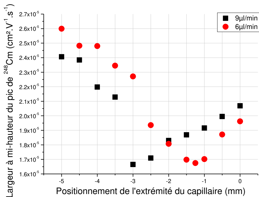
Figure 27. Largeur à mi-hauteur du pic d'électrophorégramme de ^{248}\text{Cm} en fonction du débit de liquide de compensation et de la position de l'extrémité du capillaire par rapport au nez du nébuliseur [21].
