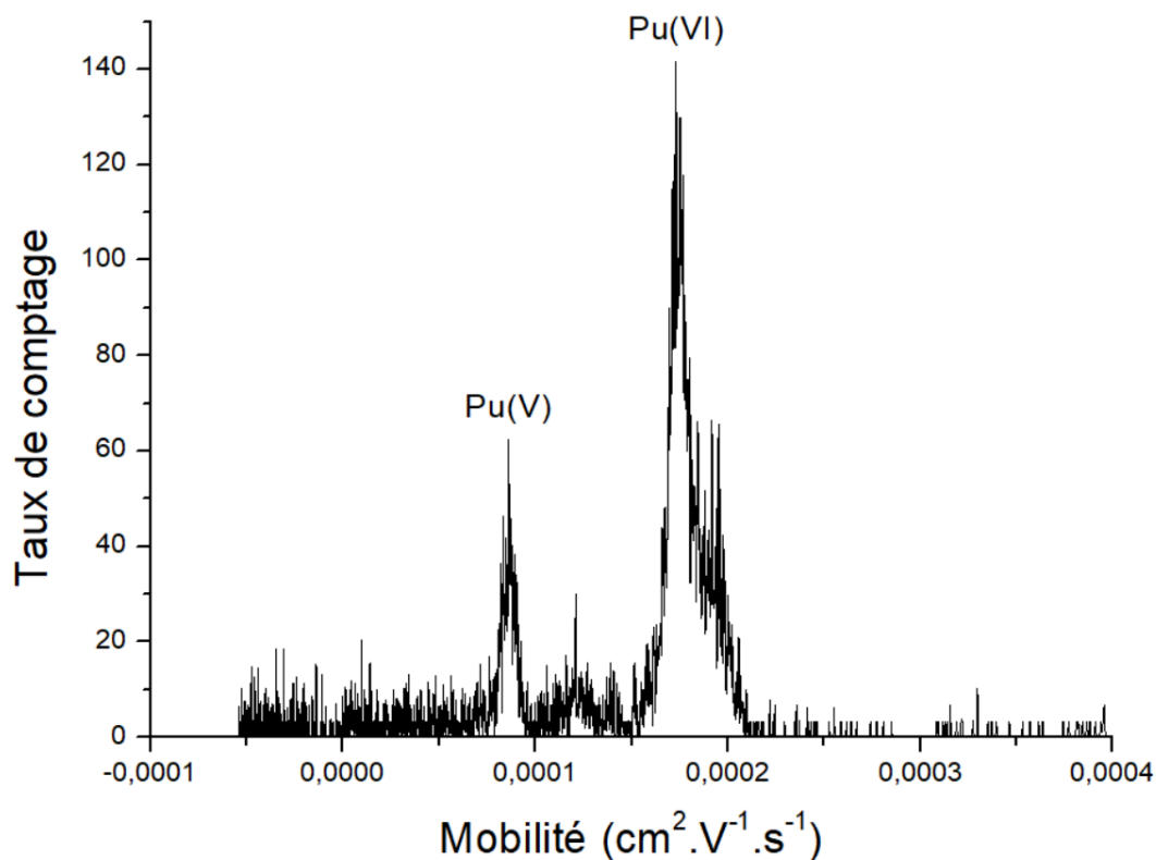
Figure 34. Electrophorogramme de Pu(VI) et Pu(V) à partir d'une solution de 239 Pu à 10 -8 M en milieu NaClO 4 0,202 m à pH = 3 et T = 25 °C.
