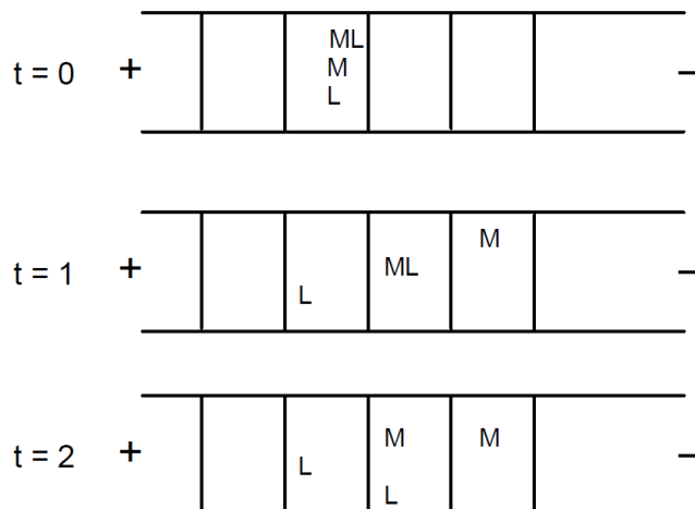
Figure 31. Schéma représentant le comportement d'un complexe ML labile en l'absence de ligand au sein de l'électrolyte. t=0 : le complexe, le ligand et le métal sont localisés dans la même tranche d'électrolyte. t=1 : le métal migre plus rapidement que le complexe qui migre lui-même plus rapidement que le ligand. t=2 : l'absence de ligand dans l'électrolyte entraîne la dissociation totale du complexe. L'unité de temps associée à ces étapes correspond à un pas de temps nécessaire au changement de bande de migration du complexe.
