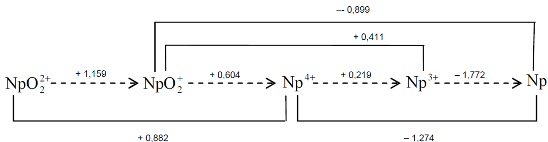
Figure 3. Potentiels standards des différents couples mettant en jeu le neptunium (exprimés en V/ENH) à 25 °C et à force ionique nulle [16].
