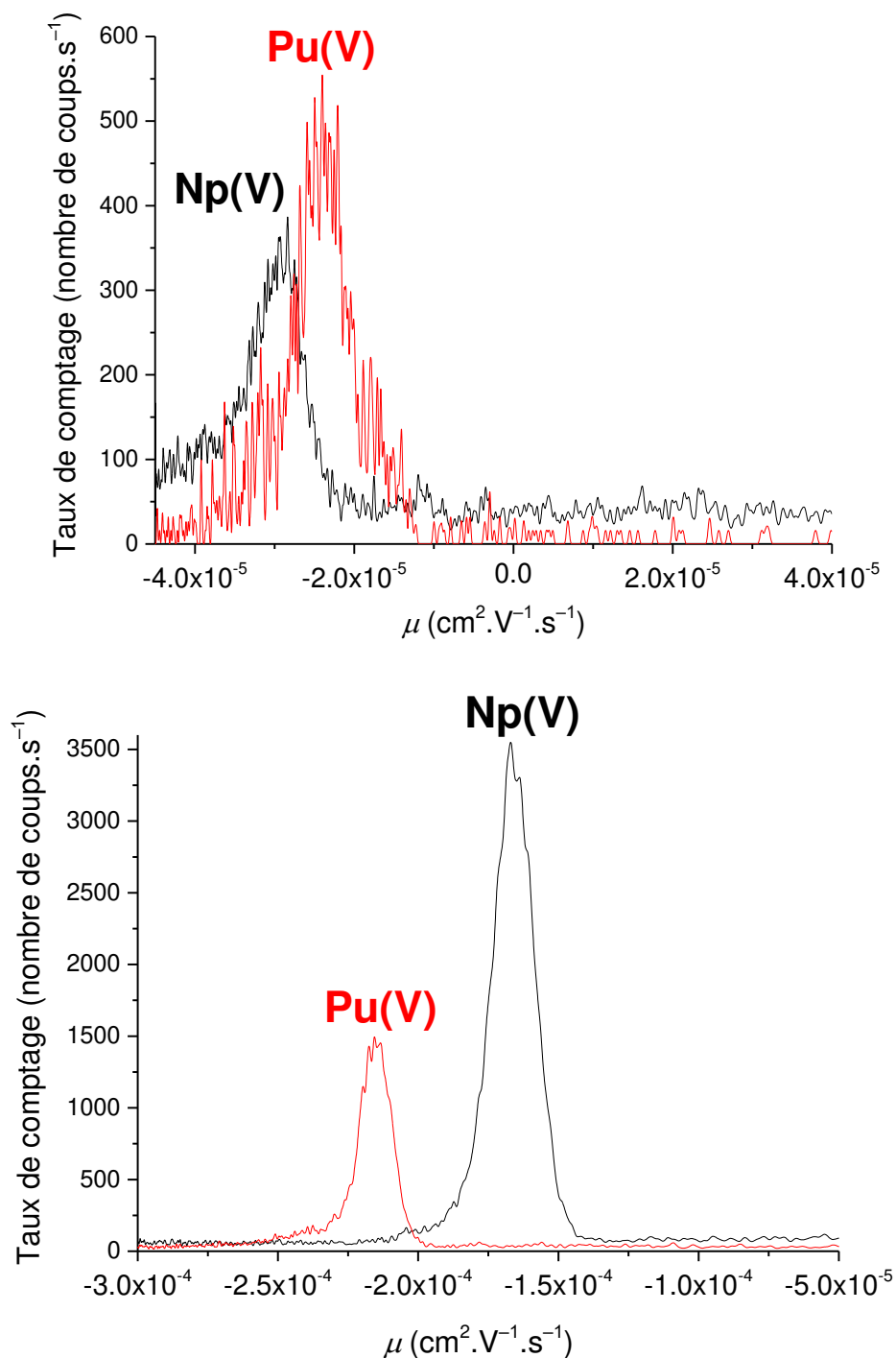
Figure 39. Electrophorégrammes obtenus dans NaClO 4 0,202 m avec [\text{CO}_3^{2-}] = 10^{-2}\text{M} et [\text{NpO}_2^+] = [\text{PuO}_2^+] = 10^{-8}\text{M} pour les espèces carbonatées de Np(V) (en noir) et de Pu(V) (en rouge) à 25°C (en haut) et à 50°C (en bas). L'axe des mobilités est obtenu par correction du temps de séparation avec le flux électroosmotique.
