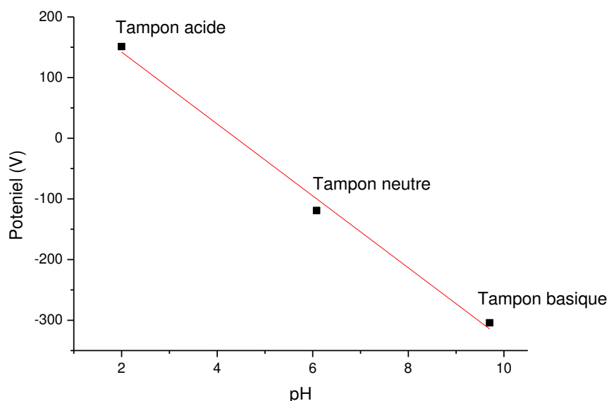
Figure 28. Représentation graphique de la relation de Nernst reliant le potentiel et le pH de solutions tampon carbonate à 25 °C et à une force ionique de 0,20 M.
