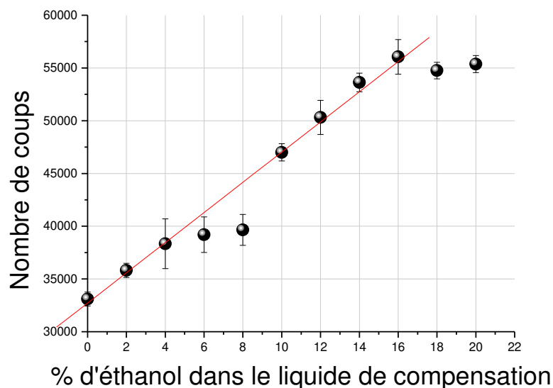
Figure 24. Sensibilité en fonction de la proportion d'éthanol au sein du liquide de compensation dans le cas de ^{238}\text{U} [21].
