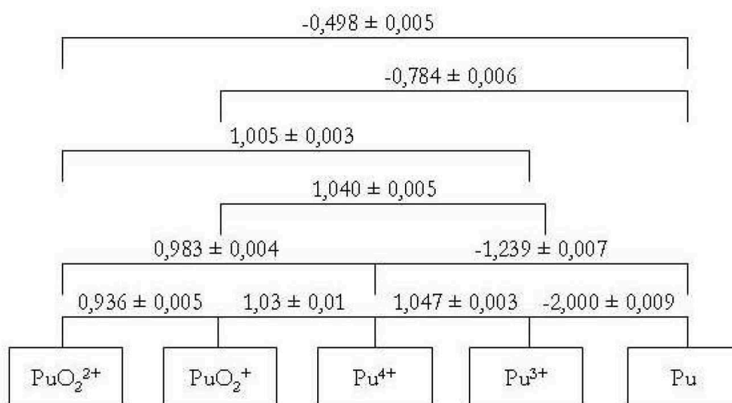
Figure 5. Potentiels standards des différents couples mettant en jeu le plutonium (exprimés en V/ENH) à 25 °C et à force ionique nulle [16].
