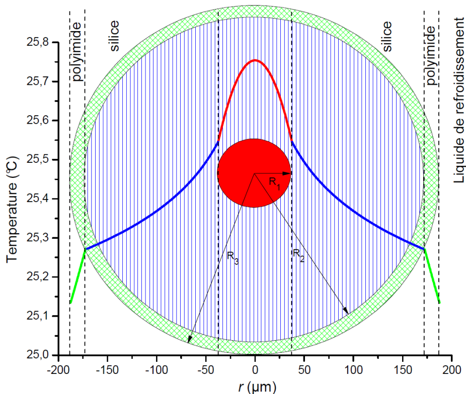
Figure 13. Schéma de coupe d'un capillaire et le profil de température interne pour une solution de perchlorate de sodium à 0,20 M lors d'une séparation électrophorétique de 7 kV à 25 °C [3].
