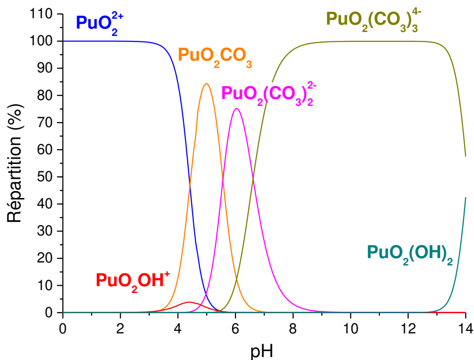
Figure 37. Diagramme de répartition des espèces présentes dans une solution de Pu(VI) à 10^{-8} M en milieu carbonate 0,1 M et \text{NaClO}_4 à 25 \pm 1 °C et à I = 0,202 m (réalisé à partir des constantes obtenues dans cette étude et des constantes d'hydrolyse de la littérature [4]).
