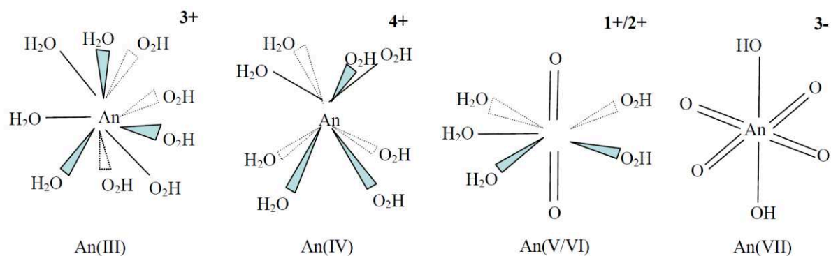
Figure 2. Première sphère d'hydratation des actinides selon leur degré d'oxydation.
