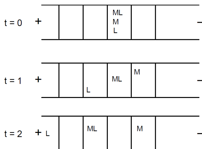
Figure 33. Schéma représentant le comportement d'un complexe ML stable. t=0 : le complexe, le métal et le ligand sont localisés dans la même tranche d'électrolyte. t=1 : le métal migre plus rapidement que le complexe qui migre plus rapidement que le ligand. t=2 : pas de dismutation du complexe, les trois espèces migrent à des vitesses différentes.
