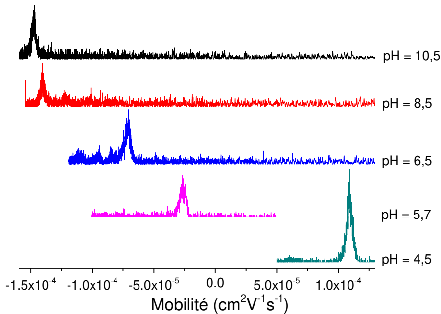
Figure 35. Electrophorégrammes de complexes de carbonates de Pu(VI) à différents pH en milieu NaClO 4 0,202 m et à 25 ± 1 °C. La concentration en ions carbonate varie de 10 -1 M (pH = 10,5) à 10 -8 M (pH = 4,5) et la concentration en Pu est de 10 -9 M.
