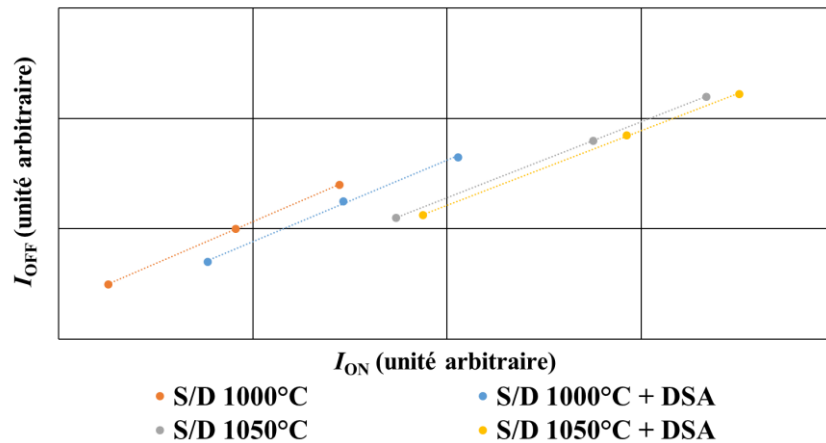
Figure 51 I_{OFF} = f(I_{ON}) pour des MOS d'aire 0,06 \times 1,00 \mu\text{m}^2 en fonction de l'utilisation d'un DSA et de la température du recuit d'activation (valeurs médianes)
