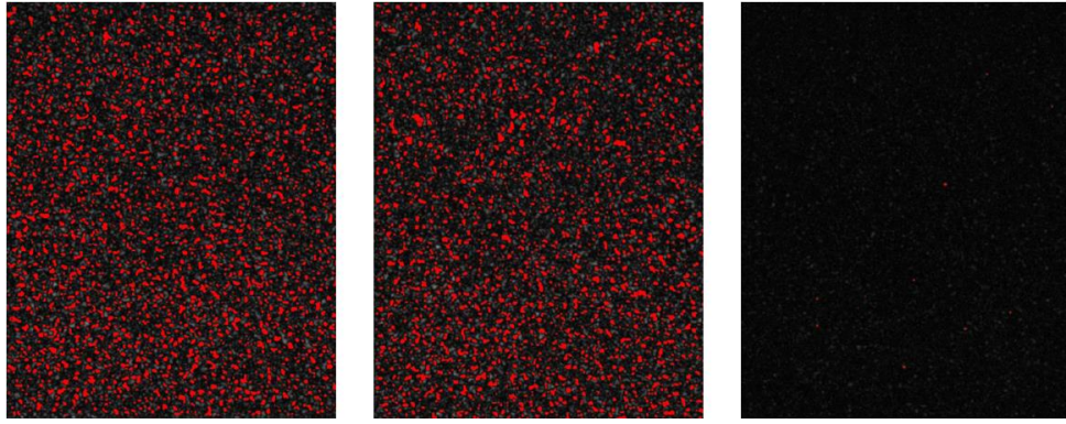
Figure 116 Reconstruction issues de la technique de photoluminescence montrant les défauts étendus en fonction de l'espèce implantée (arsenic à gauche, phosphore au centre et carbone plus phosphore à droite)
