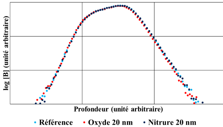
Figure 65 Profils de bore en fonction du procédé de fabrication utilisé issus de SIMS
