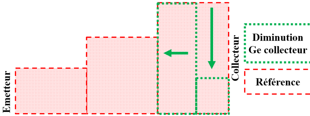
Figure 77 Représentation schématique de la diminution du taux de germanium côté collecteur
