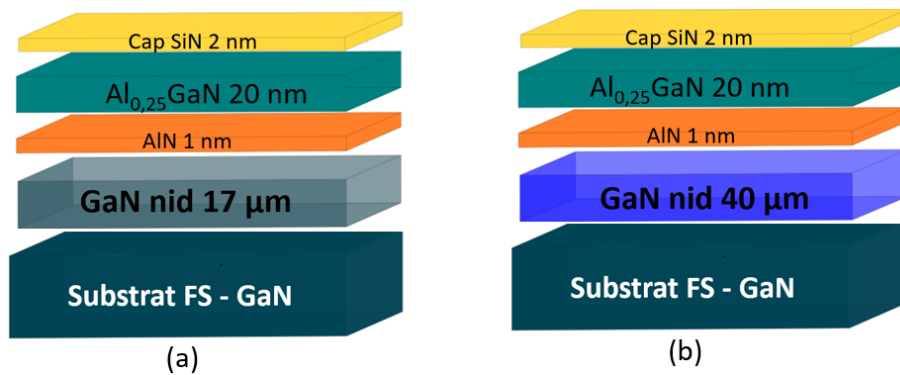
Figure 3. 7 : Structures HEMTs AlGaN/GaN sur substrat FS-GaN: (a) avec 17 \mu\text{m} de GaN-nid, (b) avec 40 \mu\text{m} de GaN-nid
