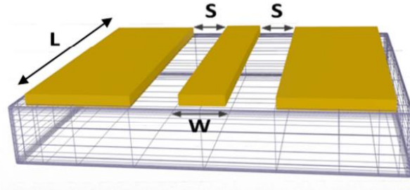
Figure 3. 6 : Topologie d'une ligne de transmission CPW
