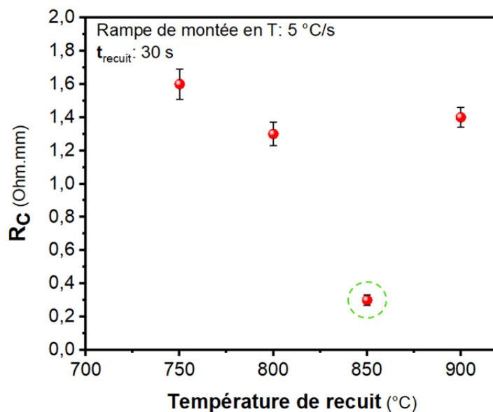
Figure 2.30 : Résistance de contact en fonction de la température de recuit pour une rampe de montée en température de 5 °C/s
