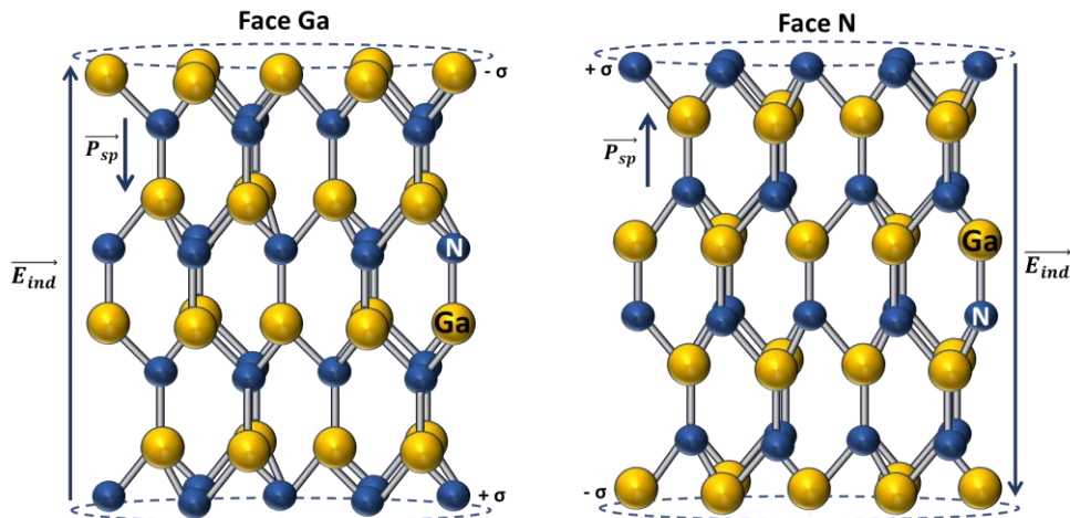
Figure 1.4 : Représentation du champ électrique généré à travers deux couches fines de GaN hexagonales de polarité différente
