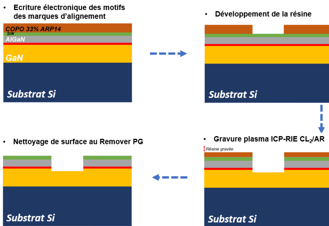
Figure 2. 19 : Schéma descriptif de la réalisation des marques d'alignement
