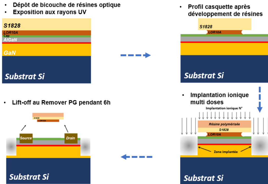
Figure 2. 11 : Schéma descriptif de l'étape de l'isolation des composants par implantation ionique
