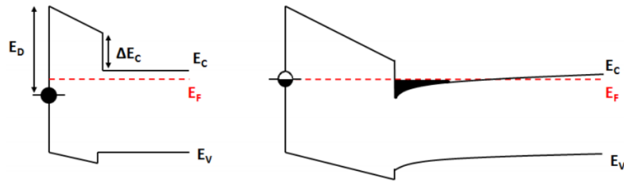
Figure 1. 6 : Diagramme de bandes de deux structures AlGaN/GaN avec une épaisseur d'AlGaN inférieure (à gauche) et supérieure (à droite) à l'épaisseur de barrière critique nécessaire à la formation du gaz d'électrons
