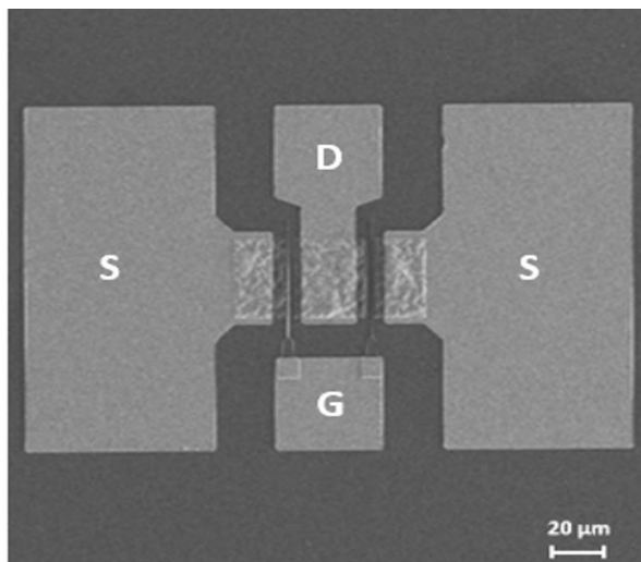
Figure 2. 37 : Image MEB d'une vue de haut d'un HEMT AlGaIn/GaN sur substrat FS-GaN en fin de procédé de fabrication
