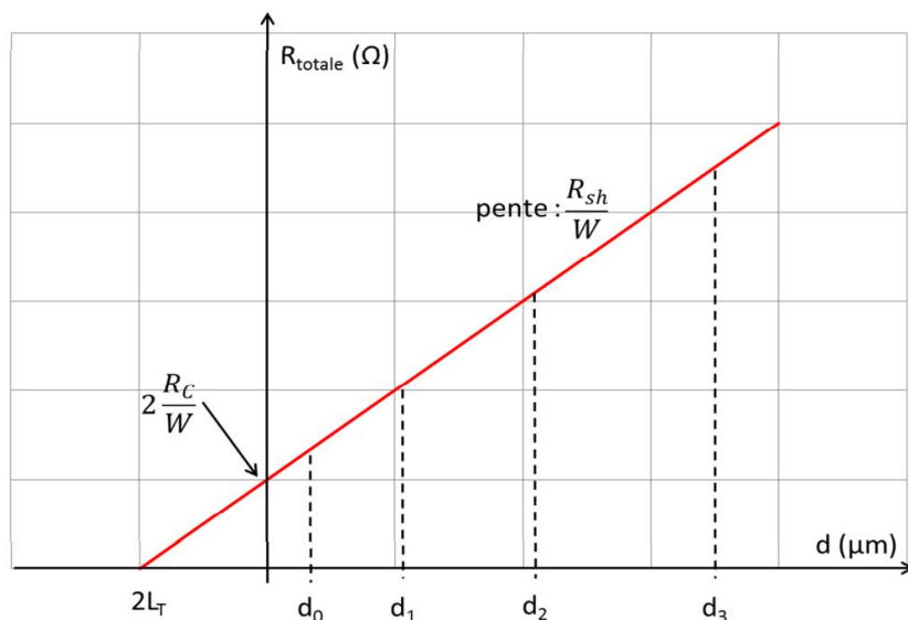
Figure 2. 26 : Résistance totale mesurée en fonction de la distance entre les contacts ohmiques
