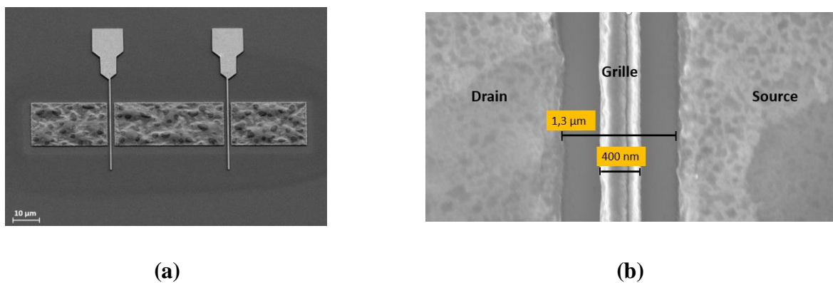
Figure 2. 35 : (a) Vue d'ensemble du transistor après lift-off de la grille, (b) agrandissement d'une vue de haut sur l'espace source-drain
