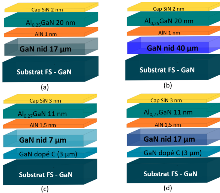
Figure 1. 20 : Structures HEMT fournies par le CRHEA : (a) avec 17 µm de GaN nid, (b) avec 40 µm de GaN nid, (c) avec 3 µm de GaN dopé C et 7 µm de GaN nid, (d) avec 3 µm de GaN dopé C et 17 µm de GaN nid
