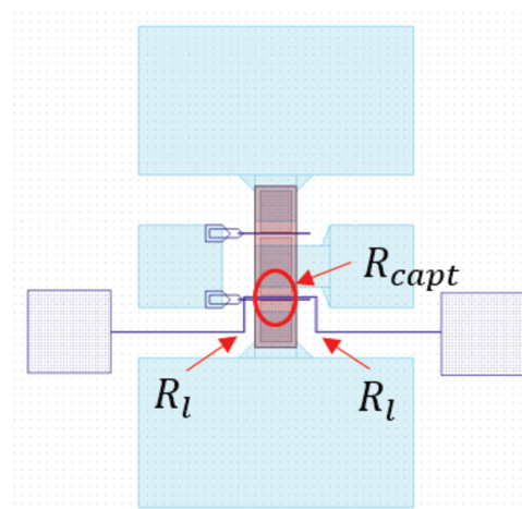
Figure 39 Layout d'un capteur de base intégré dans un transistor présentant des lignes d'accès coplanaires
