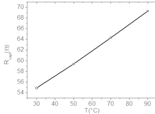
Figure 83 Courbe de calibration du capteur
