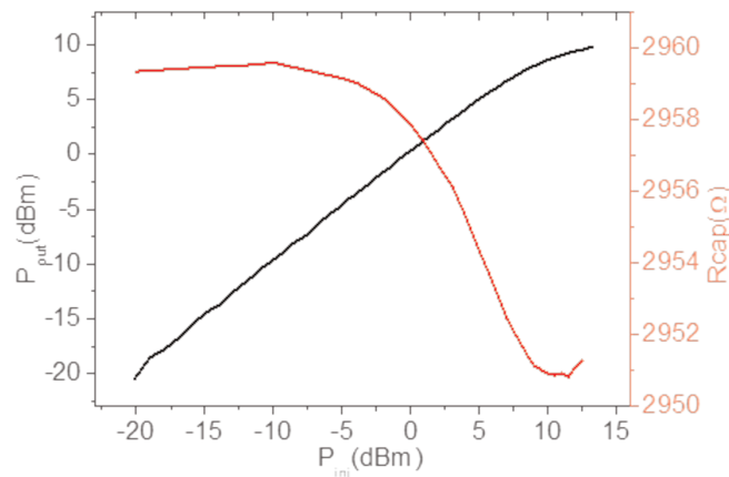
Figure 91 Evolution de la résistance du capteur à deux accès et de la puissance de sortie en fonction de la puissance injectée
