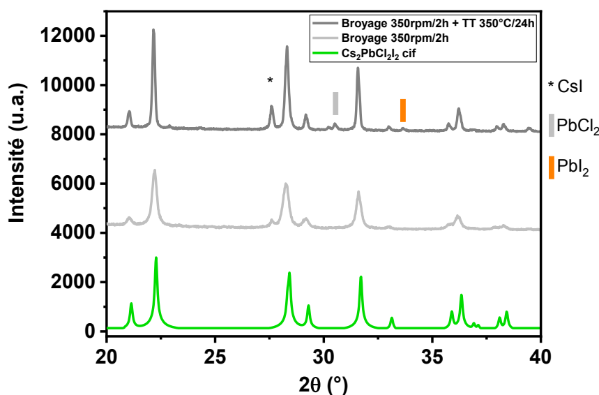
Figure 4 Diffractogrammes aux RX d'un échantillon préparé par un mélange de CsI et PbCl 2 broyé au broyeur planétaire puis traité à 350°C/24h sous air.
