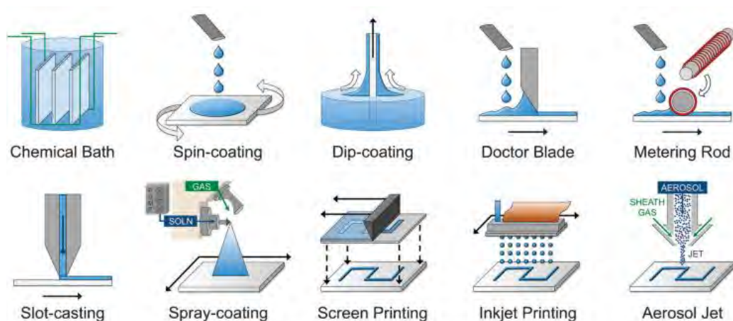
Figure 6 Procédés de fabrication de films minces [15].
