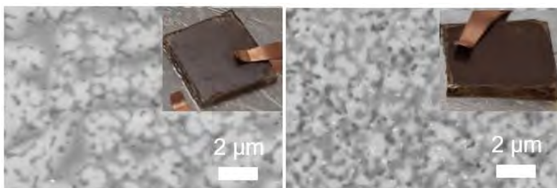
Flux à 1 bar et 0,5 cm 50°C/2 min → 140°C/5 min → 300°C/10 min
