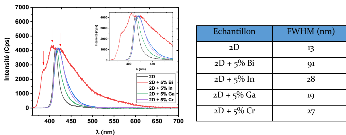
Figure 28 Spectres UV-Visible de photoluminescence des monocristaux de \text{Cs}_2\text{Pb}_{1-x}\text{M}_x\text{Cl}_2\text{I}_2 pour x=0 et x=5\% avec M = \text{Bi}, \text{Ga}, \text{In} et \text{Cr} et largeurs à mi-hauteur du pic d'émission de photoluminescence des monocristaux correspondants.
