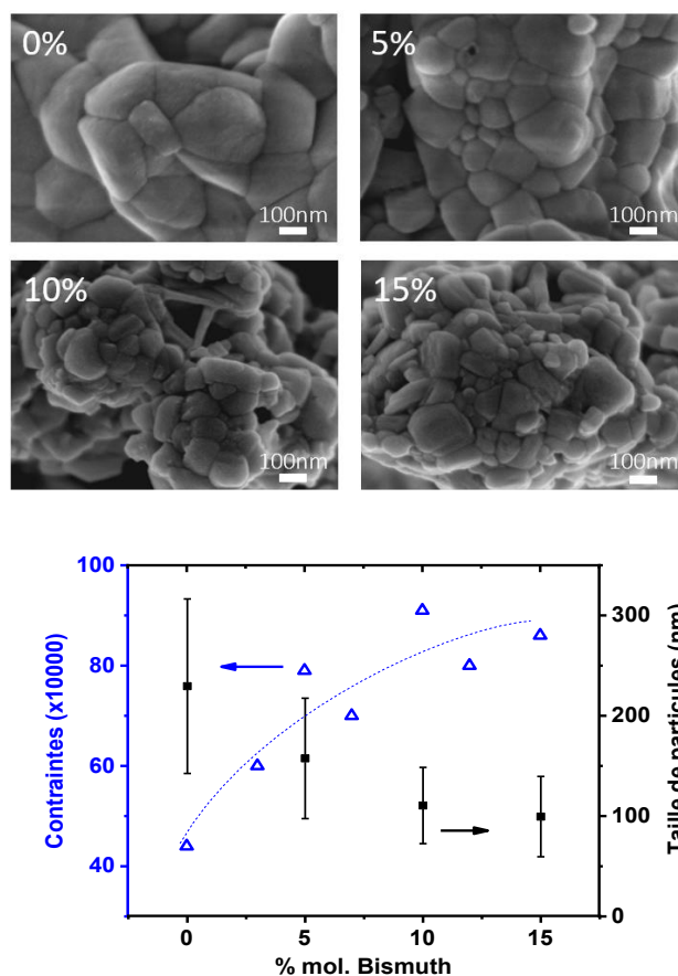
Figure 6 Images MEB de Cs 2 Pb 1-x Bi x Cl 2 I 2 pour différents taux de bismuth (à gauche). Micro-contraintes et tailles de particules en fonction du taux de bismuth (à droite).
