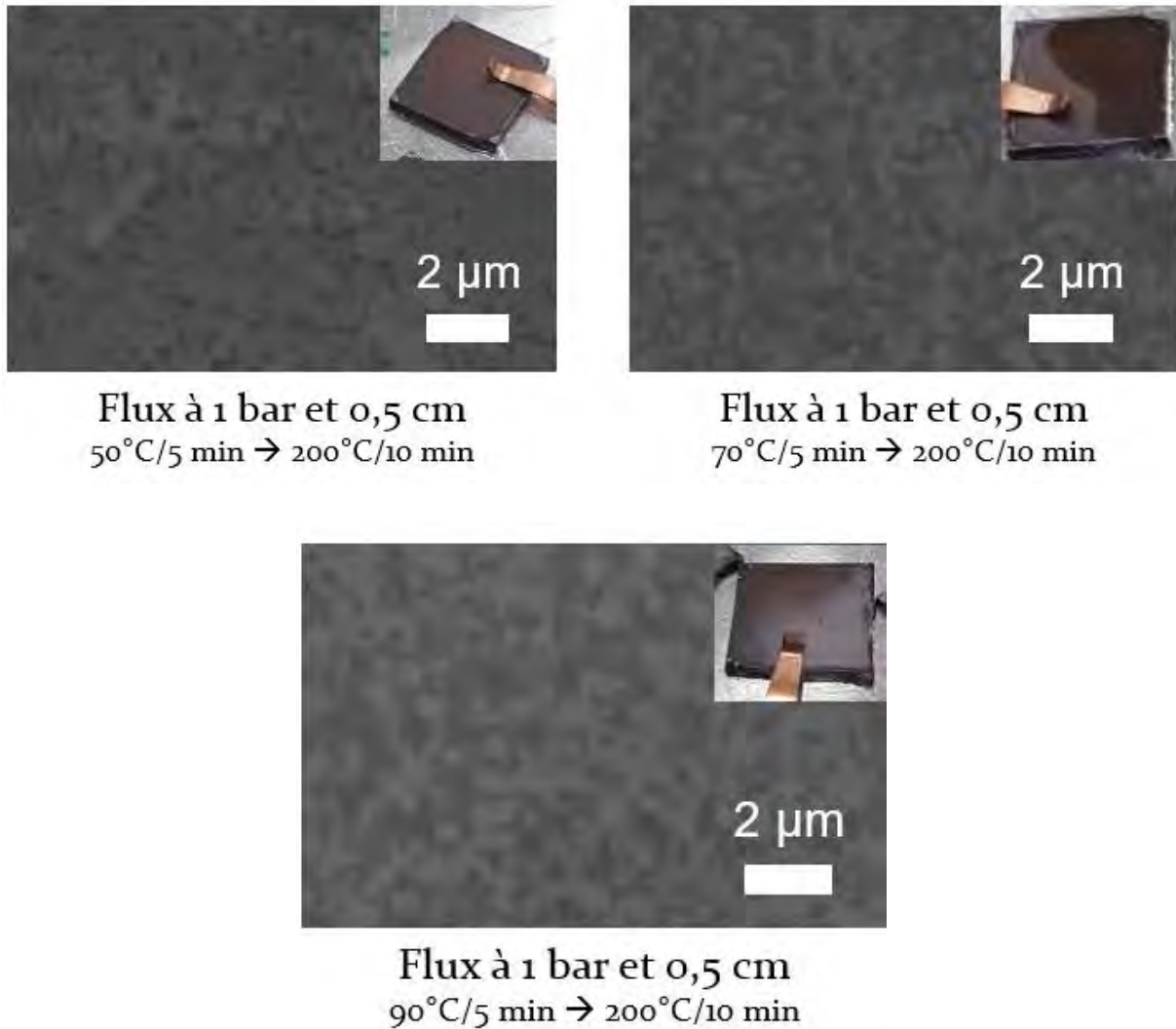
Figure 12 Images MEB et photographies correspondantes de dépôts de \text{CsPbI}_2\text{Br} sur \text{FTO}/\text{SnO}_2 en fonction de la première température de traitement thermique ( T_1 ).
