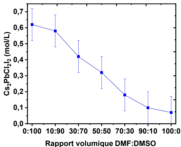
Figure 13 Concentration maximale de \text{Cs}_2\text{PbCl}_2\text{I}_2 en fonction du rapport DMF:DMSO.
