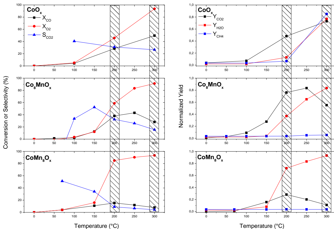
Figure 4. Données spectromètre de masse à quadrupôle(QMS) (a), (b), (c) des \text{CoO}_x\text{-MnO}_x . Conditions: 1 mbar de 1% \text{CO} , 1% \text{O}_2 et 98% \text{H}_2 , plage de température entre 50 et 300 °C avec une vitesse de chauffe de 10 °C / min entre chaque étage de température. Avant les tests d'activité, les échantillons ont été prétraités dans la chambre XPS sous 1 mbar de \text{H}_2 à 400 °C pendant 1 h.
