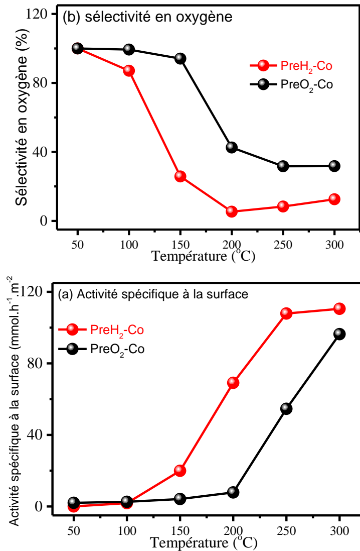
Figure 1. a) Activité spécifique de surface ou quantité de CO convertie par surface en mmol h -1 m -2 et b) Sélectivité O 2 en CO 2 pour PreO 2 -Co et PreH 2 -Co en fonction des mesures de chromatographie en phase gazeuse (GC) en fonction de la température.
