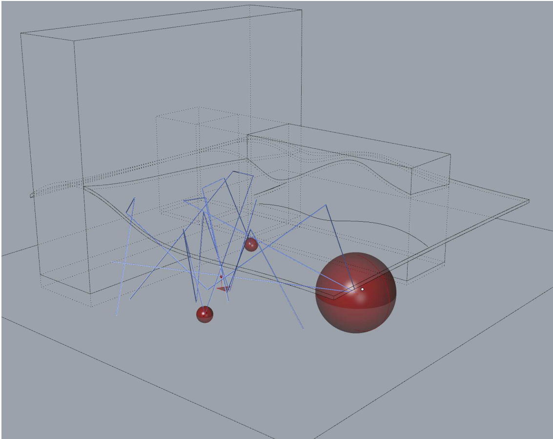
FIGURE 5.18 – Exemple d'une visualisation des premières, deuxièmes et troisièmes réflexions avec EsquisSons
