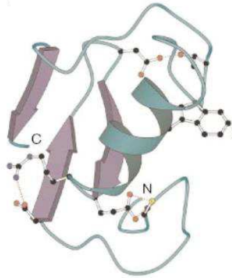
U-box protéine
