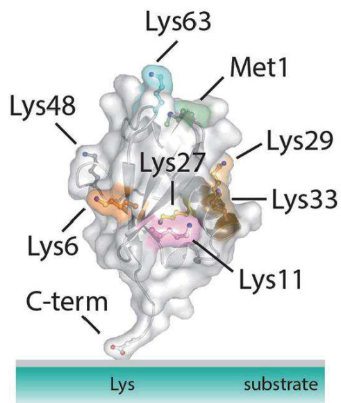
Figure 1.1.1 : L'ubiquitine
