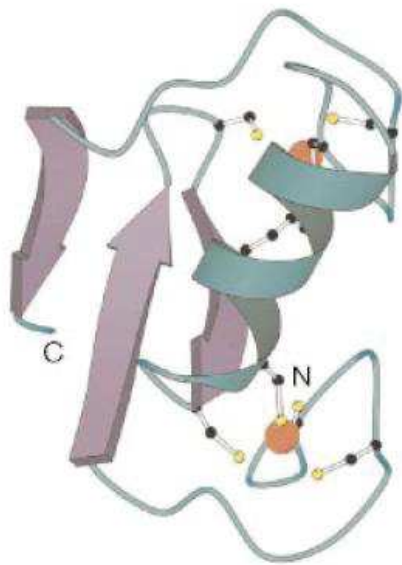
RING protéine
