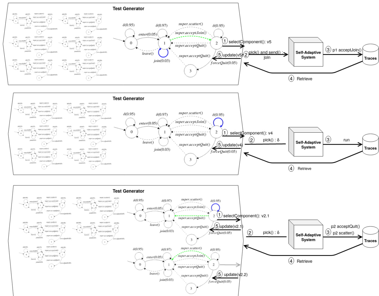
FIGURE 5.13 – Processus de génération d'évènements de test en ligne
