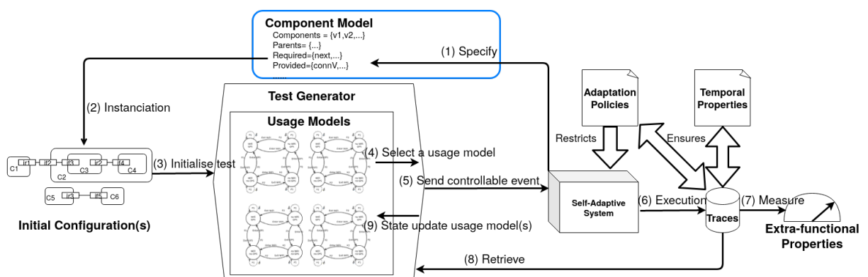
FIGURE 1.1 – Processus de génération de tests en ligne
