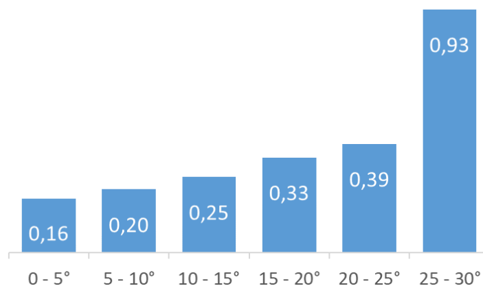
Figure 52 - Pourcentage de fausses détections en fonction de la topographie pour des plages de pentes données
