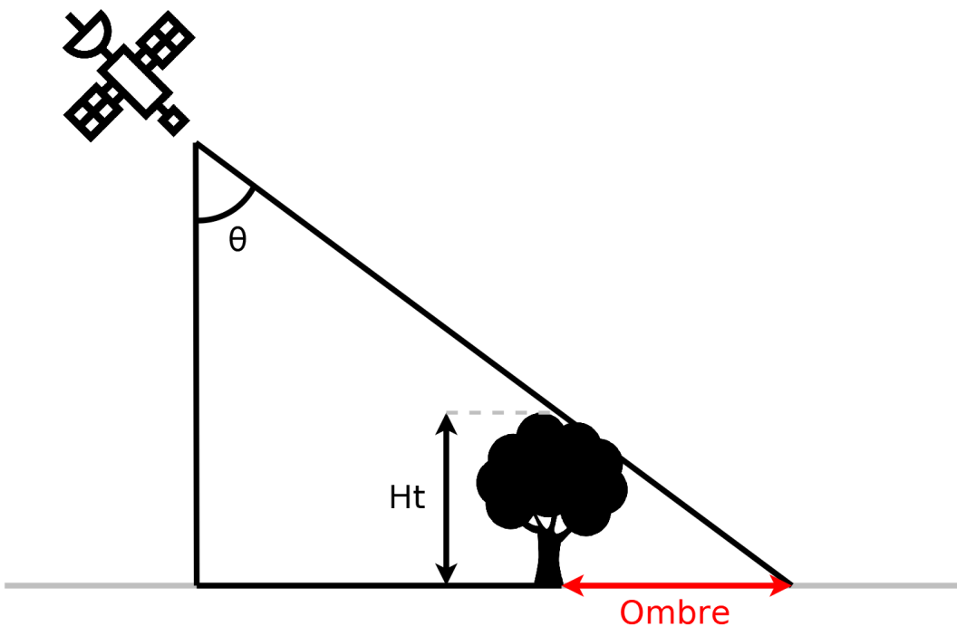
Figure 44 – Schéma de la relation entre l'angle d'incidence \theta , la hauteur d'un arbre Ht et la taille d'une ombre projetée sur sol plat.
