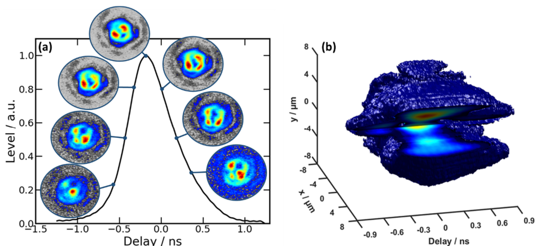
Figure 22 : Cartographie ST du faisceau au début du processus de nettoyage Kerr à 1,4 kW (Longueur de fibre : 5 m)
