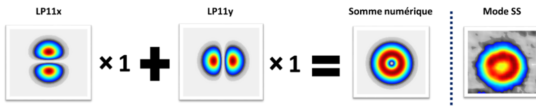
Figure 15 : Comparaison entre la somme en champ de mode LP11x et LP11y et la répartition modale issue de la mesure SS de la cascade Raman
