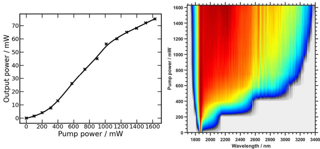
Figure 23 : (Gauche) Puissance mesurée à la sortie de la fibre InF 3 en fonction de la puissance de la pompe. (Droite) Évolution correspondante du profil spectral.
