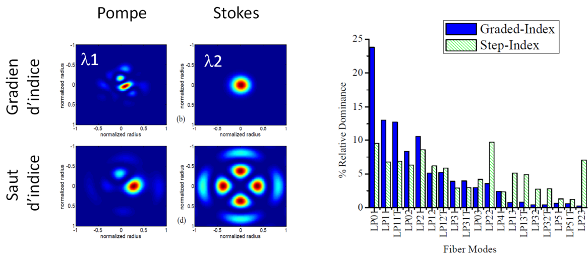
Figure 5 : Gauche, processus de nettoyage Raman dans une GIMF et dans une fibre à saut d'indice; Droite, Gain Raman en fonction des modes dans une GIMF. [Terry 2007]
