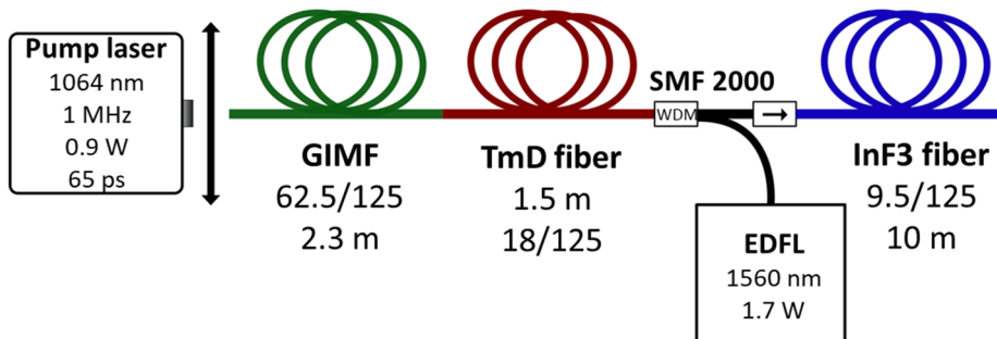
Figure 21 : Montage expérimental de l'amplification des GPI
