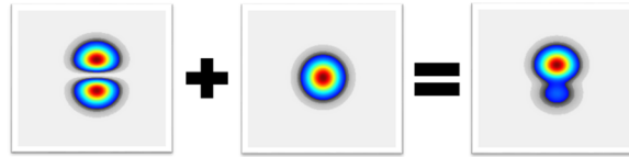
Figure 28 : Somme numérique d'un LP01 et d'un LP11 ; l'énergie sur le LP11 est le double de l'énergie sur le LP01
