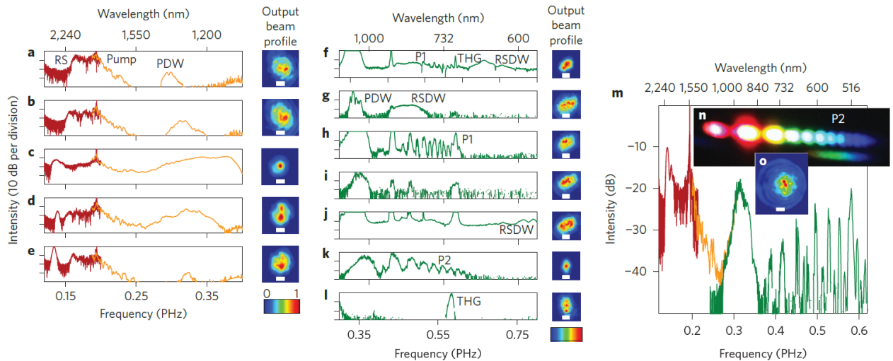
Figure 10 : Évolution spectrale pour plusieurs excitations modales. Les courbes sont les spectres infrarouges (a-e), les spectres visibles (f-i) et la somme des deux (m). Les images sont les champs proches du faisceau en sortie de GIMF correspondantes. [Wright 2015]
