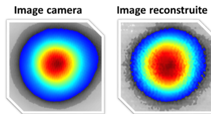
Figure 16 : Comparaison entre l'image en champ proche d'un faisceau gaussien pris à la caméra CCD et l'image résultant de l'intégration dans le temps des images issues de la mesure ST
