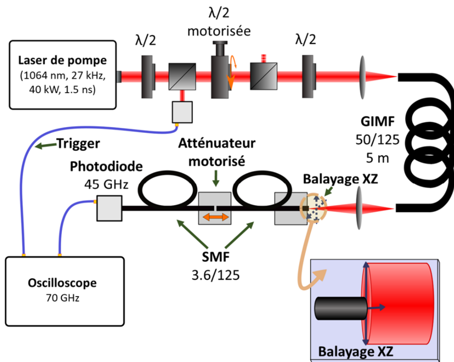
Figure 13 : Configuration expérimentale pour la cartographie spatiotemporelle du faisceau.
