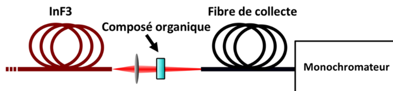
Figure 35 : Banc expérimental de spectroscopie IR
