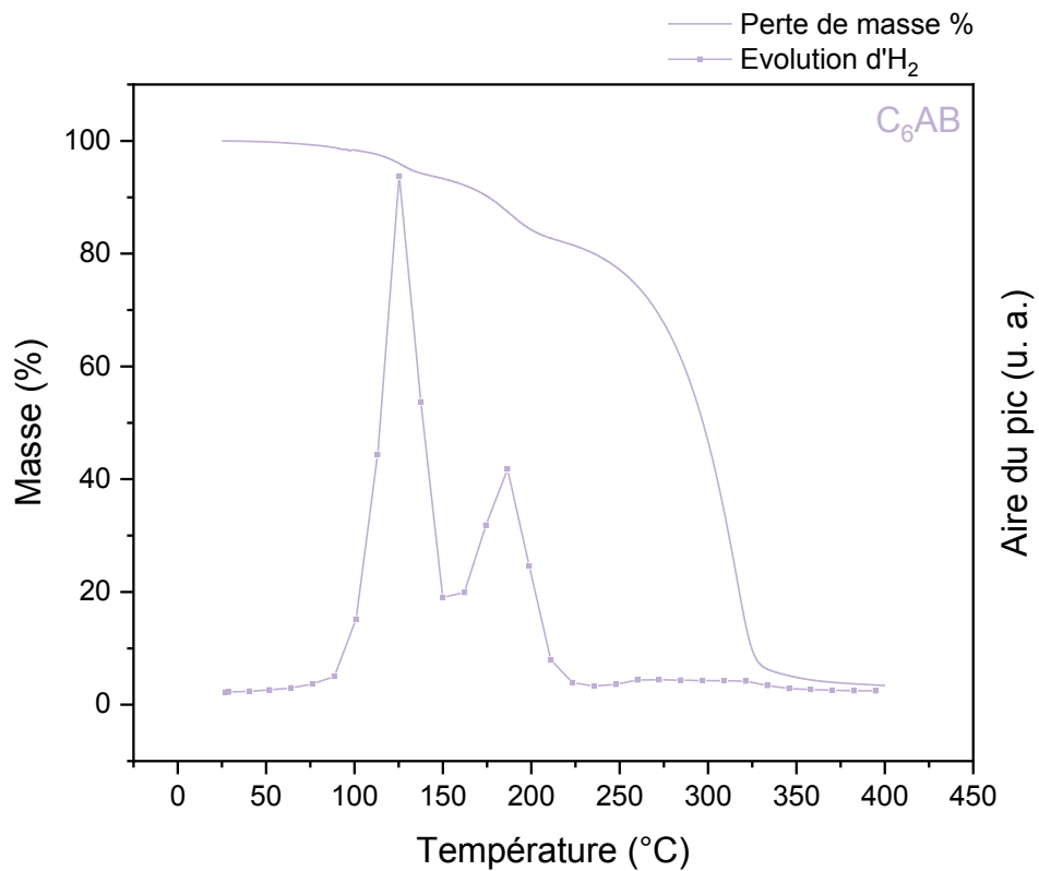
Figure A14 : Analyse ATG/ \mu GC-MS du C 6 AB de 25 à 400 °C (5 °C.min -1 ), m_{C_6AB} = 14,84 mg
