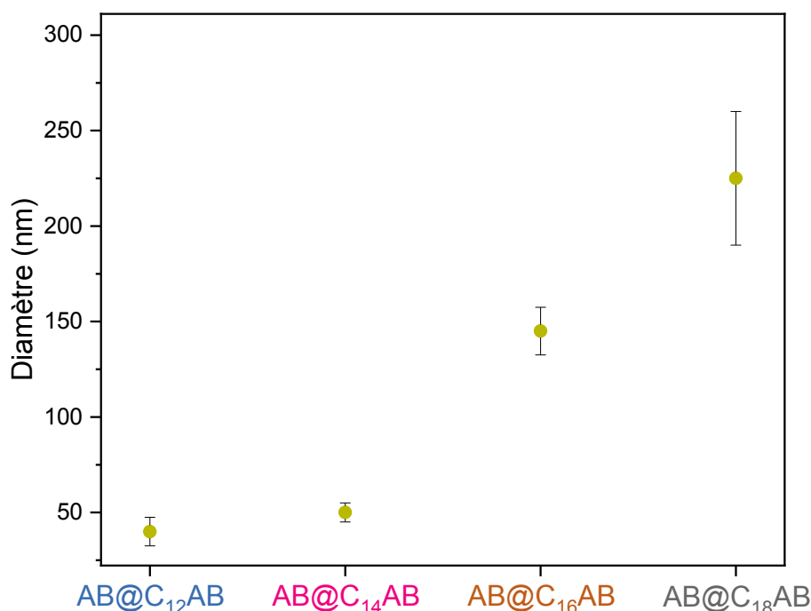
Figure 13 : Evolution des tailles moyennes des particules AB@C x AB en fonction x à l'échelle logarithmique, x étant la longueur de la chaîne alkyle C x AB
