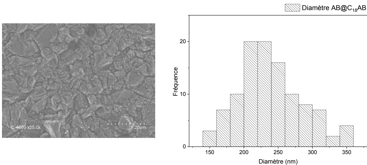
Figure 15 : Histogramme statistique (à droite) de la taille des particules observées sur l'image MEB (à gauche)
