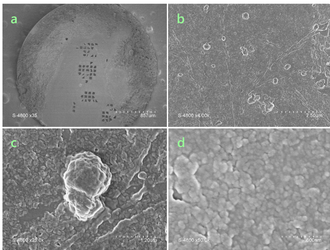
Figure 18 : Micrographes MEB d'ammonia borane préparé via la méthode d'antiprécipitation avec le CHEAB
