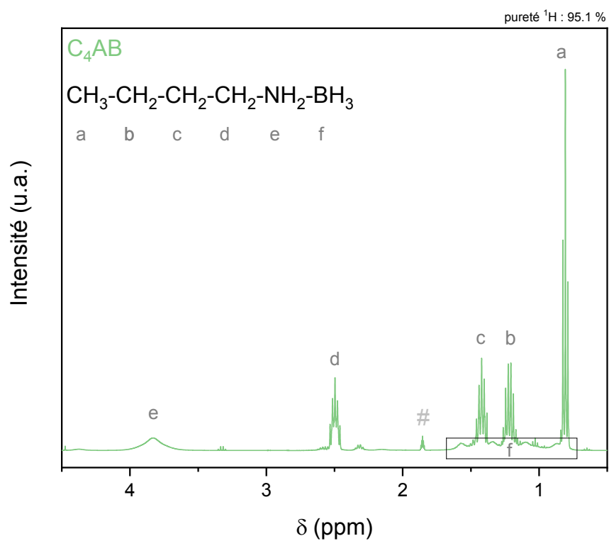
Figure A2 : Spectre RMN liquide du 1 H du C 4 AB solubilisé dans CD 3 CN
