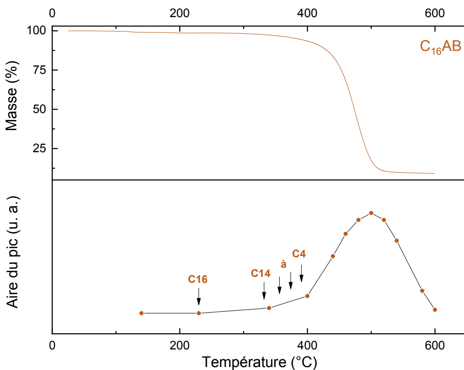
Figure 14 : Thermogramme ATG du C 16 AB (en haut) accompagné d'une représentation graphique (en bas) de l'apparition des gaz de décomposition (alcane et alcène) en fonction de la température
