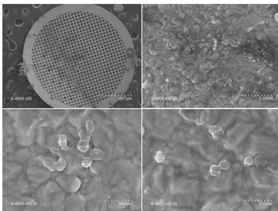
Figure 19 : Micrographes MEB d'ammonia borane préparé via la méthode d'antiprécipitation avec le C2C6AB
