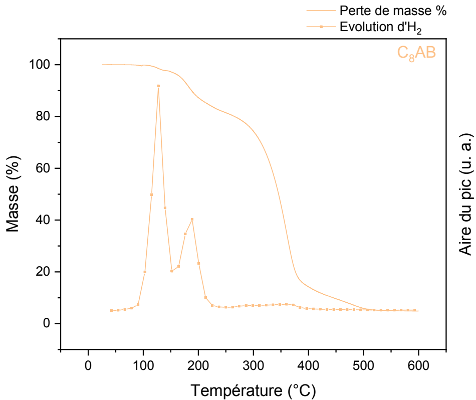
Figure A16 : Analyse ATG/ \mu GC-MS du C 8 AB de 25 à 600 °C (5 °C.min -1 ), m C 8 AB =13,85 mg
