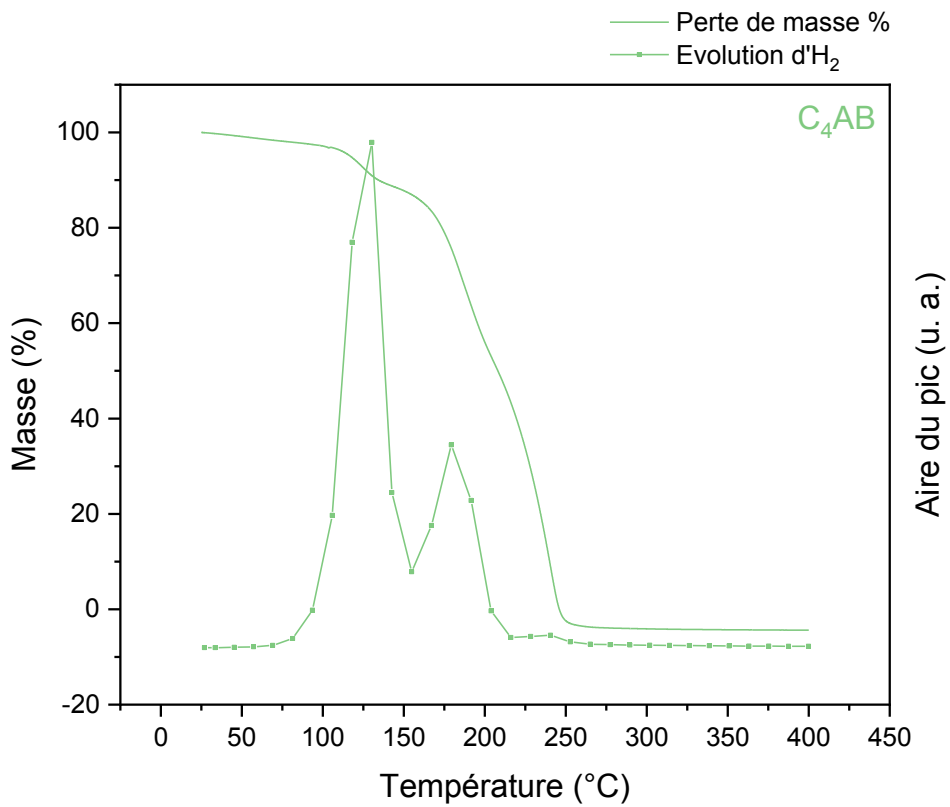
Figure A12 : Analyse ATG/ \mu GC-MS du C 4 AB de 25 à 400 °C (5 °C.min -1 ), m C 4 AB = 10,99 mg
