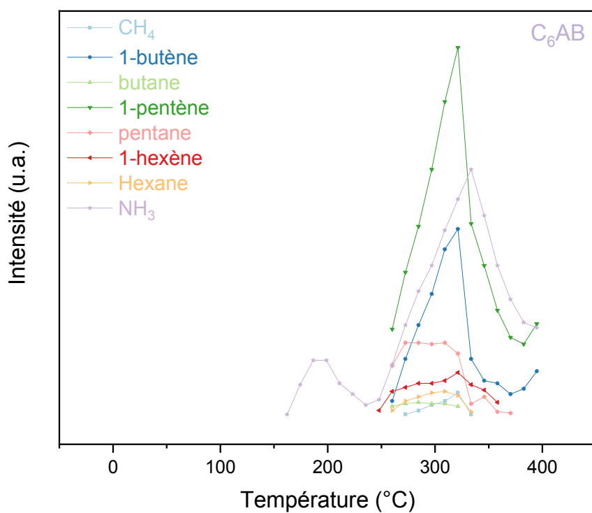
Figure A15 : Suivi de l'évolution des gaz de décomposition du C 6 AB en fonction de la température, obtenu par ATG/ \mu GC-MS
