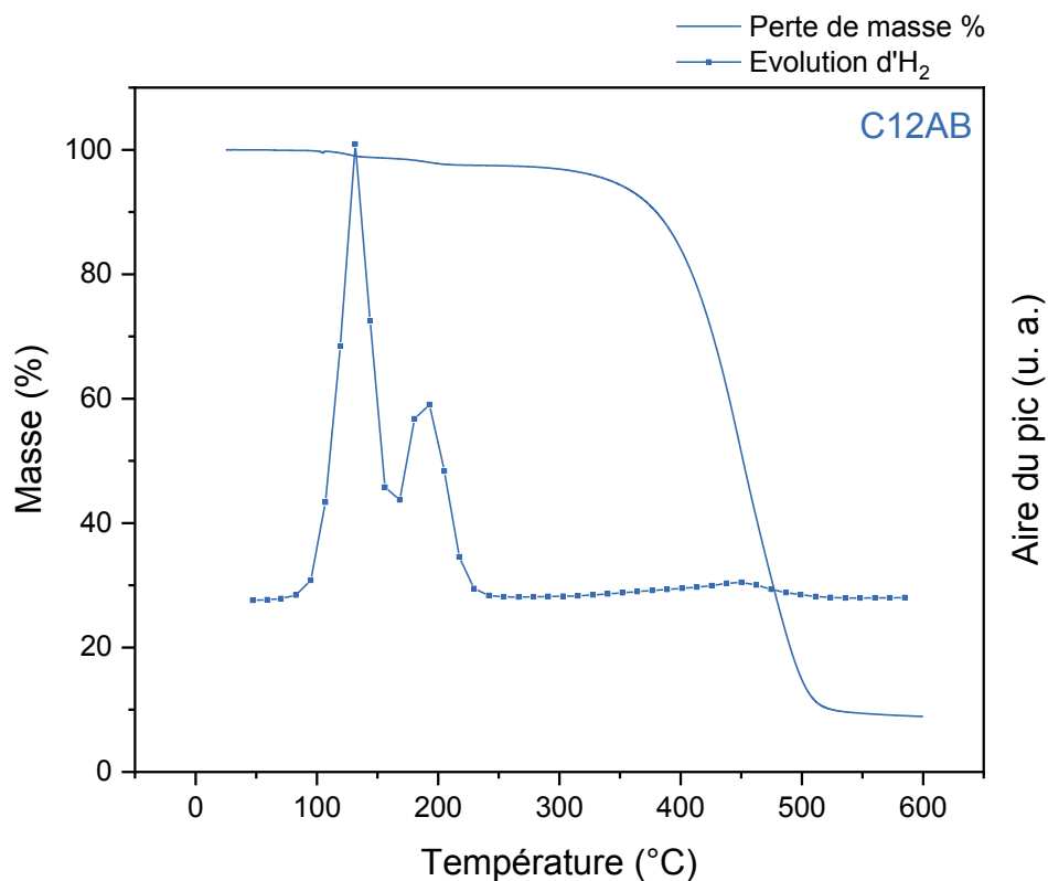
Figure A20 : Analyse ATG/ \mu GC-MS du C 12 AB de 25 à 600 °C (5 °C.min -1 ), m C12AB =12,48 mg
