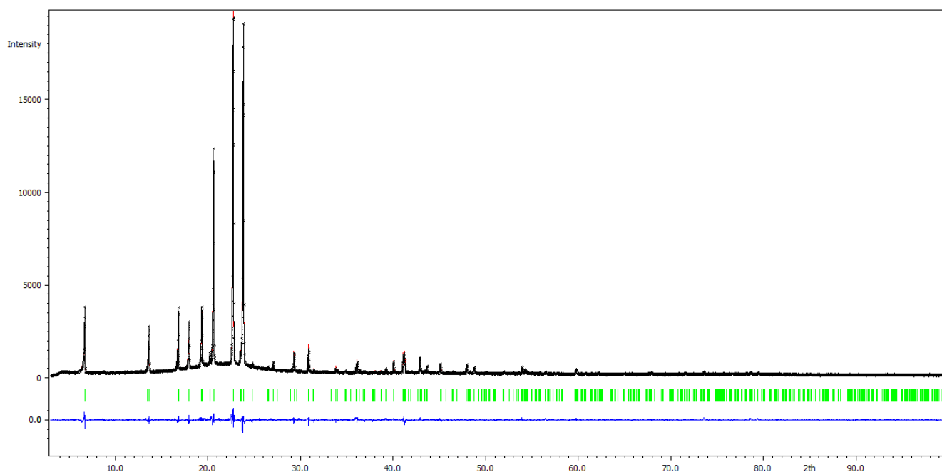
Figure A28 : Diffractogramme des rayons X observé (ligne noire) et calculé (ligne rouge) par affinement Rietveld de C_8AB . La courbe du bas (en bleu) est le tracé de leur différence sur la même intensité d'échelle et les repères (en vert) sont les angles calculés pour les pics de Bragg en 2\theta
