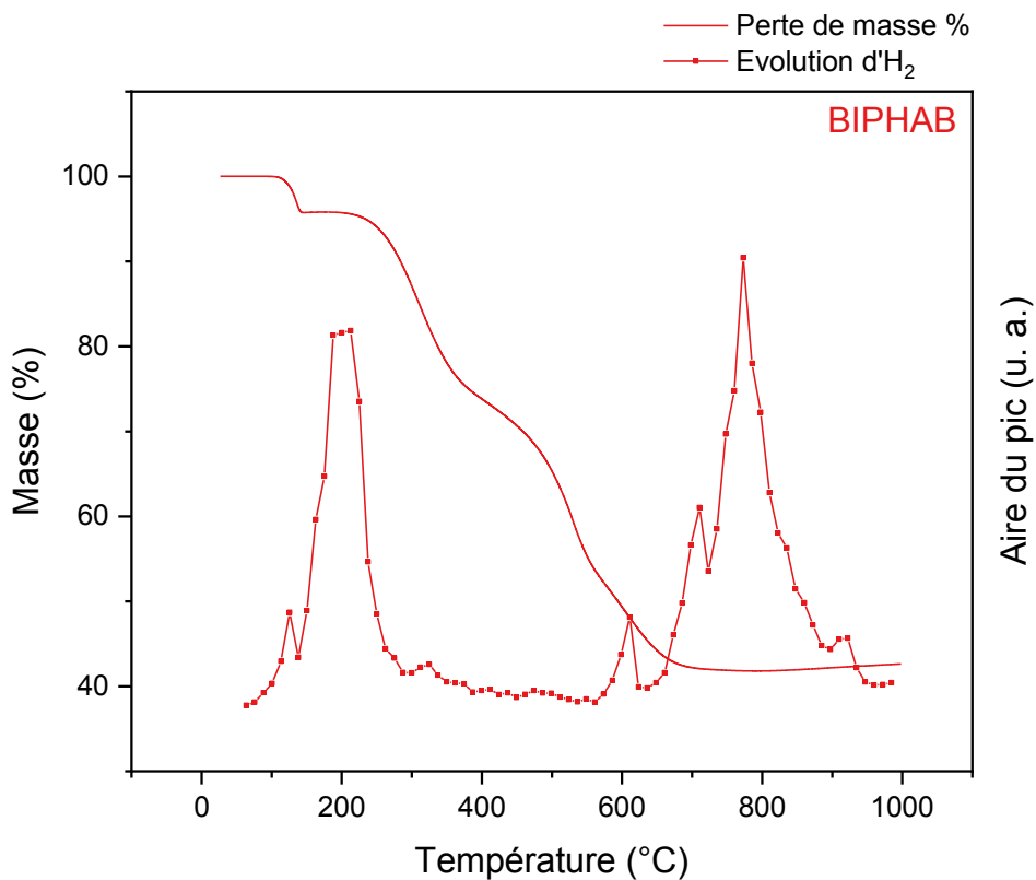
Figure 24 : Analyse ATG/ \mu GC-MS du BIPHAB de 25 à 1000 °C (5 °C.min -1 ), m_{\text{BIPHAB}}=20,01 mg
