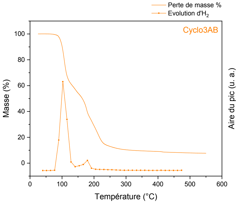
Figure 32 : Analyse ATG/ \mu GC-MS du Cyclo3AB de 25 à 600 °C (5 °C.min -1 ), m_{\text{Cyclo3AB}}=16,42 mg
