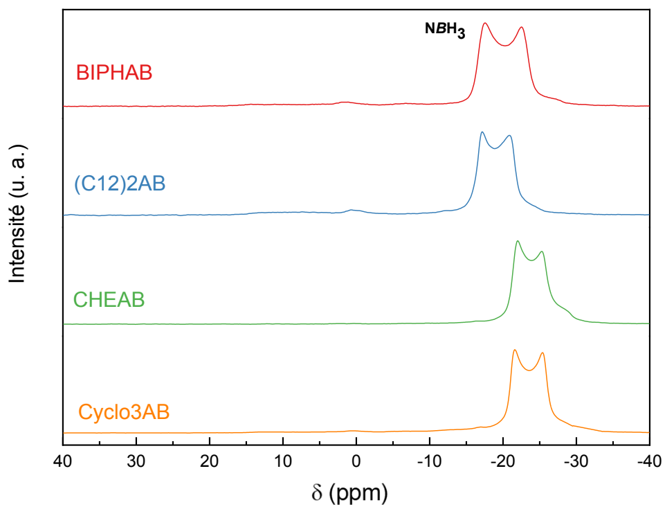
Figure 19 : Spectres RMN solide à l'angle magique du ^{11}\text{B} des NAB
