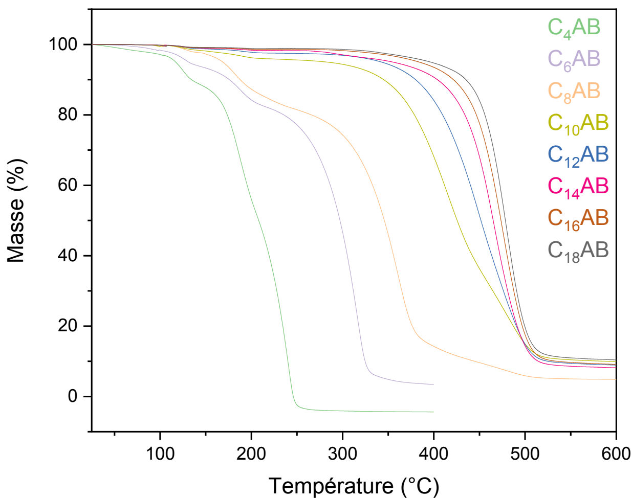
Figure 12 : Thermogrammes ATG de 25 à 400 °C (5 °C.min -1 ), sous N 2 , pour C 4 AB (m=10,99 mg) et C 6 AB (m=14,84 mg) ; de 25 à 600 °C (5 °C.min -1 ) pour C 8 AB (m=13,45 mg), C 10 AB (m=11,96 mg), C 12 AB (m=12,48 mg), C 14 AB (m=14,52 mg), C 16 AB (m=12,06 mg) et C 18 AB (m=14,42 mg)
