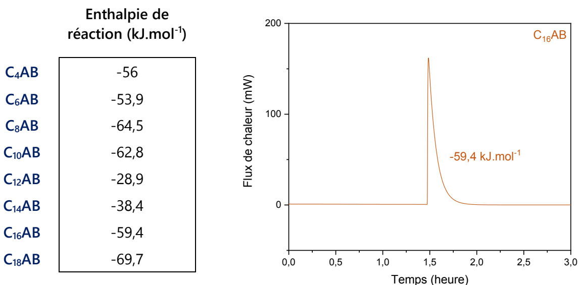
Figure 2 : Liste des enthalpies de réaction (kJ.mol -1 ) pour les différents C x AB ; x étant le nombre de carbone des C x AB (à gauche) et graphe obtenu suite à l'analyse de la synthèse du C 16 AB par calorimètre Calvet C80 (à droite)
