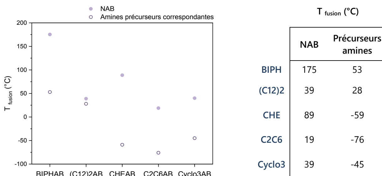
Figure 21 : Comparaison des températures de fusion des NAB par rapport à leur précurseur amine
