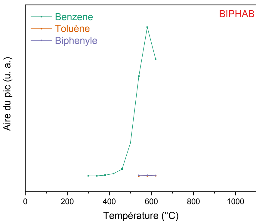
Figure 25 : Suivi de l'évolution des gaz de décomposition du BIPHAB en fonction de la température, obtenu par ATG/ \mu GC-MS
