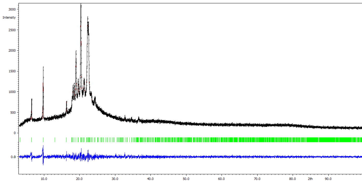
Figure 35 : Diffractogramme des rayons X observé (ligne noire) et calculé (ligne rouge) par affinement LeBail du (C12)2AB. La courbe du bas (en bleu) est le tracé de leur différence sur la même intensité d'échelle et les repères (en vert) sont les angles calculés pour les pics de Bragg en 2\theta
