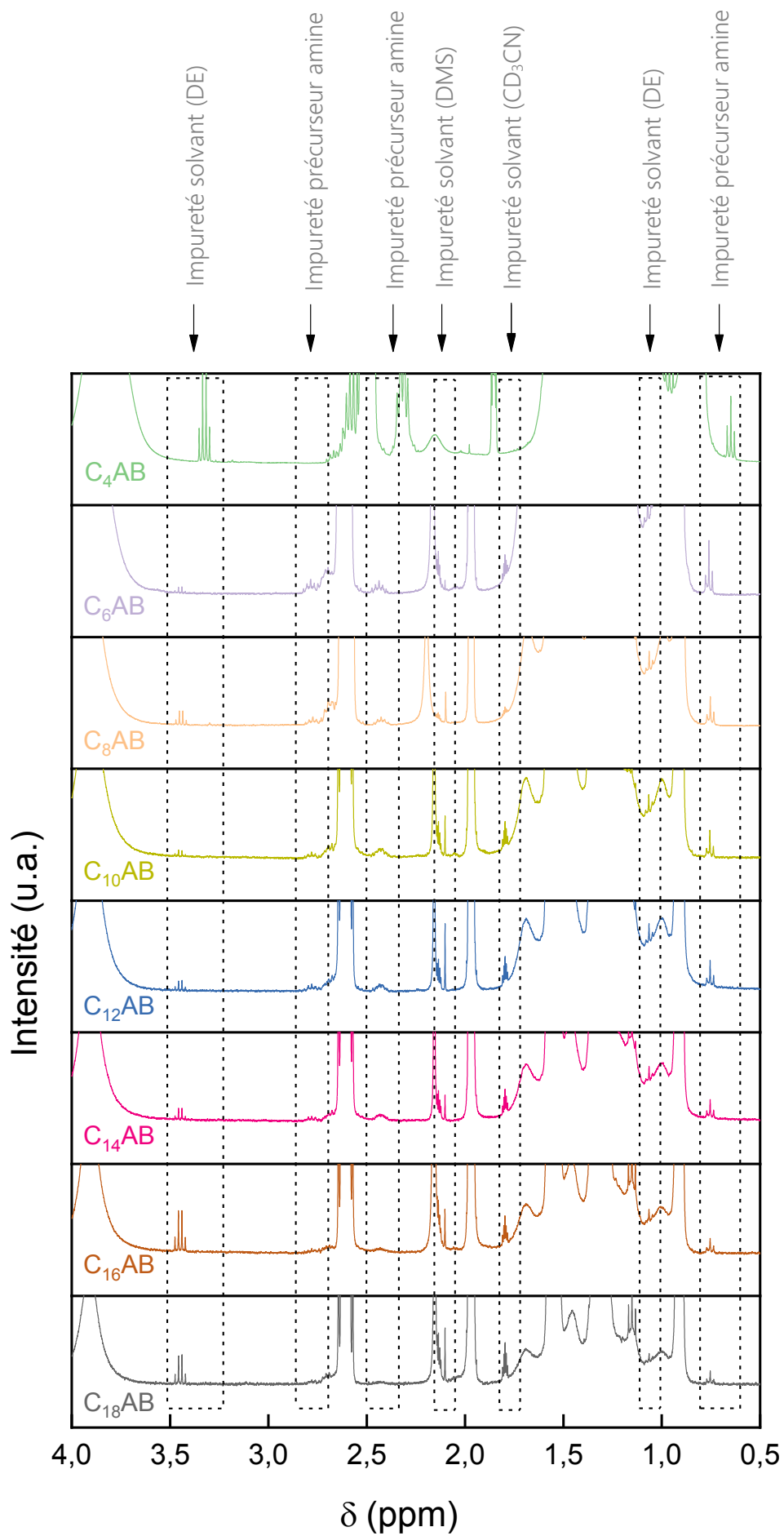
Figure A10 : Spectres RMN liquide du ^1\text{H} avec zoom sur les impuretés présentes dans les \text{C}_x\text{AB} solubilisés dans \text{CD}_3\text{CN}
