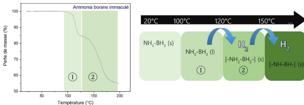
Figure 4 : Analyse thermogravimétrique de l'ammonia borane à l'état brut accompagné du schéma de la perte associé des deux premiers équivalents \text{H}_2 (soit 200 °C)
