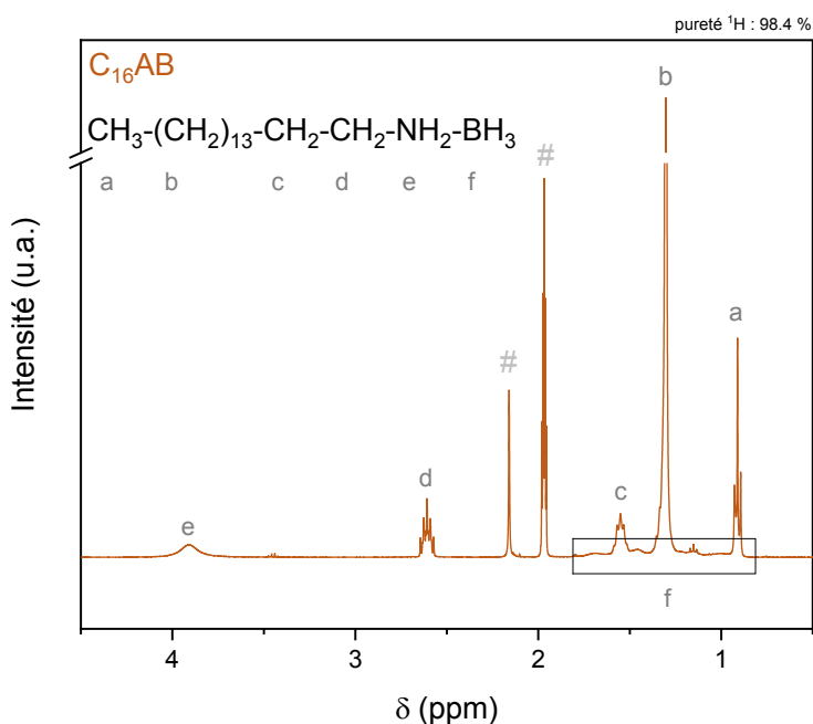
Figure 6 : Spectre RMN liquide du ^1\text{H} du \text{C}_{16}\text{AB} solubilisé dans \text{CD}_3\text{CN} d-3
