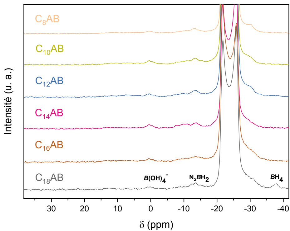
Figure 9 : Spectres RMN solide à l'angle magique du ^{11}\text{B} des \text{C}_x\text{AB}
