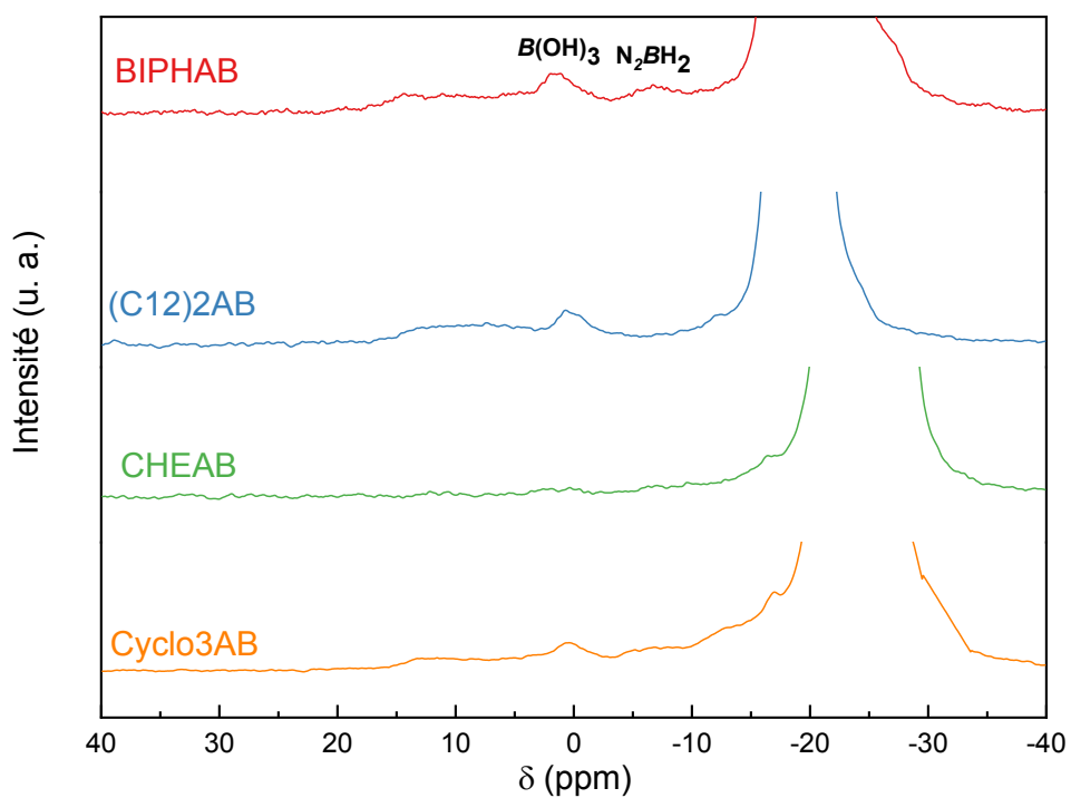
Figure 20 : Spectres RMN solide à l'angle magique du ^{11}\text{B} des NAB
