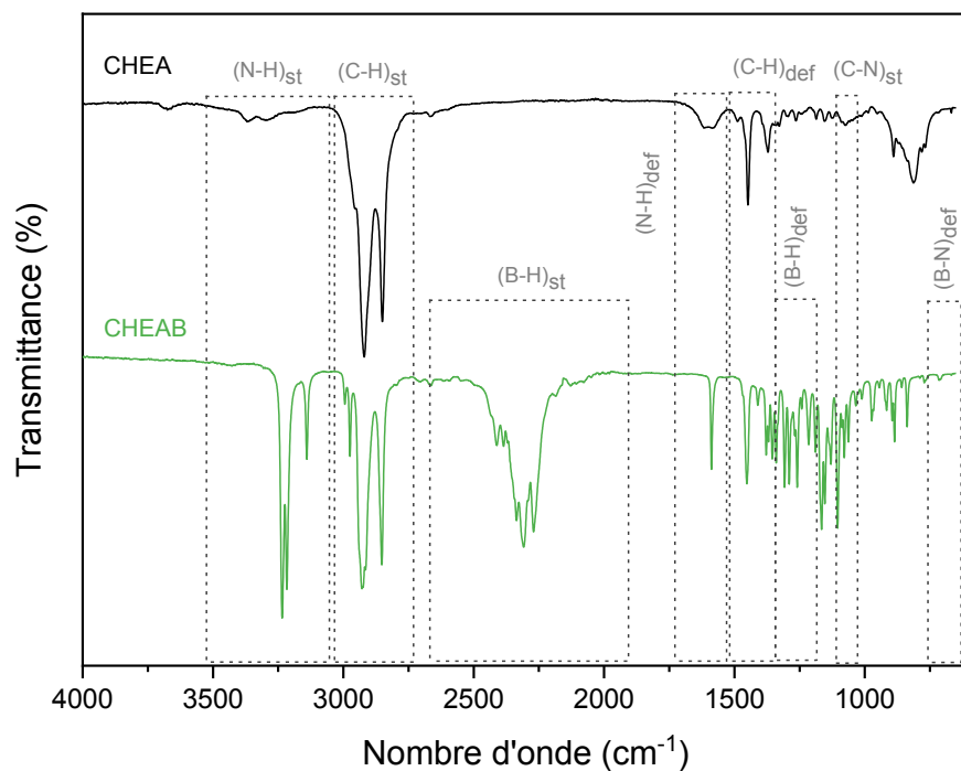
Figure 4 : Spectre IRTF du CHEA (en haut) et du CHEAB (en bas)
