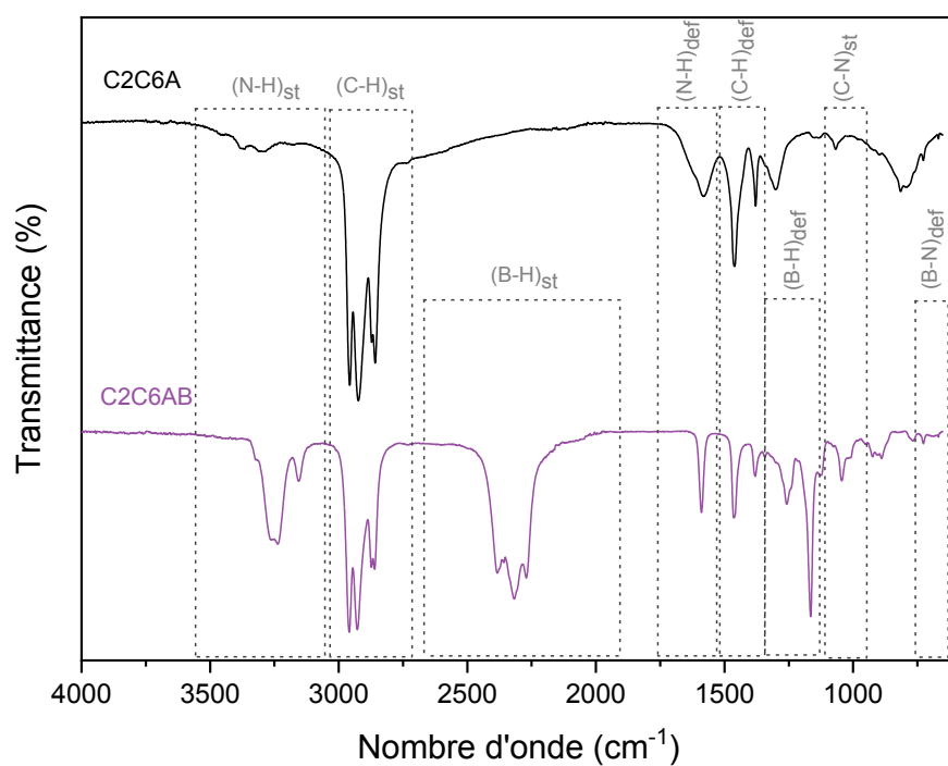
Figure 5 : Spectre IRTF du C2C6A (en haut) et du C2C6AB (en bas)
