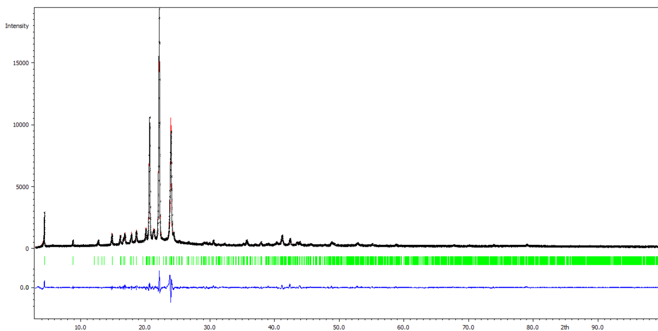
Figure A31 : Diffractogramme des rayons X observé (ligne noire) et calculé (ligne rouge) par affinement Rietveld de C 14 AB. La courbe du bas (en bleu) est le tracé de leur différence sur la même intensité d'échelle et les repères (en vert) sont les angles calculés pour les pics de Bragg en 2θ
