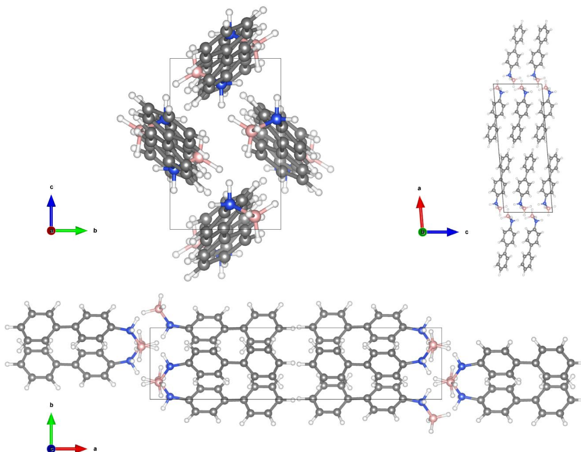
Figure 37 : Structure cristalline du BIPHAB ; les atomes H, B, N et C sont représentés en blanc, rose, bleu et gris foncé respectivement
