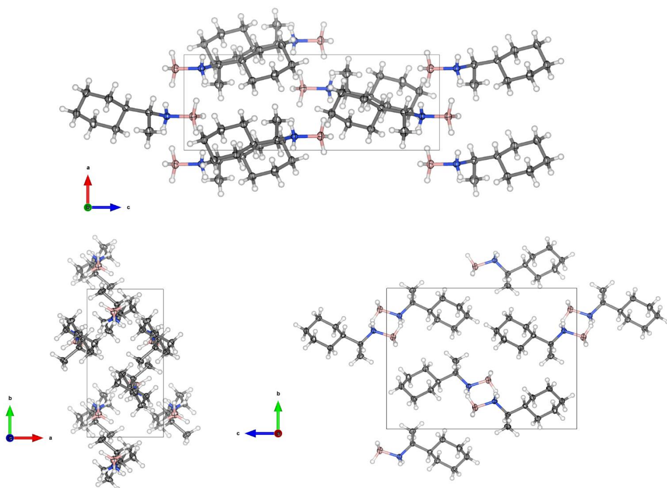
Figure 38 : Structure cristalline du CHEAB ; les atomes H, B, N et C sont représentés en blanc, rose, bleu et gris foncé respectivement
