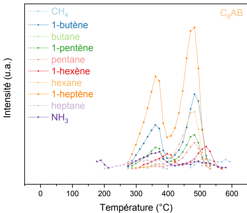
Figure A17 : Suivi de l'évolution des gaz de décomposition du C 8 AB en fonction de la température, obtenu par ATG/ \mu GC-MS
