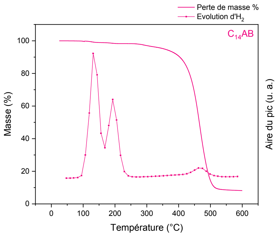
Figure A21 : Analyse ATG/ \mu GC-MS du C 14 AB de 25 à 600 °C (5 °C.min -1 ), m C14AB =14,52 mg
