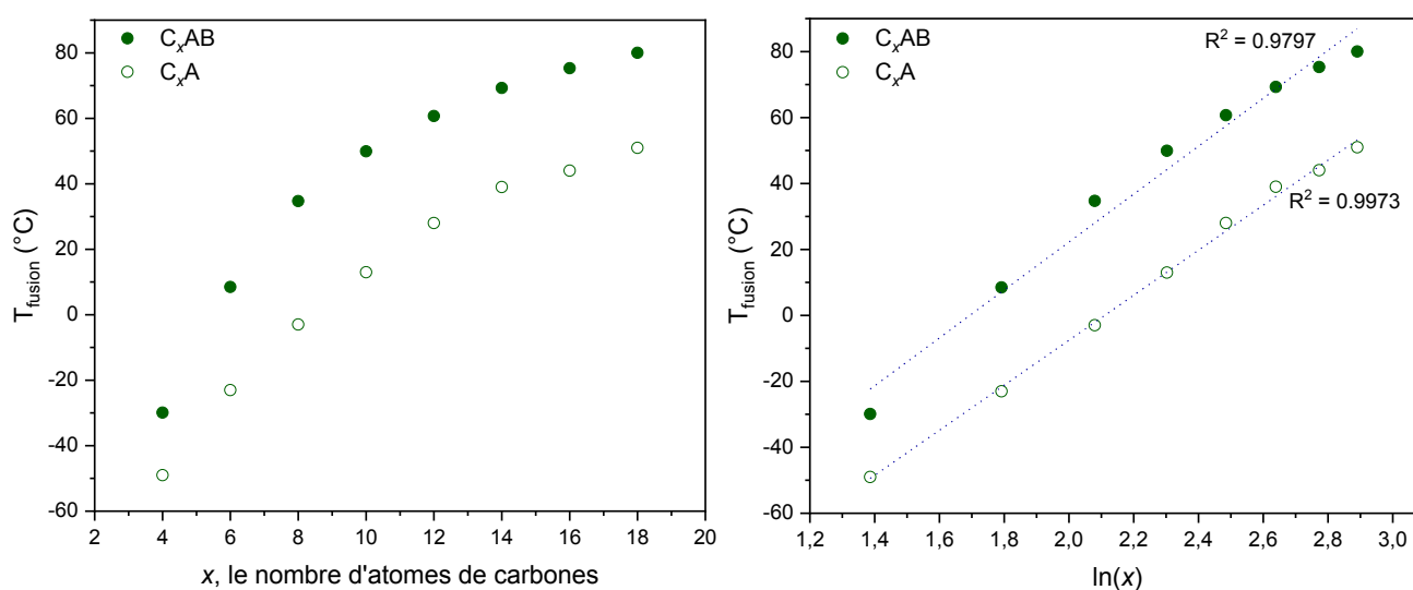
Figure 10 : Évolution des températures de fusion en fonction du nombre d'atomes de carbones des C_xA et C_xAB (à gauche) et en fonction de \ln(x) (à droite)
