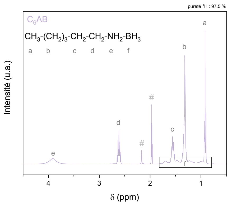
Figure A3 : Spectre RMN liquide du 1 H du C 6 AB solubilisé dans CD 3 CN
