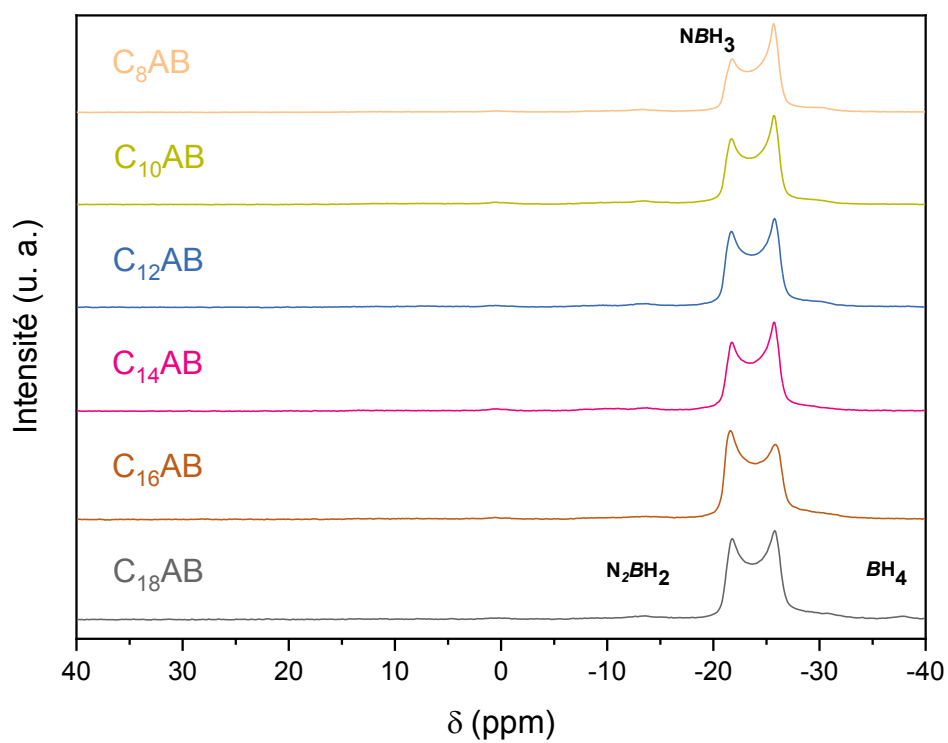
Figure 8 : Spectres RMN solide à l'angle magique du ^{11}\text{B} des \text{C}_x\text{AB}
