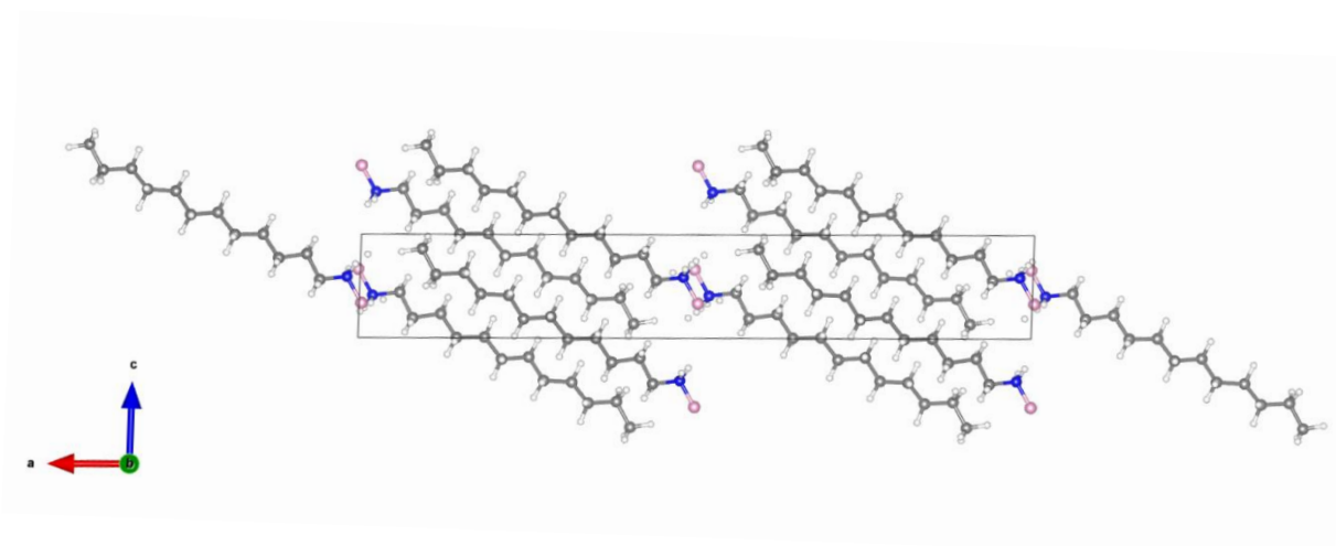
Figure 1 : Modèle structural du C_{12}AB obtenu par l'affinement des résultats de DRX, selon l'axe b permettant de mettre évidence les interactions dihydrogènes B-H^{\delta-} \cdots H^{\delta+}-N
