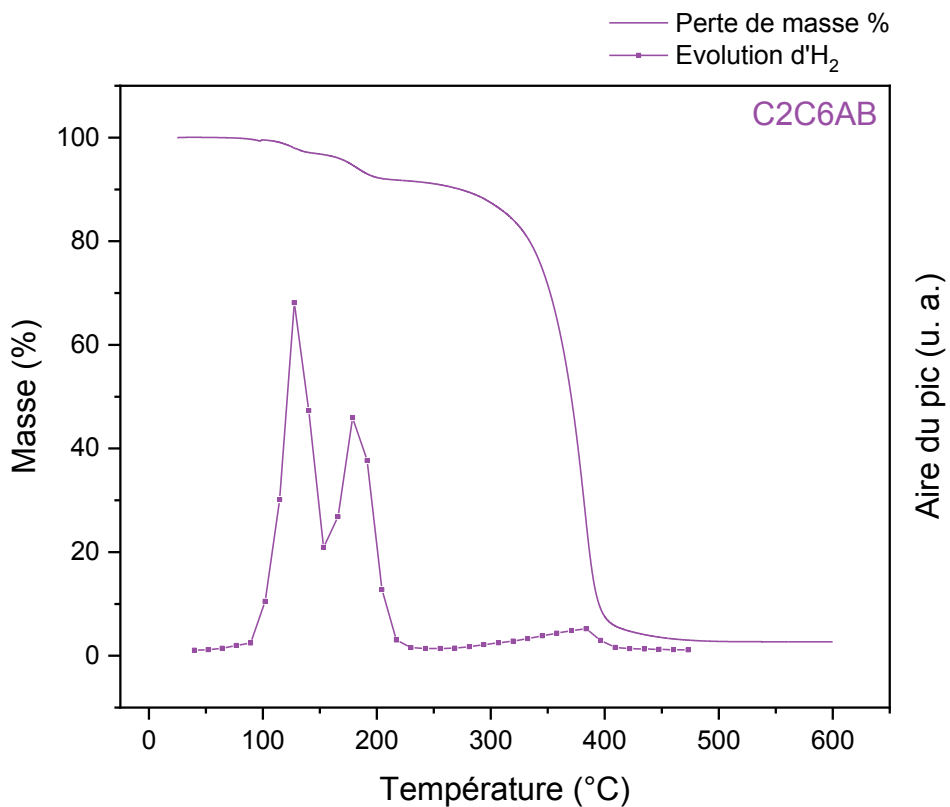
Figure 30 : Analyse ATG/ \mu GC-MS du C2C6AB de 25 à 600 °C (5 °C.min -1 ), m_{\text{C2C6AB}}=25,31 mg
