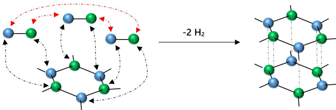
Figure 8 : Formation schématique de la borazine par empilement de l'ammonia borane sur le réseau hexagonal BN selon Demirci 55
