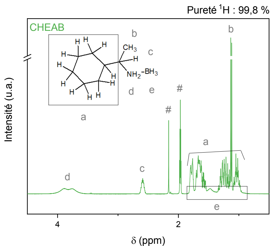
Figure 14 : Spectre RMN liquide du ^1\text{H} du CHEAB solubilisé dans \text{CD}_3\text{CN} (# = signaux confirmant la présence d'impuretés provenant du solvant deutéré)
