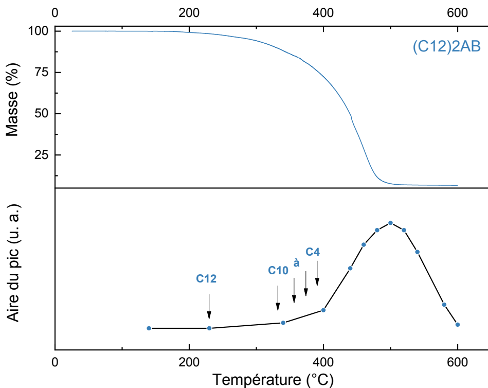
Figure 27 : Thermogramme ATG du (C12)2AB (en haut) accompagné d'une représentation graphique (en bas) de l'apparition des gaz de décomposition (alcane et alcène) en fonction de la température
