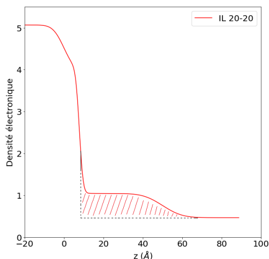
FIGURE 5.21 – Surplus d’électrons à la surface de l’électrode par rapport à une surface platinée / liquide ionique idéale ; exemple du profil de l’échantillon
