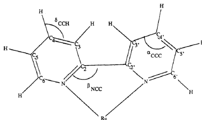
FIGURE 3.10 – Structure du \text{Ru}(\text{bpy})_3 , notations des angles utilisés au tableau 3.3, reproduit de [55]. La structure de cet ion \text{Ru}(\text{bpy})_3 est très semblable à celle du \text{Co}(\text{bpy})_3 (figure 3.2)
