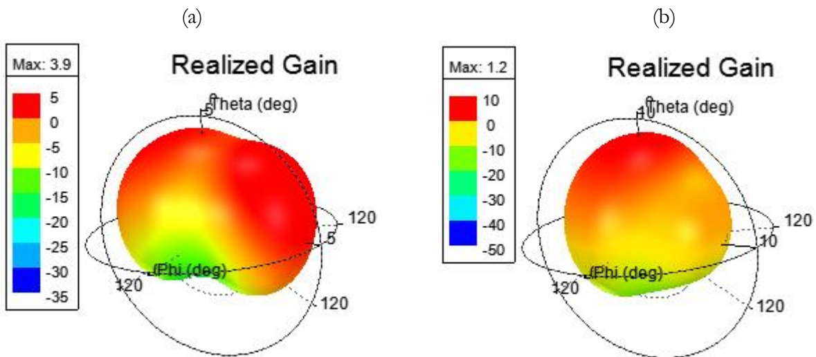
Figure 3- 10 : Gain obtenu par simulation pour les deux fréquences de résonances de l'antenne patch circulaire entourée de structures de type champignons.
