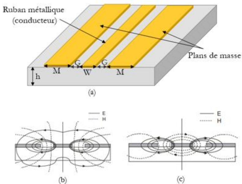
Figure 1- 17 : Ligne coplanaire : (a) Structure géométrique. (b) mode pair et (c) mode impair (figure extraite de [Sghier2013]).
