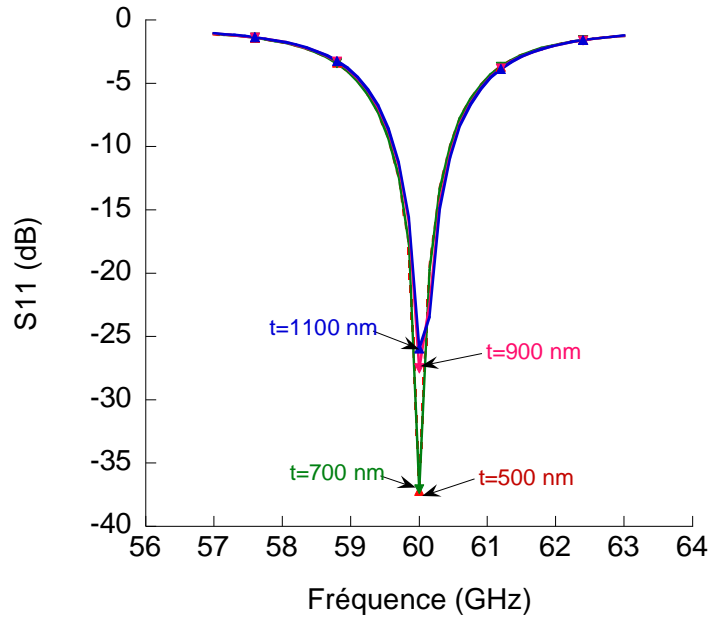
Figure 3- 27 : Coefficient de réflexion (dB) de l'antenne patch rectangulaire sur BCB en fonction de la fréquence pour différentes épaisseur de métallisation.
