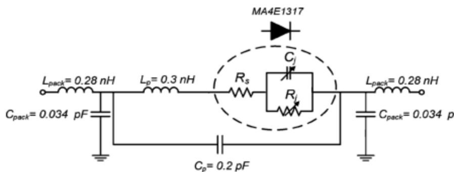
Figure 4- 21 : Modèle de circuit réel de la diode Schottky et ses paramètres parasites (incluant le packaging), figure extraite de [Shabnam2015].
