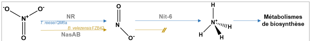
Figure 35 : Réduction du nitrate par voie assimilatoire chez T. reesei QM6a et B. velezensis FZB42 en nitrite par la nitrate réductase NR et NasAB respectivement, puis en ammonium par la nitrite réductase Nit6 chez Trichoderma . Le gène codant pour une nitrite réductase (NirA) dans Bacillus n'est pas présent chez B. velezensis (d'après KEGG)
