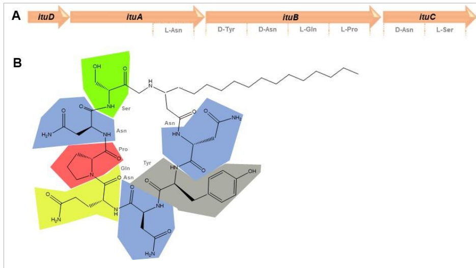
Figure 8 : (A) Opéron itu formé de 4 gènes : ituA , ituB , ituC , ituD codant pour les synthétases nonribosomiques responsables de l'incorporation des 7 monomères composants l'iturine, (B) Structure cyclisée de l'iturine présentant une chaîne d'acide gras linéaire de 16 atomes de carbone (la taille de la chaîne d'acide gras pouvant varier de 14 à 17 atomes de carbone) (d'après Tsuge et al. , 2005)
