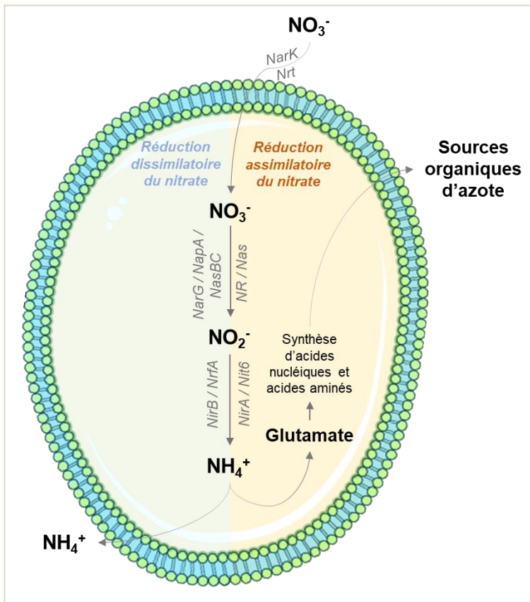
Figure 11 : Utilisation du nitrate extracellulaire par voie dissimilaire (le nitrate est réduit en nitrite puis en ammonium sécrété) et assimilatoire (le nitrate est réduit en nitrite puis en ammonium qui servira à la synthèse du glutamate). L'azote présent sur le glutamate servira ensuite à la synthèse d'autres molécules azotées tels que d'autres acides aminés et les acides nucléiques qui pourront éventuellement être excrétés dans le milieu extracellulaire.
