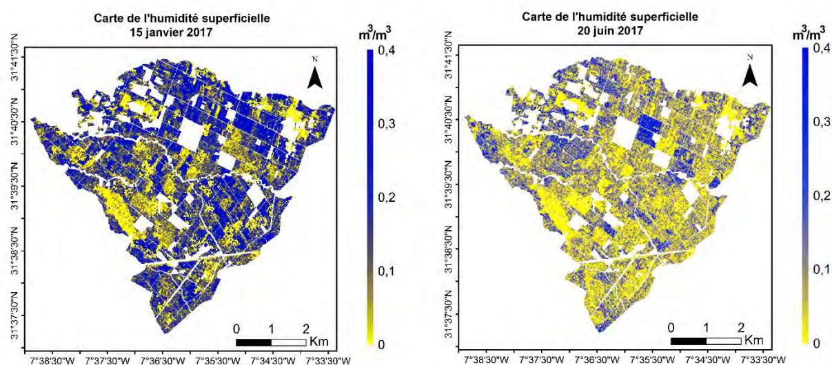
Figure V. 4 : Cartes d'humidité de surface du sol sur un périmètre irrigué situé à 40 km à l'est de Marrakech nommé R3 pour deux conditions de SSM différentes : condition humide (15 janvier 2017) et condition sèche (20 juin 2017).
