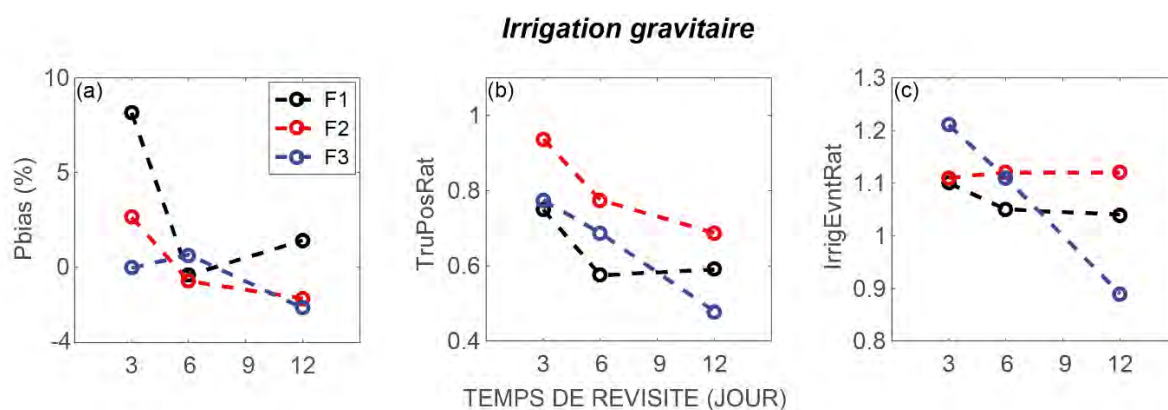
Figure VI. 6 : Statistiques (Pbias (a), TruPosRat (b) et IrrigEvntRat (c)) sur les parcelles F1, F2 et F3 irriguées en gravitaire pour différentes fréquence d'observations : 3, 6 et 12 jours.
