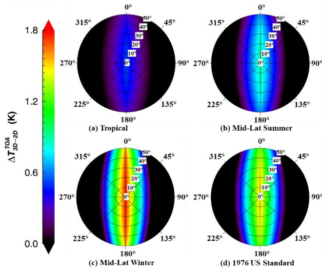
Fig. 8. Amplitude de l'impact des structures 3-D et de leur rayonnement sur les mesures TIR sur un canyon de rue observé par satellite pour différents types atmosphériques. Les paramètres supplémentaires requis ont été définis comme valeurs par défaut répertoriées dans Table 2.
