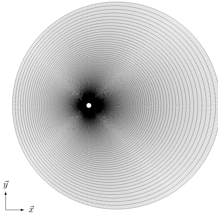
FIGURE 3.11 – Vue d'ensemble du maillage utilisé.
