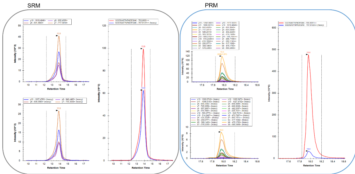
Figure II-36. Comparaison de la quantification d'un peptide d'OspC par microLC-SRM et nanoLC-PRM dans une biopsie cutanée de patient. Le peptide GGDSASTNPDESAK (OspC) a été quantifié dans la biopsie 003-044 par SRM et PRM avec des valeurs de 3,5 fmol/mg biopsie et 192,7 pmol/ mg biopsie, respectivement.
