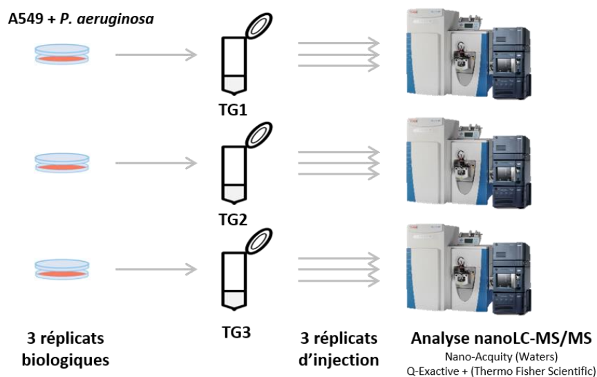
Figure IV-8. Analyse de la reproductibilité biologique et de la répétabilité technique. Trois lots de cellules A549 infectées par P. aeruginosa ont été préparés par TG (TG1, TG2, TG3), puis chaque mélange peptidique a été analysé 3 fois (Inj1, Inj2, Inj3) par nanoLC-MS/MS (750 ng injectés).
