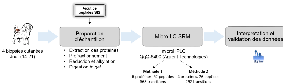
Figure II-14. Analyse des peaux de chiens infectés en ciblant neuf protéines de Borrelia . Les protéines sont extraites de la peau par broyage manuel puis préfractionnées sur gel SDS-PAGE (20 bandes). Après réduction/alkylation des protéines, les peptides SIS sont ajoutés aux bandes, puis la digestion par la trypsine est effectuée. Les peptides sont analysés par LC-SRM avec les deux méthodes M1 et M2 (1 protéine commune aux deux méthodes), et les données sont interprétées à l'aide du logiciel Skyline.
