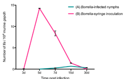
Figure II-5. Quantification par PCR de B. burgdorferi dans des biopsies cutanées de souris après une infection via des tiques ou inoculation à la seringue (A. Kern et al. , 2011)
