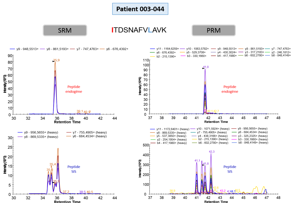
Figure II-29. Traces SRM et PRM du peptide ITDSNAFVLAVK (OspC) dans une biopsie cutanée de patient. La biopsie 003-044 a été analysée en parallèle par les deux méthodes. Dans les deux cas, les 4 isoformes du peptide SIS (I/L)TDSNAFV(L/I)AVK ont été ajoutées. Le peptide endogène est co-élué avec le troisième pic correspondant bien à la séquence ciblée.
