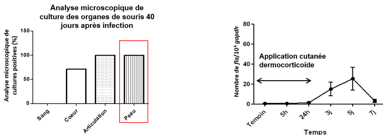
Figure II-38. Mise en évidence de la latence cutanée de Borrelia dans la peau de souris infectée par inoculation intra-dermique. Panel de gauche : Mesure de la présence de Borrelia dans différents organes 40 jours après une inoculation des bactéries. Panel de droite : Quantification PCR du gène codant la flagelline après l'application locale du clobetasol sur la peau de souris 40 jours après l'infection.
