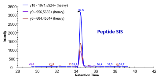
Figure II-19. Illustration du décalage de Tr pour deux répliquats d'analyse de la biopsie 001-001. Tous les critères de validation sont satisfaits pour le répliquat 1 (co-élution des transitions, respect du rapport des transitions, co-élution des peptides SIS et endogène). Par contre pour le répliquat 2, les peptides SIS et endogène ne sont pas bien co-élus.
