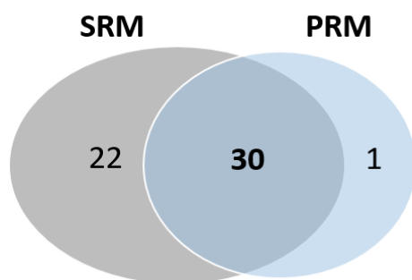
Figure II-24. Nombre de peptides pour lesquels la LLOQ par spectrométrie de masse ciblée a été déterminée. Les LLOQ de 53 peptides sur les 56 ciblés ont été déterminées par LC-SRM et/ou LC-PRM.
