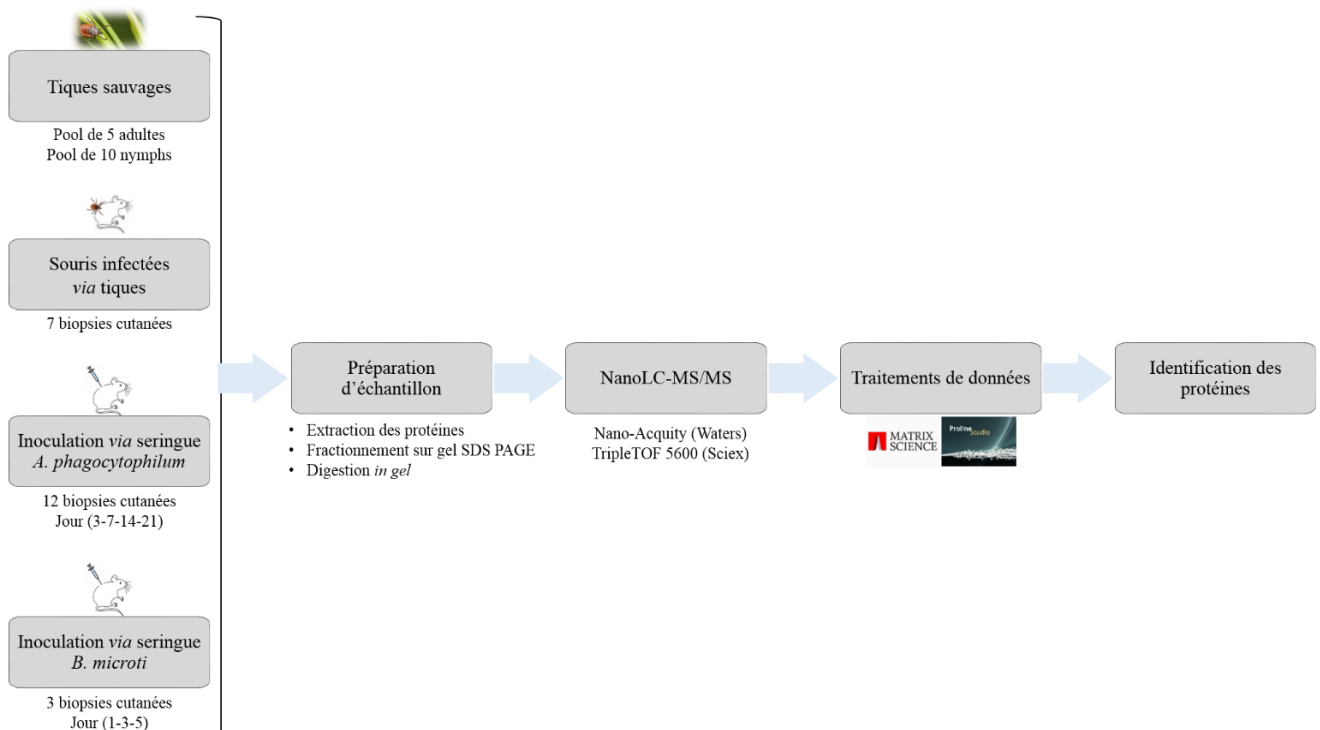
Figure III-3. Stratégie analytique d'identification des protéines dans les tiques et peaux de souris. Les protéines sont extraites et séparées sur gel SDS-PAGE. Les pistes de gel sont découpées en bandes de 2 mm. La digestion in gel est effectuée par la trypsine. Les peptides générés sont analysés par nanoLC-MS/MS. Les données générées sont traitées par l'algorithme de recherche Mascot et la validation des protéines est effectuée par le logiciel Proline.
