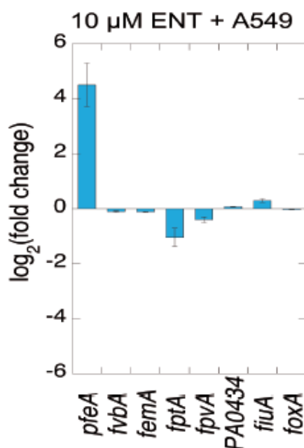
Figure IV-19. Histogramme représentant les variations d'abondance des gènes codant des protéines de P. aeruginosa dans des cellules infectées en présence de 10 \mu\text{M} ENT. La RT-qPCR a été réalisée sur des cellules A549 infectées par P. aeruginosa après 3 d'incubation. Les données ont été normalisées avec le gène de référence uvrD pour les triplicats biologiques.
