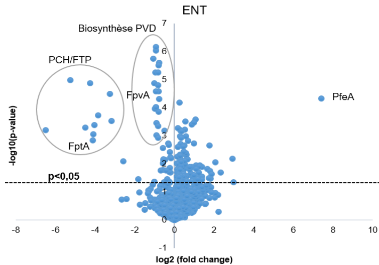
Figure IV-18. Volcano plot représentant les variations d'abondance des protéines de P. aeruginosa dans des cellules infectées en absence (Témoin) ou en présence de 10 \mu M ENT. La statistique a été faite avec un test t de Welch. Sur les 1462 quantifiées, 195 sont différentiellement exprimées ( p < 0,05 ). Les cercles indiquent les protéines impliquées dans les voies pyochéline (PCH) et pyoverdine (PVD).
