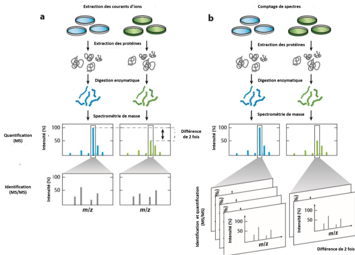
Figure I-15. a. Approche sans marquage et avec extraction de courant d'ions : les échantillons sont digérés séparément, puis analysés par spectrométrie de masse. La quantification relative est obtenue en comparant les signaux MS pour chaque peptide (quantification MS). b. Approches sans marquage et avec comptage de spectres : les échantillons sont digérés séparément, puis analysés par spectrométrie de masse. La quantification relative est obtenue en comparant le nombre de spectres MS/MS pour chaque protéine. Figure adaptée de (J. A. Ankney et al. , 2018)
