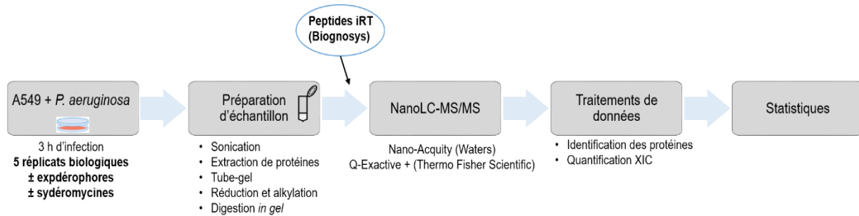
Figure IV-12. Schéma analytique utilisé pour l'étude différentielle des protéines de P. aeruginosa dans des cellules épithéliales pulmonaires infectées, en présence des différents exosidérophores. Chaque échantillon a été préparé indépendamment 5 fois, puis traité dans les mêmes conditions par approche TG et analyse nanoLC-MS/MS (gradient 120 min, 750 ng injectés). Des peptides iRT ont été ajoutés avant l'injection nanoLC-MS/MS. La quantification label-free a été réalisée en extrayant les signaux MS1 (quantification XIC). La banque de données utilisée pour le traitement des données est une banque générée à partir des protéines humaines et des protéines de P. aeruginosa PAO1 de UniProtKB.
