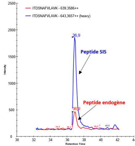
2. Co-élution entre le peptide endogène et le peptide SIS
