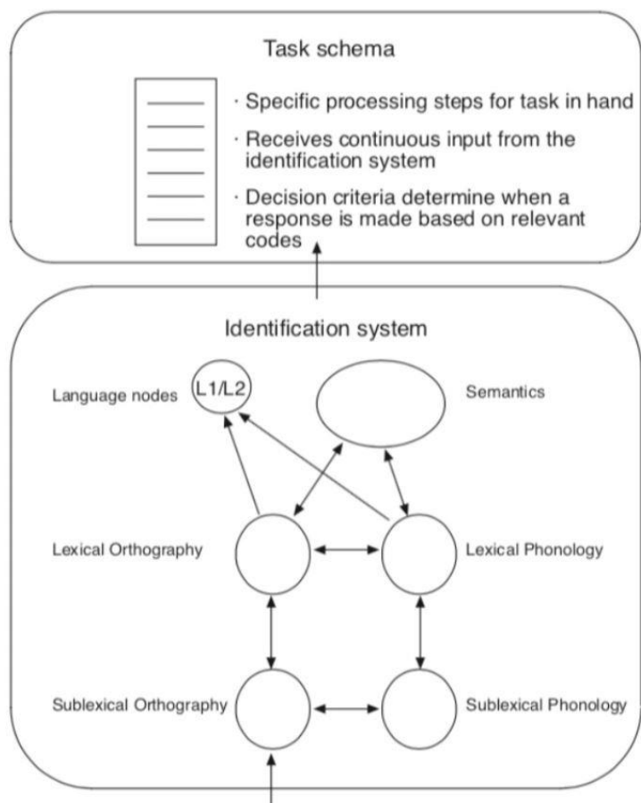
Figure 3. Bilingual Interactive Activation plus (Dijkstra & Van Heuven, 1998 ; Van Heuven, Dijkstra & Grainger, 1998).
