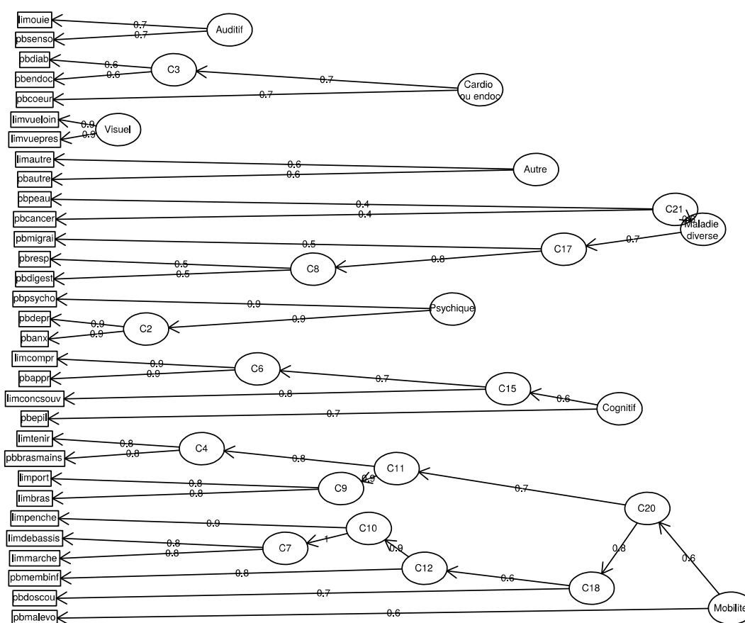
Figure A.2.2 Classification hiérarchique de variables
