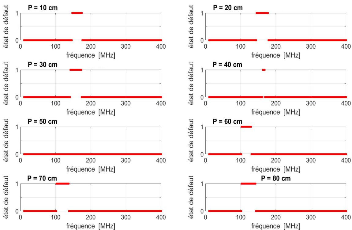
Figure 34 : Mêmes résultats que la Figure 33 pour \tau = 10 dB
