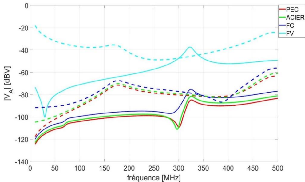
Figure 96 : Tension induite sur l'impédance 50 \Omega reliant l'antenne et la carrosserie pour les différentes métallisations de la carrosserie et les 2 configurations de charges terminales (équilibrée et non équilibrée)
