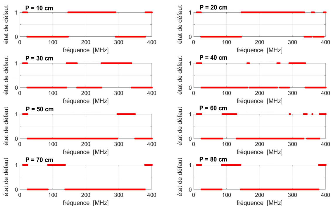
Figure 33 : Intégrité du signal du signal carré (défini par A_u = 1 V et f_u = 50 MHz) sur le câble non blindé d'une longueur de 1m en fonction de la fréquence pour une perturbation appliquée définie par I_{bci} = 100 mA et \tau = 0 dB pour chaque position de la sonde d'injection (une valeur «1» à une fréquence donnée signifie un défaut d'intégrité du signal et un «0» l'absence de défaut).
