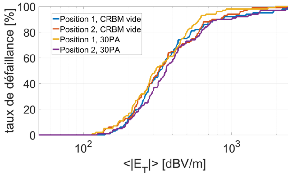
Figure 63 : Taux de défaillance obtenu pour une paire torsadée non-blindée de 1m pour les quatre configurations du montage mentionnées, f_u = 50 MHz, A_u = 1 V et f_p = 500 GHz, \tau = 0 dB.
