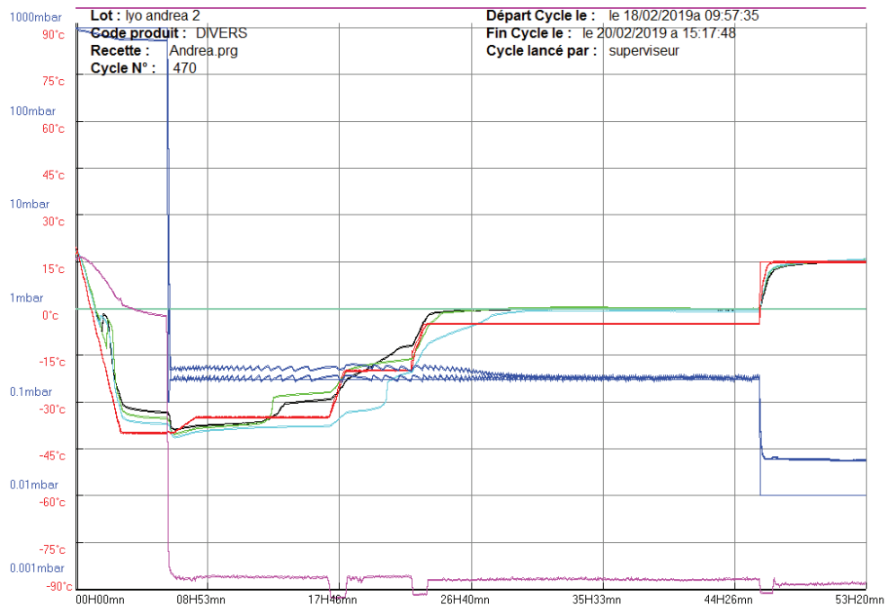
Figure A.3. Conditions opératoires de la lyophilisation.
