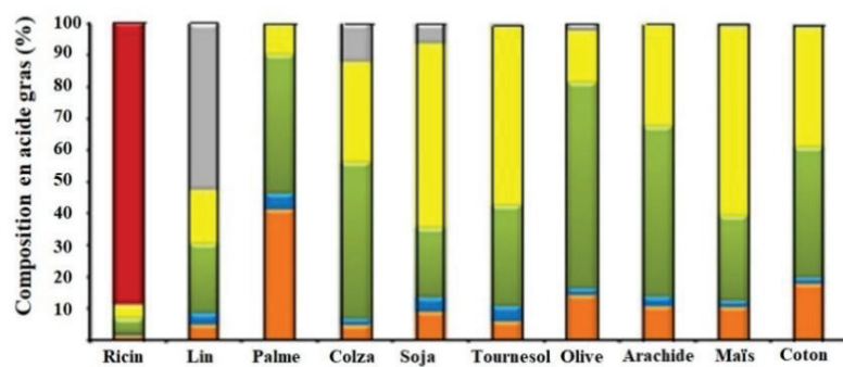
Figure 1.3. Composition moyenne en acide gras (%) de quelques huiles végétales.
