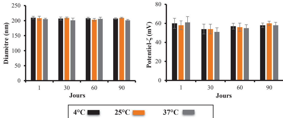
Figure 4.18. Stabilité des nanoparticules à base de PMMA chargées d'huile en termes de taille et de potentiel \zeta .
