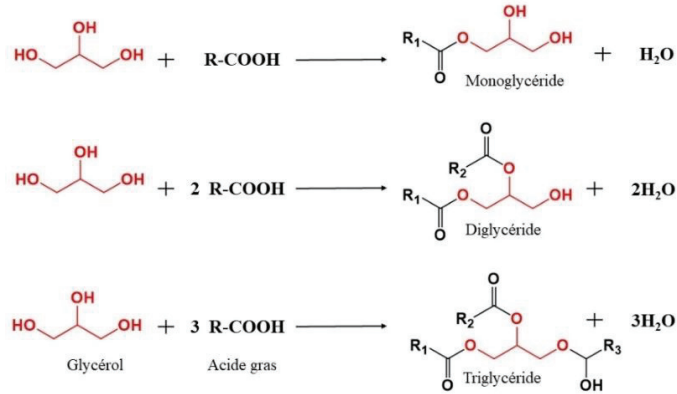
Figure I.2. Représentation schématique des monoglycérides, diglycérides et triglycérides.
