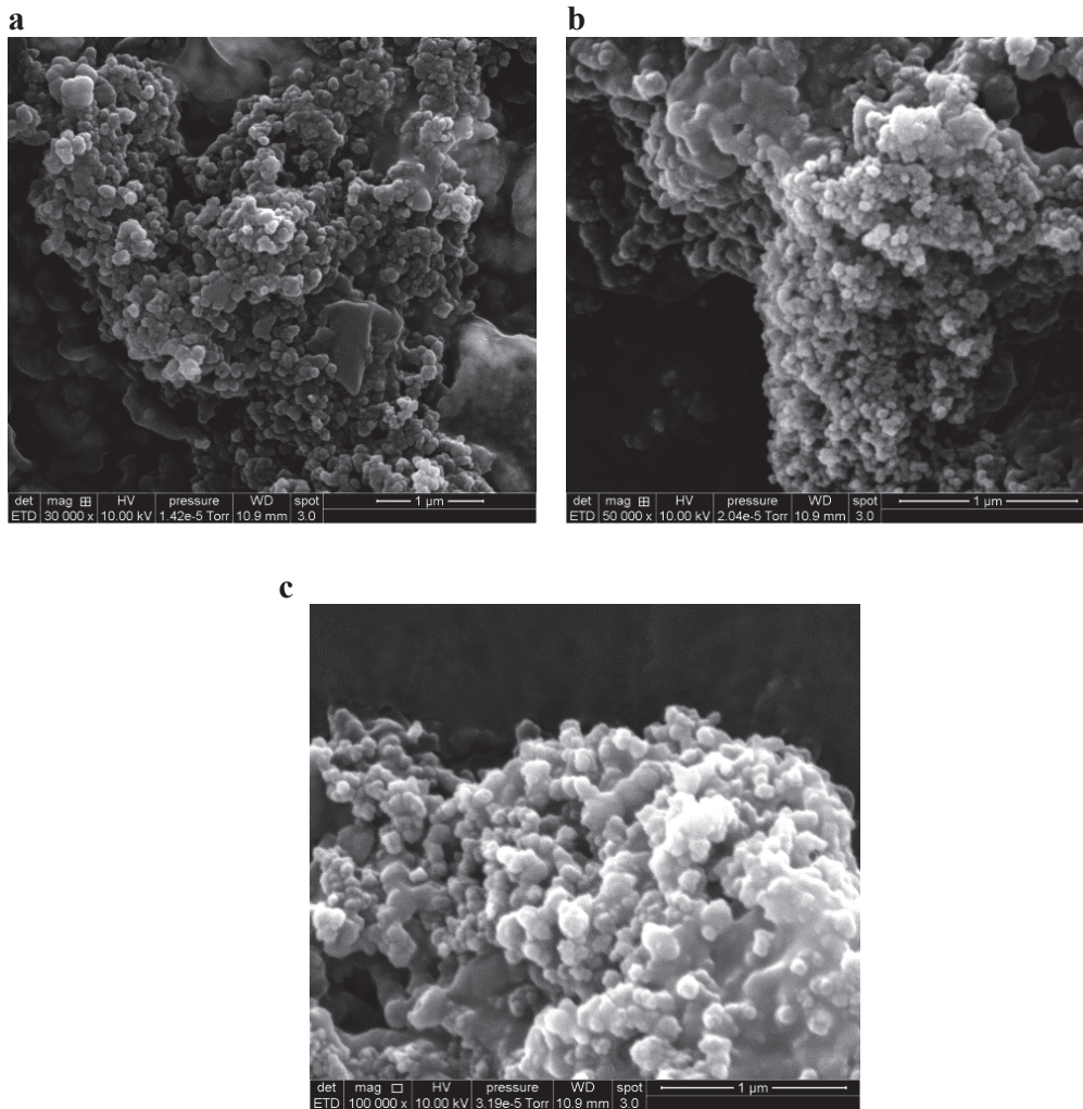
Figure 4.7. Images de nanoparticules à base de PMMA préparées avec de l'acétone ( a ), de l'éthanol ( b ) et du méthanol ( c ) par microscopie électronique à balayage.
