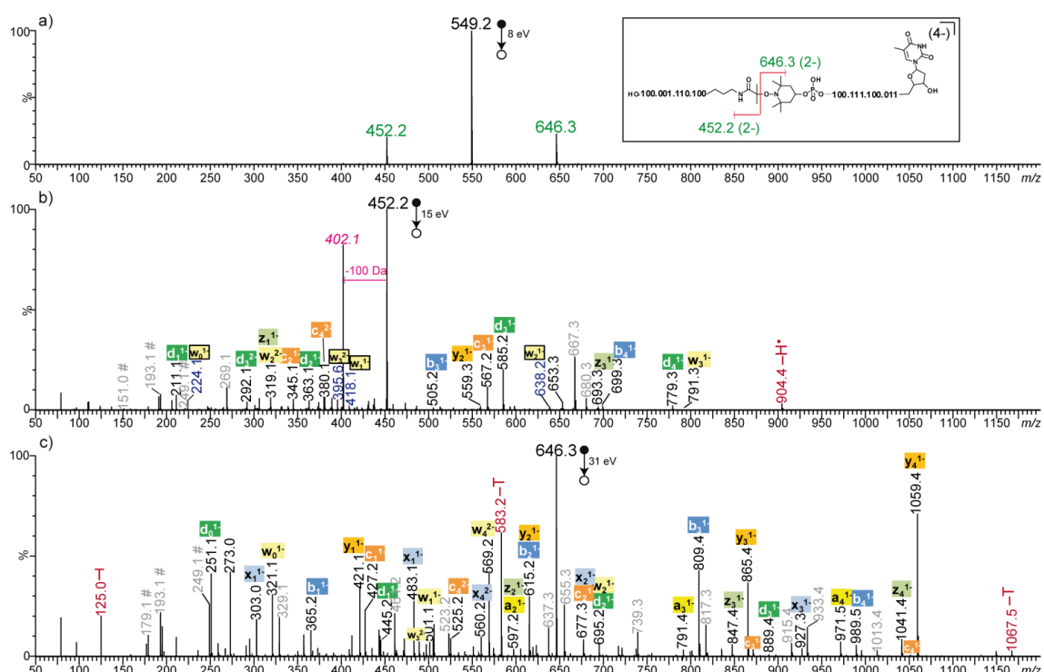
Figure SI-II. 82 : Séquençage de l'oligophosphate détecté comme étant P7. (a) Spectre ESI-MS/MS de l'ion [M-4H]^{4-} à m/z 549,2 et schéma de fragmentation. (b) Spectre pseudo-MS 3 du bloc 1 à m/z 452,2. Les ions encadrés en bleu sont des fragments obtenus après gain d'un H + . (c) Spectre pseudo-MS 3 du bloc 2 à m/z 643,2. Les fragments secondaires (dont les monomères déprotonés, #) sont annotés en gris.
