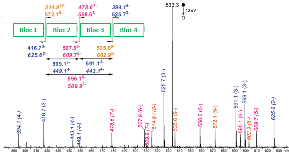
Figure SI-III. 9 : Séquençage de P_{RISCOPE3} . Spectre MS/MS de l'ion [M - 12H]^{12-} à m/z 533,3 et schéma d'homolyse des liaisons alcoxyamines.
