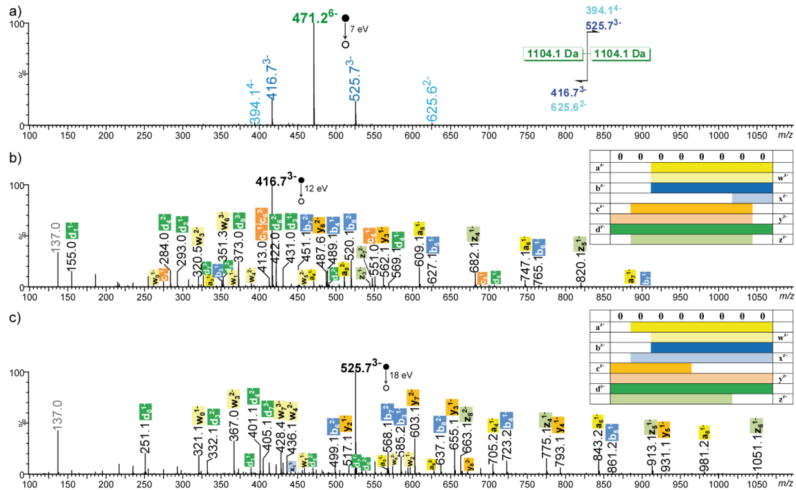
Figure SI-III. 8 : Séquençage de P_{RISCOPE1} . (a) Spectre MS/MS de l'ion [M - 6H]^{6-} à m/z 471,2 et schéma d'homolyse de la liaison alcoxyamine. (b) Spectres pseudo-MS 3 du bloc 1 à m/z 416,7 et couverture de la séquence. (c) Spectres pseudo-MS 3 du bloc 2 à m/z 525,7. Les monomères déprotonés, [O - H]^{-} à m/z 137,0 pour les deux blocs, sont annotés en gris.
