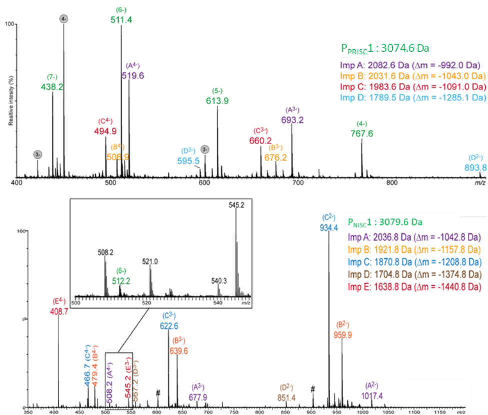
Figure III. 22: (En haut) Spectre ESI-MS en mode négatif de P PRISC 1 en vert. (En bas) Spectre ESI-MS en mode négatif de P NISC 1 en vert. Les impuretés sont annotées en couleurs. Les pics annotés par un rond gris correspondent à des fragments formés en source. # Amas de sel.
