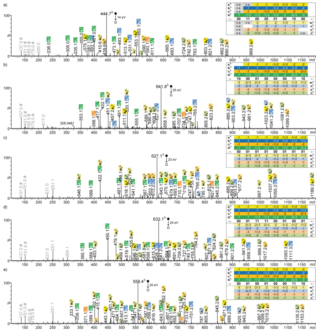
Figure SI-III. 14 : Séquençage en pseudo-MS 3 de PR2. (a) Spectre pseudo-MS 3 du bloc 1 à m/z 447,7 et couverture de la séquence. (b) Spectre pseudo-MS 3 du bloc 2 à m/z 641,8 et couverture de la séquence. (c) Spectre pseudo-MS 3 du bloc 3 à m/z 627,1 et couverture de la séquence. (d) Spectre pseudo-MS 3 du bloc 4 à m/z 633,1 et couverture de la séquence. (e) Spectre pseudo-MS 3 du bloc 5 à m/z 558,4 et couverture de la séquence. Les monomères déprotonés sont annotés en gris.
