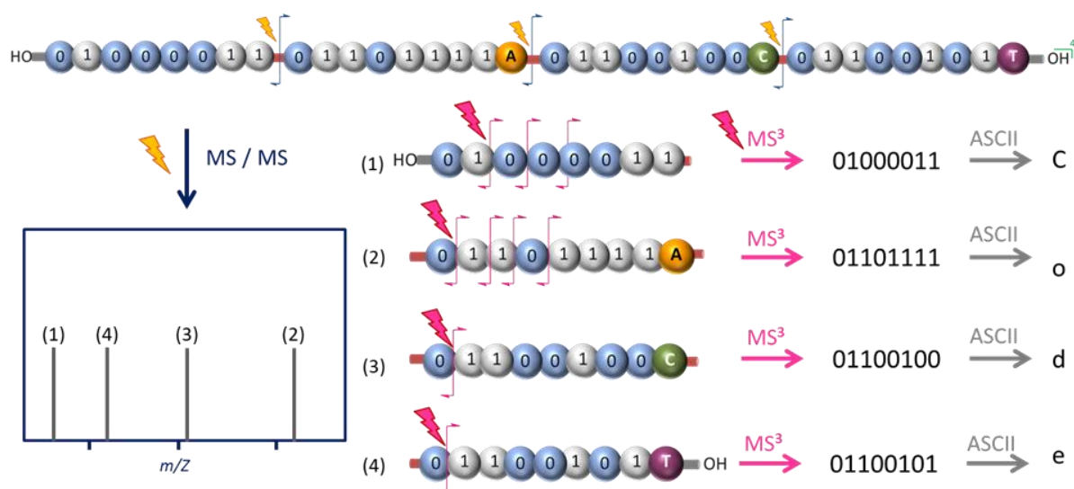
Figure I. 25: Représentation schématisée du séquençage en spectrométrie de masse d'un polymère numérique contenant 4 octets d'information. Séquence codée avec 2 monomères différents. Adaptée de la littérature. 25
