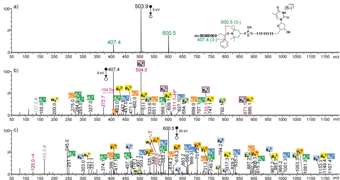
Figure SI-III. 2 : Séquençage de P_{ROSC1} . (a) Spectre ESI-MS/MS de l'ion [M-6H]^{6-} à m/z 503,9 et schéma de fragmentation. (b) Spectre pseudo-MS 3 du bloc 1 à m/z 407,4. L'ion à ms/Z 611,1 provient de l'élimination d'un H^+ à partir de l'ion précurseur. Les ions encadrés en rouge sont des fragments obtenus après abstraction d'un H^+ . (c) Spectre pseudo-MS 3 du bloc 2 à m/z 600,5. Les fragments secondaires (dont les monomères déprotonés, #) sont annotés en gris.
