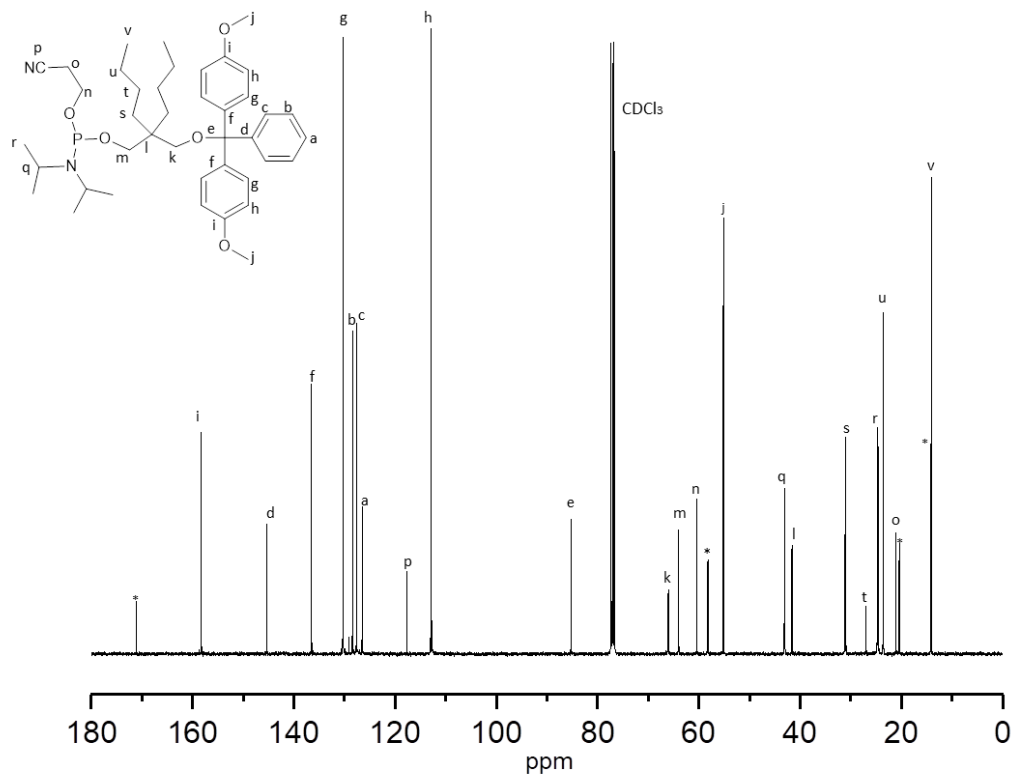
Figure SI-II. 42 : Spectre RMN ^{13}\text{C} ( \text{CDCl}_3 ) du monomère M8.
