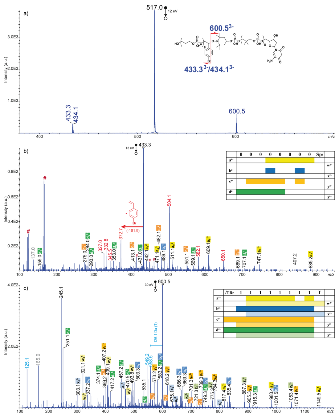
Figure SI-III. 29 : Séquençage de P EM-Br 1. (a) Spectre MS/MS de l'ion [M - 6H]^{6-} à m/z 517,0 et schéma d'homolyse des liaisons C-ON. (b) Spectre pseudo-MS 3 du bloc 1 m/z 433,3. Les pics annotés en rouge sont des fragments secondaires après perte de l'espaceur EM-Br et ceux annotés par # résultent d'interférences en source. Le tableau de couverture de séquence montre qu'aucun fragment contenant le radical styrényle n'est observé. (c) Spectre pseudo-MS 3 du bloc 2 à m/z 600,5. Les ions annotés en cyan sont liés à la perte de la base T. Les tableaux en inset montrent les couvertures de chaque bloc. Dans les spectres (b) et (c) les pics annotés en gris correspondent aux monomères déprotonés.
