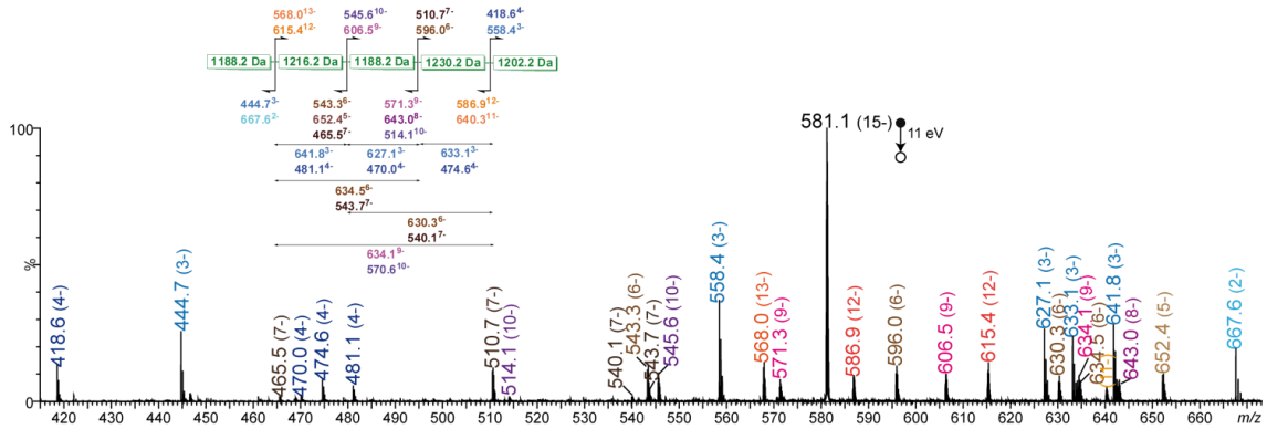
Figure SI-III. 13 : Spectre MS/MS de l'ion [M - 15H]^{15-} à m/z 581,1 de PR2.
