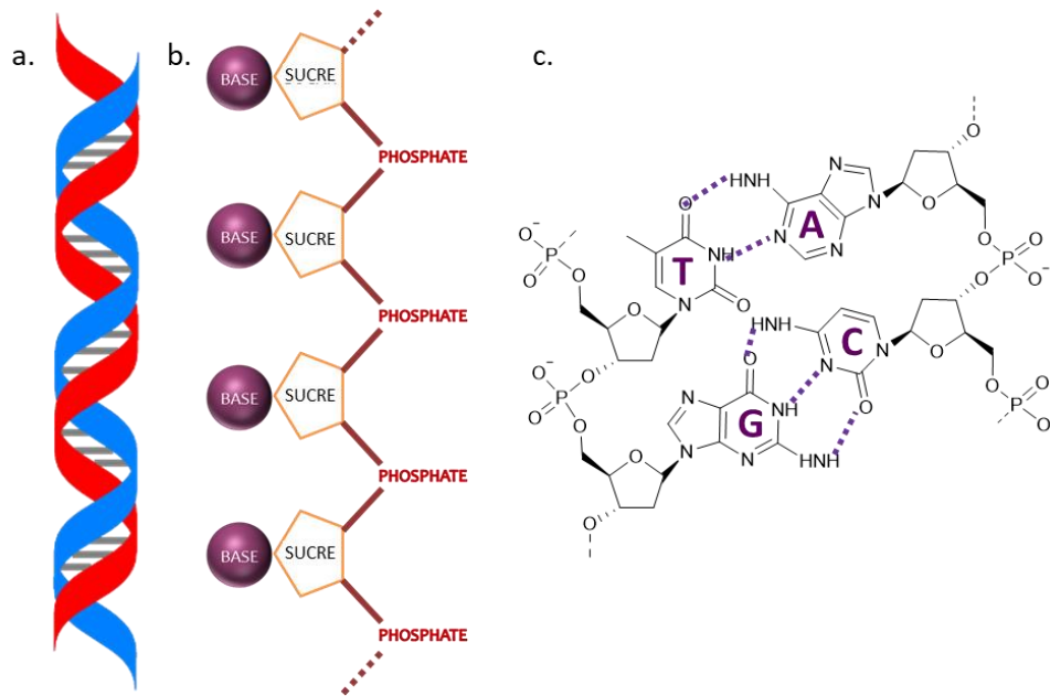
Figure 1. 1 : (a) Représentation schématique de la structure hélicoïdale de l'ADN. Les brins rouge et bleu représentent la chaîne phosphate et les lignes horizontales représentent les liaisons hydrogènes entre les paires de bases. (b) Représentation schématique de la formule chimique d'une simple chaîne. (c) Représentation des deux paires de bases de l'ADN et de leurs liaisons hydrogènes.
