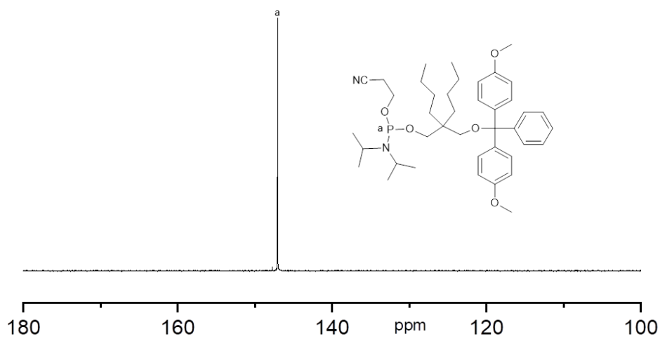
Figure SI-II. 43 : Spectre RMN ^{31}\text{P} ( \text{CDCl}_3 ) du monomère M8.
