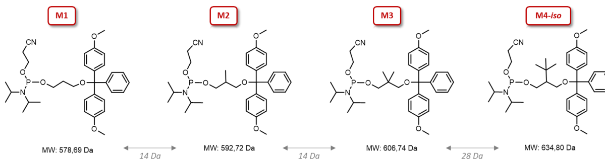
Figure II. 12 : Structure des monomères de la première génération de l'alphabet à 4 symboles.
