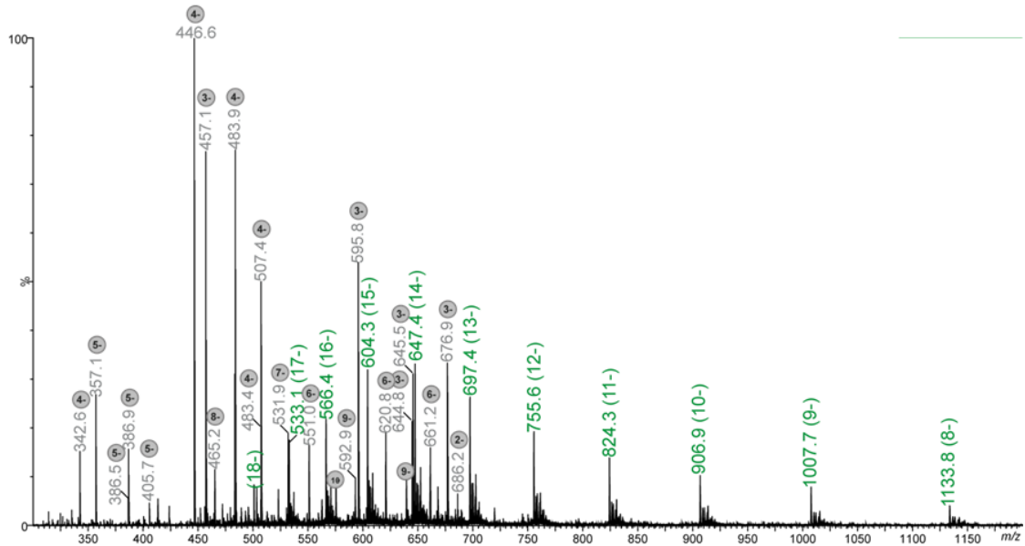
Figure SI-II. 93 : Spectre ESI-MS en mode négatif de P12. Le polymère est détecté exclusivement sous les états de charge 6- à 14- (vert). Les pics annotés en gris correspondent à des fragments formés en source.
