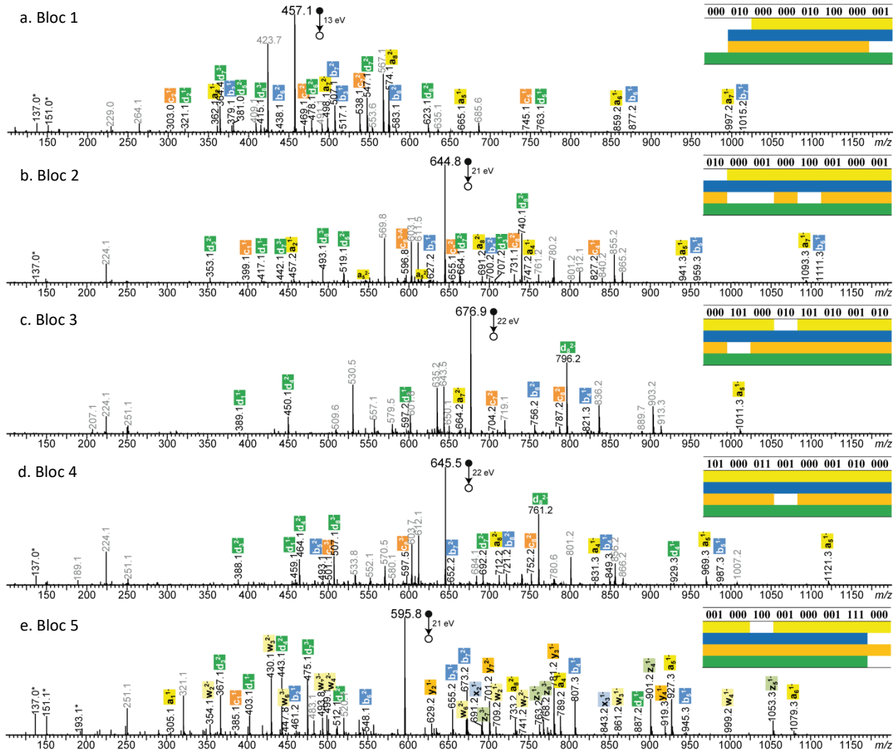
Figure SI-II. 95 : Séquençage du polymère P12. (a) Spectre pseudo-MS 3 du bloc 1 à m/z 457,1 et couverture de la séquence. (b) Spectre pseudo-MS 3 du bloc 2 à m/z 644,8 et couverture de la séquence. (c) Spectre pseudo-MS 3 du bloc 3 à m/z 676,9 et couverture de la séquence. (d) Spectre pseudo-MS 3 du bloc 4 à m/z 645,5 et couverture de la séquence. (e) Spectre pseudo-MS 3 du bloc 5 à m/z 595,8 et couverture de la séquence. Les monomères déprotonés sont annotés avec *. Les ions annotés en gris sont des fragments issus de réactions induites par le radical carboné.
