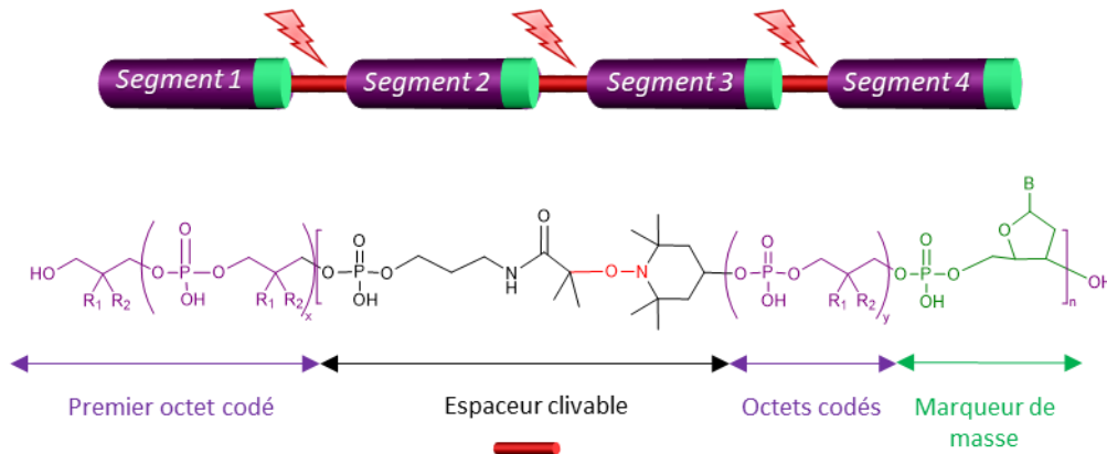
Figure 2: En haut, schéma du design d'une séquence contenant un espaceur (en rouge) et des marqueurs (en vert). En bas, exemple de structure d'une chaîne de poly(phosphodiester)s contenant un espaceur et un marqueur de masse.
