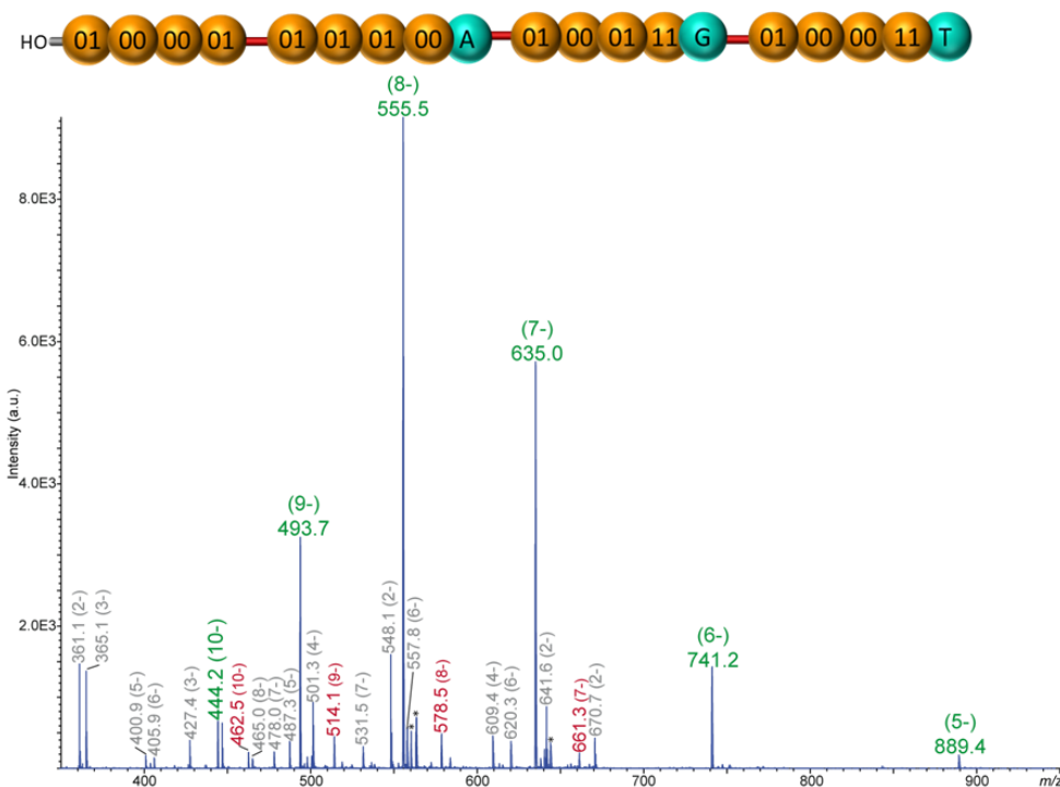
Figure SI-II. 73 : Spectre ESI-MS en mode négatif de P3. L'oligophosphate est observé sous les états de charge -5 à -10 (en vert) ainsi que des fragments formés en source après différents clivages de liaisons alcoxyamine (en gris). Une impureté mineure est également observée avec un excès de masse de 183,8 Da (en rouge).
