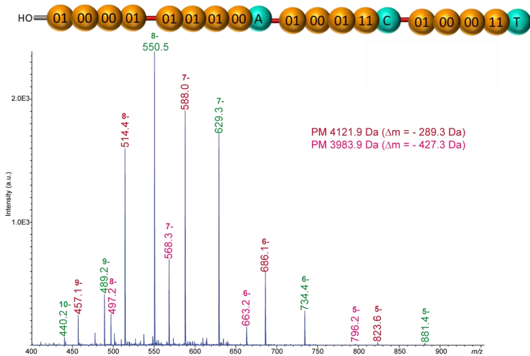
Figure SI-II. 67 : Spectre ESI-MS en mode négatif de P2. Le polymère recherché est détecté sous les états de charges -5 à -10 (en vert). Les pics annotés en rouge correspondent aux états de charge d'une molécule de masse 4121,9 Da ( \Delta m = -289,3 Da), ceux en rose correspondent aux états de charge d'une molécule de masse 3983,9 Da ( \Delta m = -427,3 Da).
