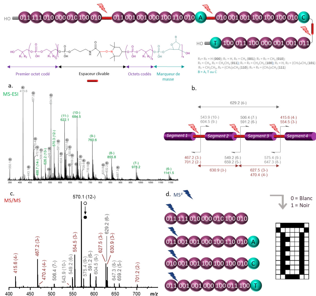
Figure II. 24 : Analyse de spectrométrie de masse du polymère P11 . (En haut) Schéma de la structure globale du polymère P11 . (a) Spectre MS montrant les différents états de charges du polymère. Les annotations grises sont des fragments formés en source. (b) Schéma de fragmentation en MS/MS. (c) Spectre de masse en tandem issu de l'ion précurseur [M-12H]^{12-} à m/z 570.1. (d) Blocs issus du spectre MS/MS, puis analyse MS^3 pour retrouver l'image encodée.
