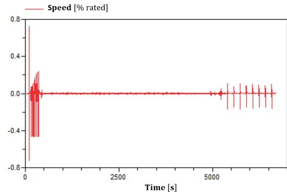
(d) Speed
