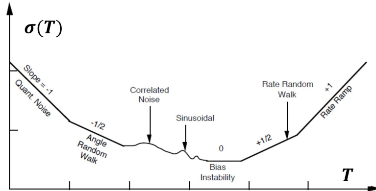
FIGURE H.1: Tracé de l'écart d'Allan (adapté de [IEE06])
