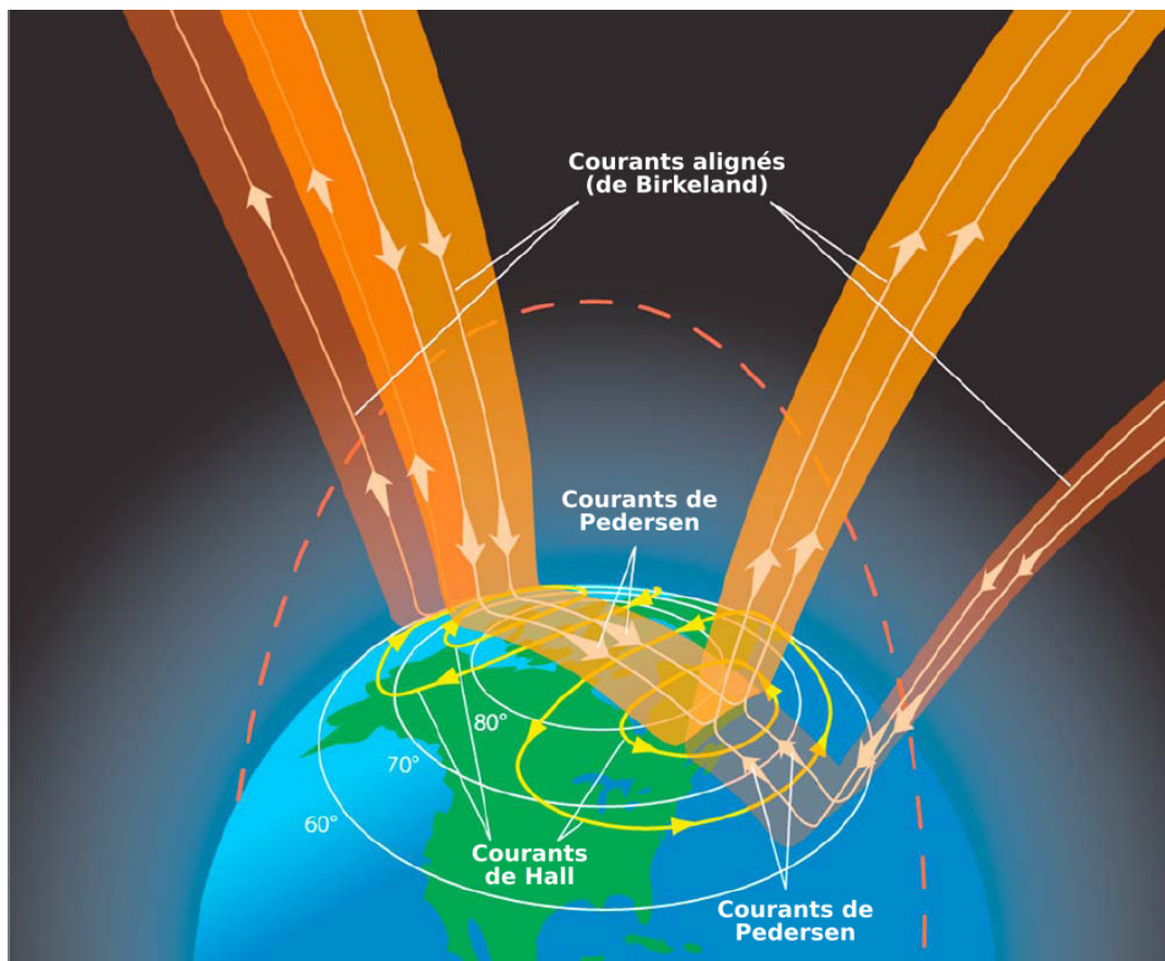
FIGURE 1.4 – Représentation schématisée des courants traversant l'ionosphère aux hautes latitudes. (crédit : adaptée de Wikipédia : Courants de Birkeland)
