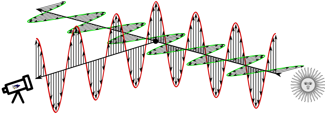
FIGURE 5.3 – Représentation schématique de la diffusion Rayleigh. Deux ondes lumineuses incidentes arrivent du coin inférieur droit avec deux directions de polarisations perpendiculaires (représentées en vert et rouge pour mieux les distinguer). Un diffuseur plus petit que la longueur d'onde est placé sur son chemin. Le plan de diffusion est le plan contenant le rayon incident et le rayon diffusé. Un observateur placé à gauche ne recevra que de la lumière polarisée verticalement (ici en rouge). Généralement, ce sera vrai pour n'importe quel observateur positionné dans un plan horizontal. On remarque que si l'observateur se place en face de la source, alors il verra les deux polarisations à la fois, soit un DoLP de 0%.
